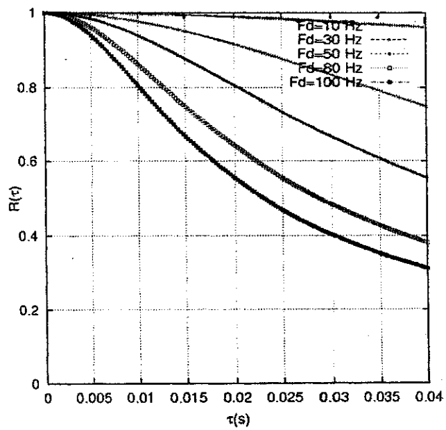
Figura 4.10: Autocorrelação do canal para diferentes valores de frequência Doppler, dispersão angular igual a 20^\circ e ângulo \phi_0 igual a 0^\circ .
