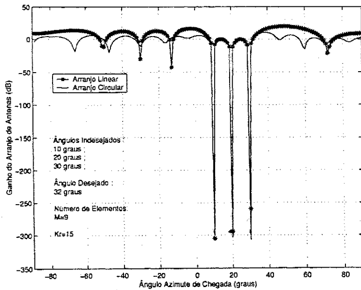
Figura 3.11: Ganho ( G_a ) do arranjo com 10 elementos e kr = 10 .
