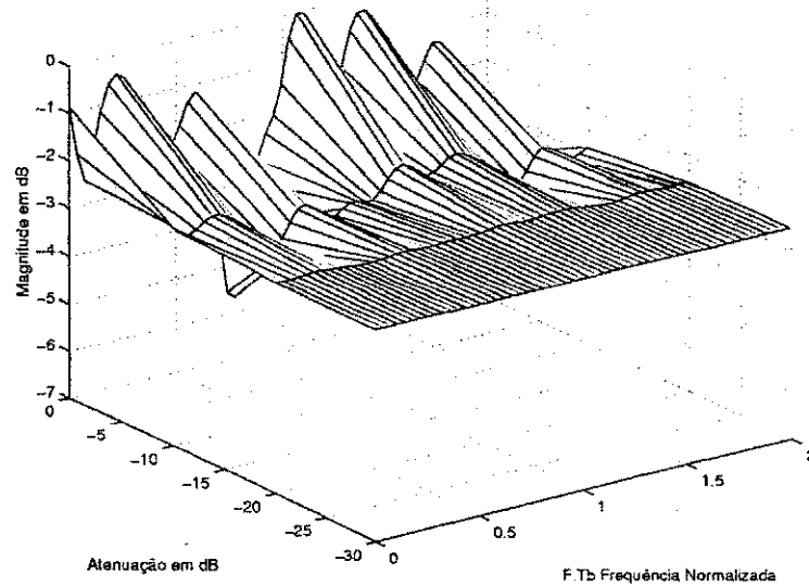
Figura 5.2: Redução da seletividade em frequência do canal com o uso de antenas inteligentes.
