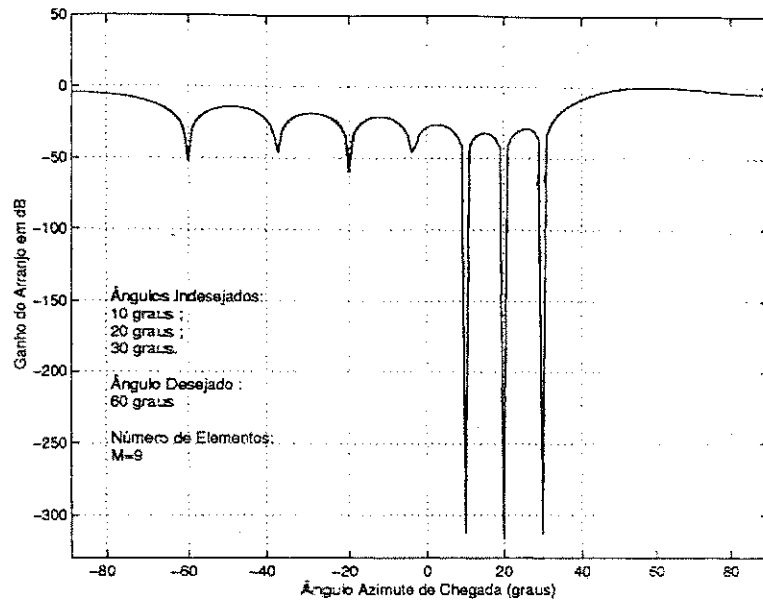
Figura 3.4: Resultado de simulação do método de autoanálise considerando um arranjo com 9 elementos.
