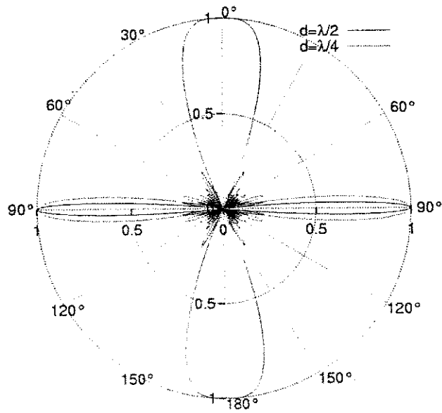
Figura 2.9: Fator de arranjo usando os coeficientes de Dolph-Tschebyscheff, 10 elementos e espaçamentos, \lambda/2 e \lambda/4 .
