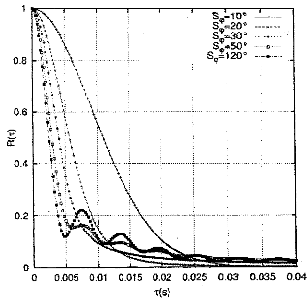
Figura 4.8: Autocorrelação do canal para diferentes valores de dispersão angular, frequência Doppler máxima igual a 100Hz e ângulo \phi_0 igual a 45^\circ .
