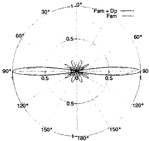
(a) Fator de arranjo médio mais o desvio padrão.
