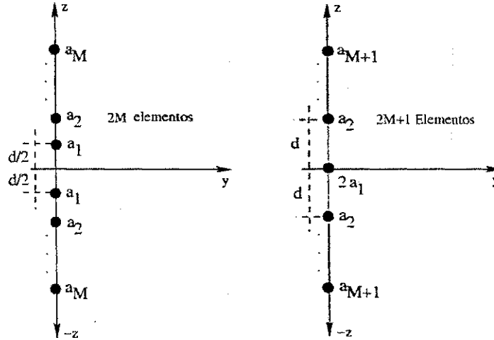
Figura-2.6: Arranjo linear com 2M e 2M + 1 elementos.
