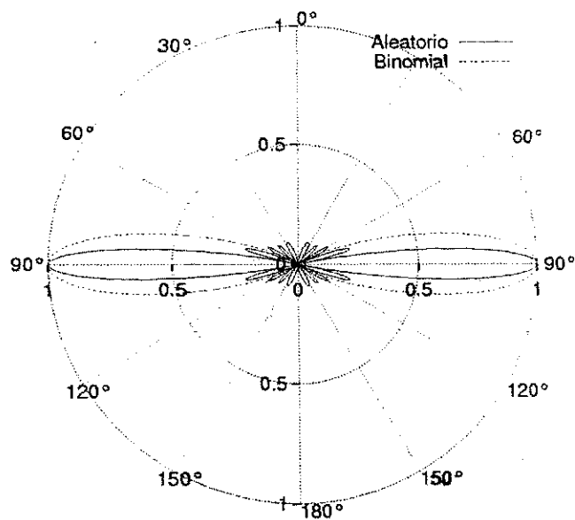
Figura 2.12: Comparação entre o uso de coeficientes aleatórios ( a_n \sim U[5, 10] ) e o uso dos coeficientes binomiais, considerando um arranjo com 10 elementos e d = \lambda/2 .
