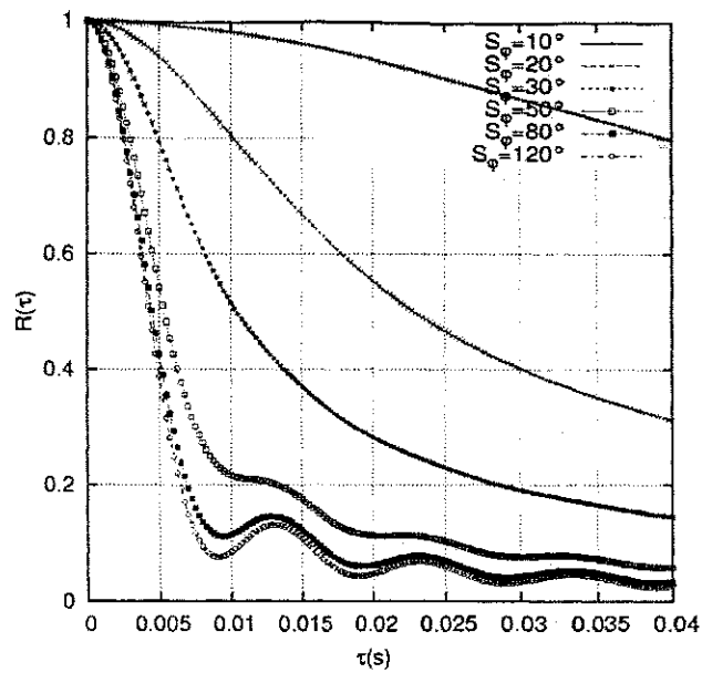
Figura 4.7: Autocorrelação do canal para diferentes valores de dispersão angular, frequência Doppler máxima igual a 100Hz e ângulo \phi_0 igual a 0^\circ .
