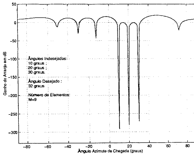
Figura 3.5: Resultado de simulação considerando um ângulo desejado muito próximo dos ângulos interferentes. Verifica-se uma redução da atenuação aplicada aos sinais indesejados.
