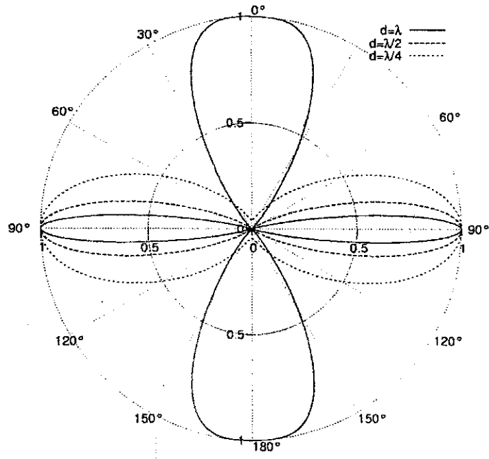
Figura 2.8: Fator de arranjo usando coeficientes binomiais e 10 elementos.
