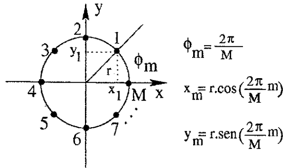
Figura 3.7: Arranjo Circular com M elementos e raio r .
