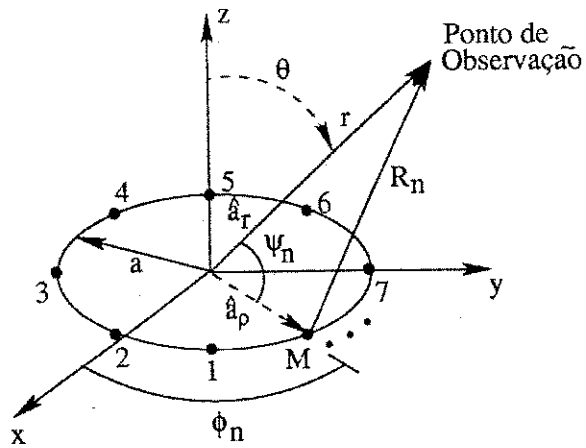
Figura 2.10: Arranjo circular.
