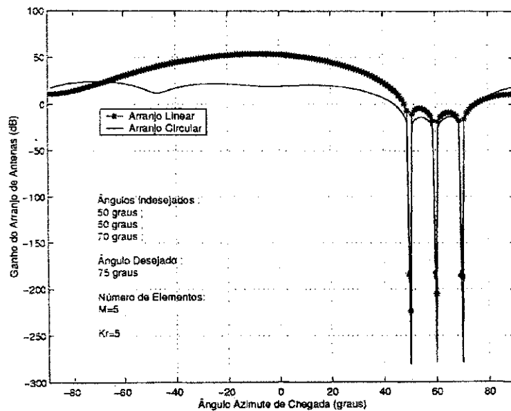
Figura 3.8: Avaliação do desempenho do método de autoanálise considerando duas configurações de arranjo, linear e circular.
