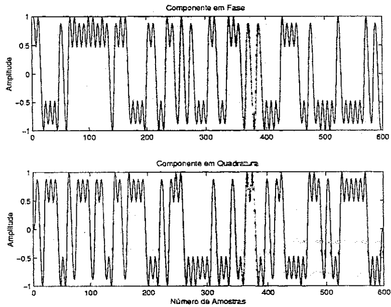
Figura A.2: Sinal GMSK no domínio do tempo.
