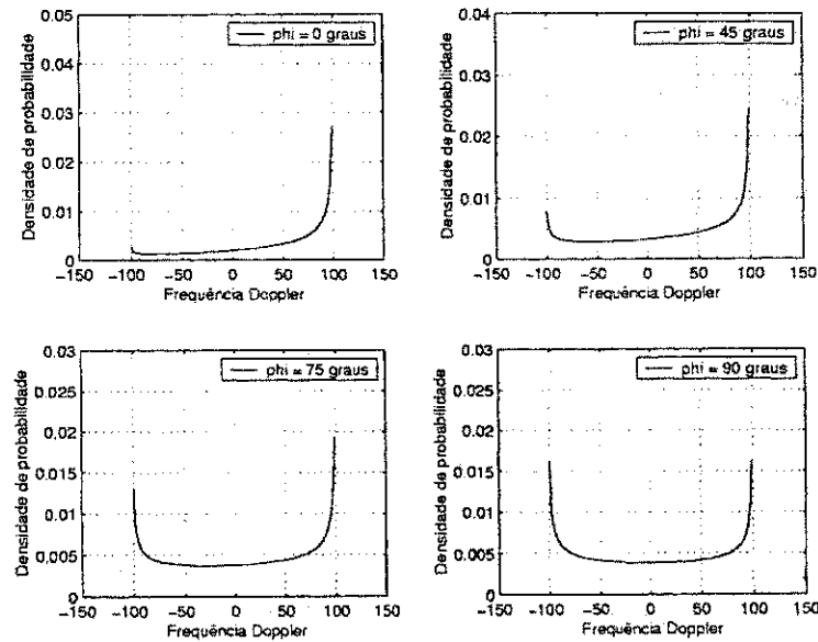
Figura 4.6: Comportamento da densidade de probabilidade da variável aleatória f_D , considerando o ângulo \phi_o igual a 0^\circ , 45^\circ , 75^\circ e 90^\circ , dispersão angular igual a 80^\circ e frequência Doppler máxima igual a 100Hz.
