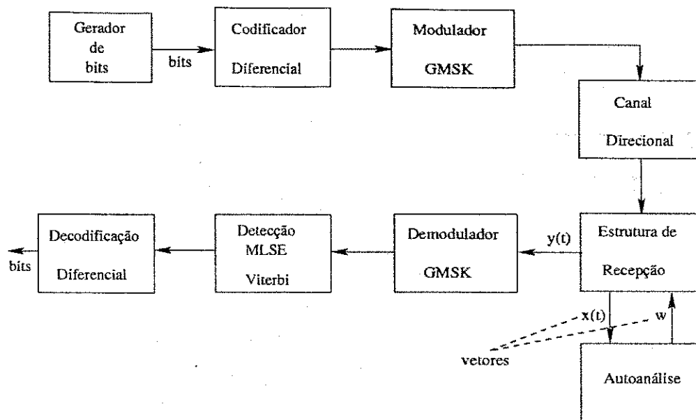
Figura 5.1: Diagrama de simulação em bloco.
