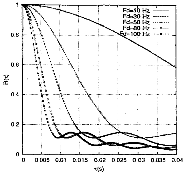
Figura 4.9: Autocorrelação do canal para diferentes valores de frequência Doppler, dispersão angular igual a 80^\circ e ângulo \phi_0 igual a 0^\circ .
