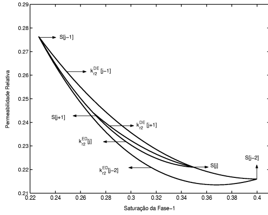
Figura 1.13: Curvas de Reversão-Caso Geral ( j par)
