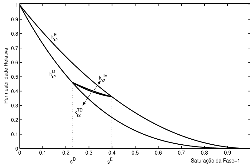
Figura 1.7: Curvas de Permeabilidade Relativa de Reversão.
