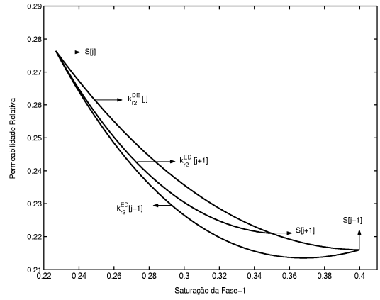
Figura 1.14: Curvas de Reversão-Caso Geral ( j ímpar)
