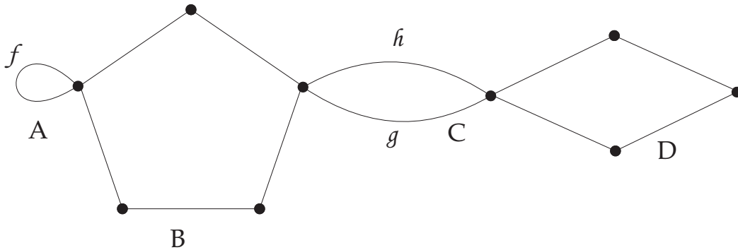
Figura 1.1: Grafo G
