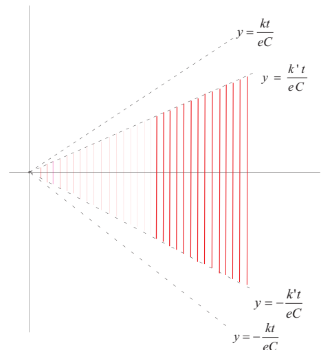
Figura 1.21: O setor \Delta_{\frac{k't}{Ce}} .
