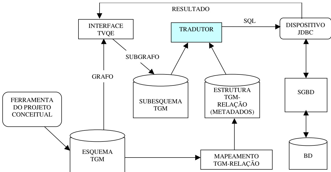
Figura 4.1 – Arquitetura funcional do TVQE
