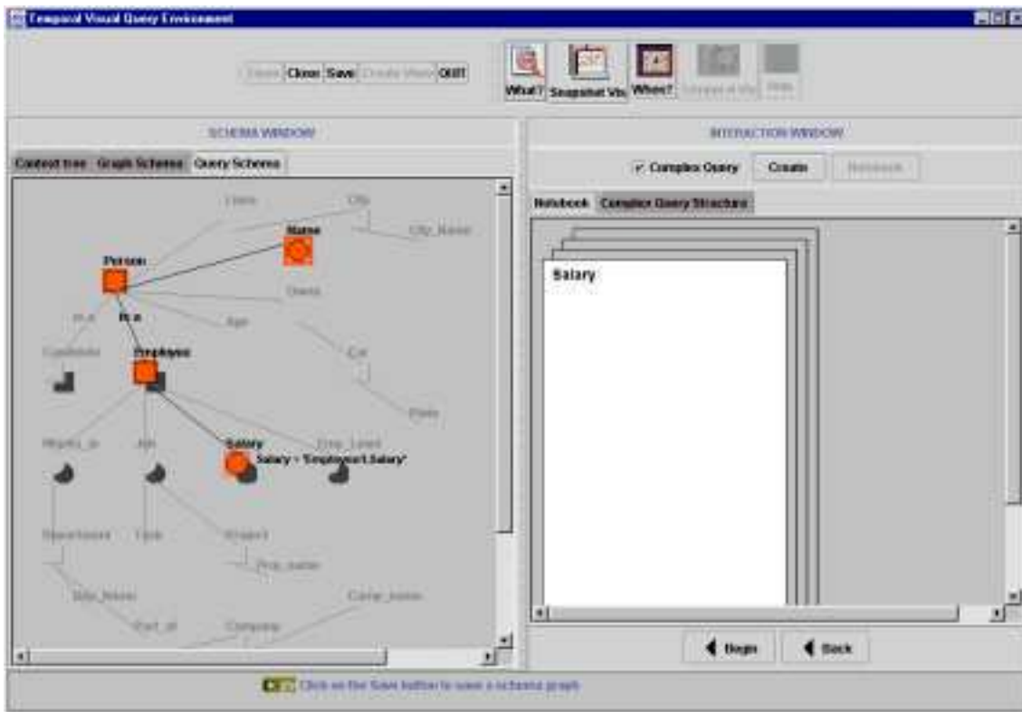
Figura 3.10 (c) – Esquema final da consulta complexa
