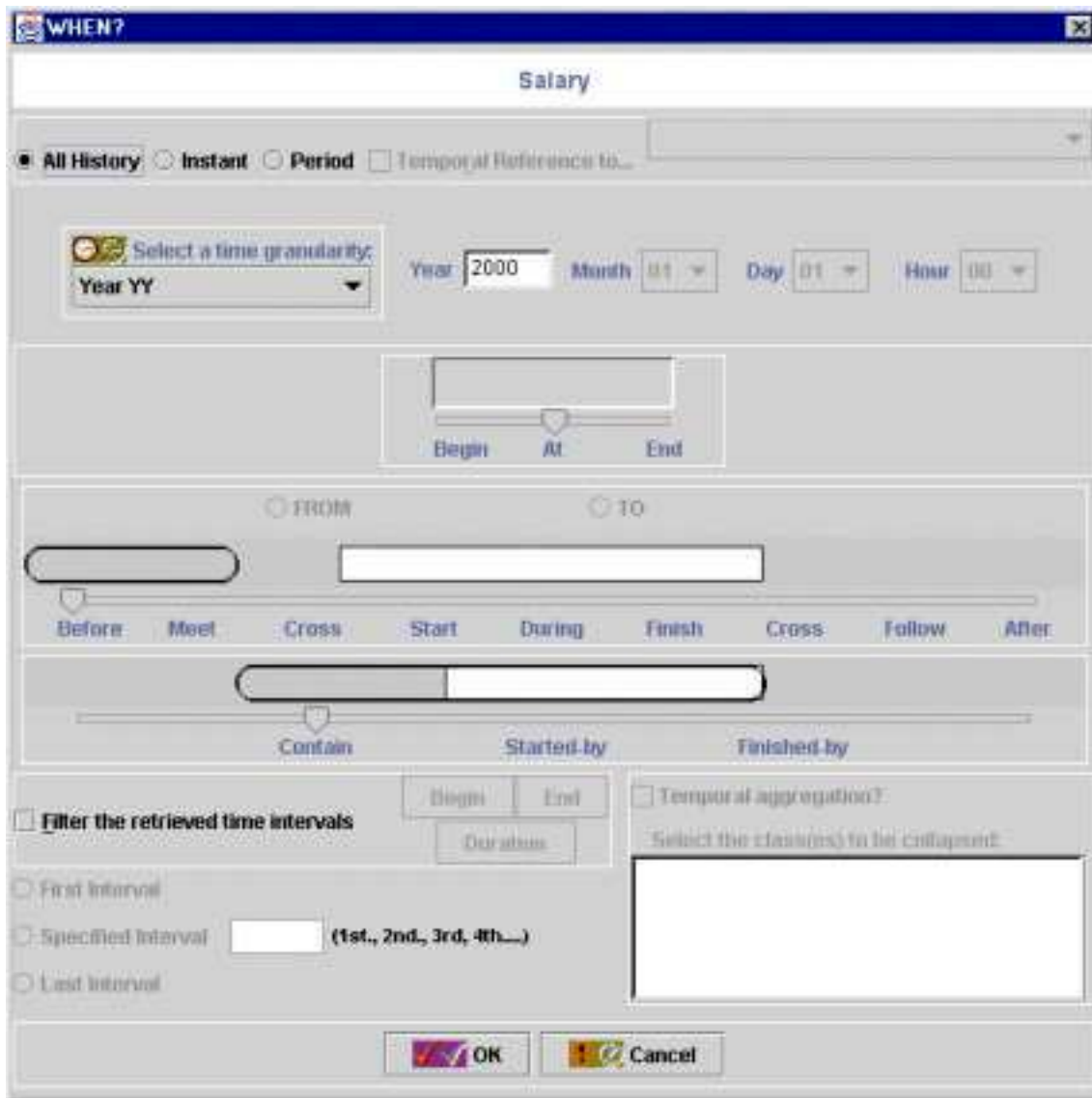
Figura 4.6 – Especificação da condição temporal All History para o atributo Salary
