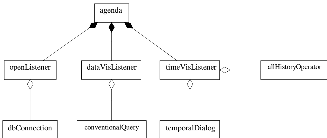
Figura 5.3 – Diagrama de Classes 1
