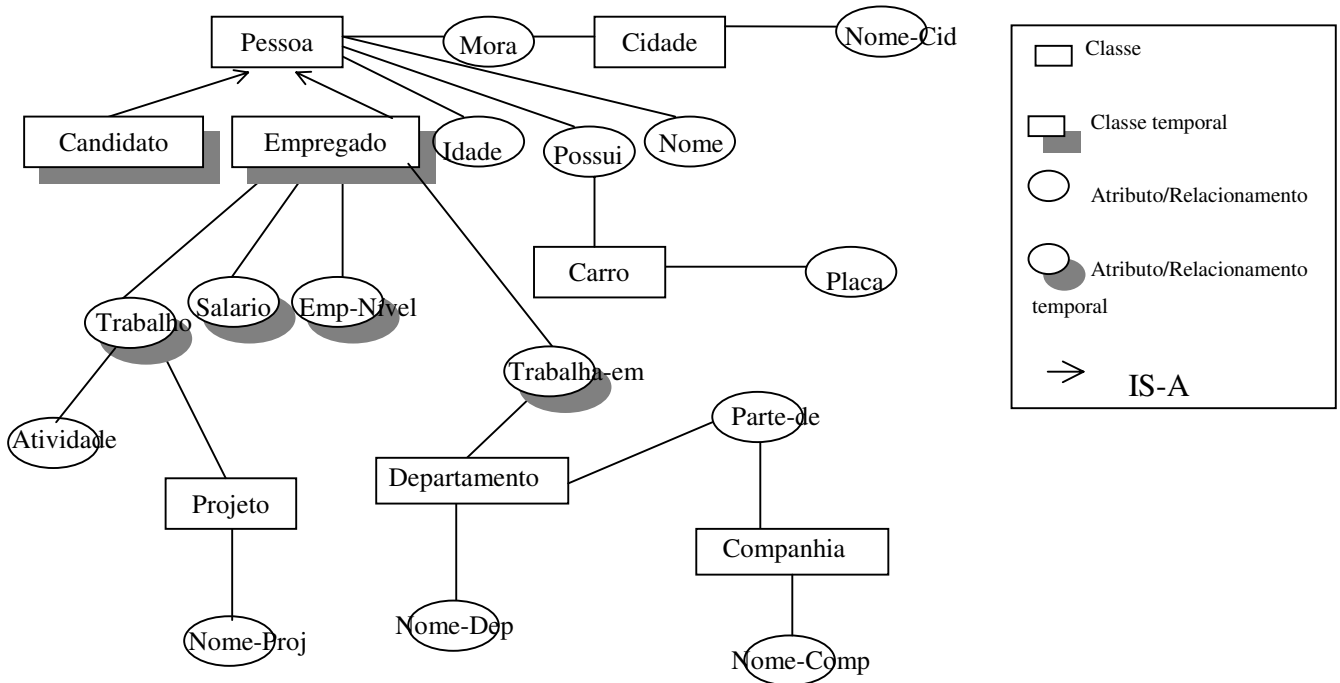
Figura 4.2 – Esquema gráfico TGM de uma agência de empregos
