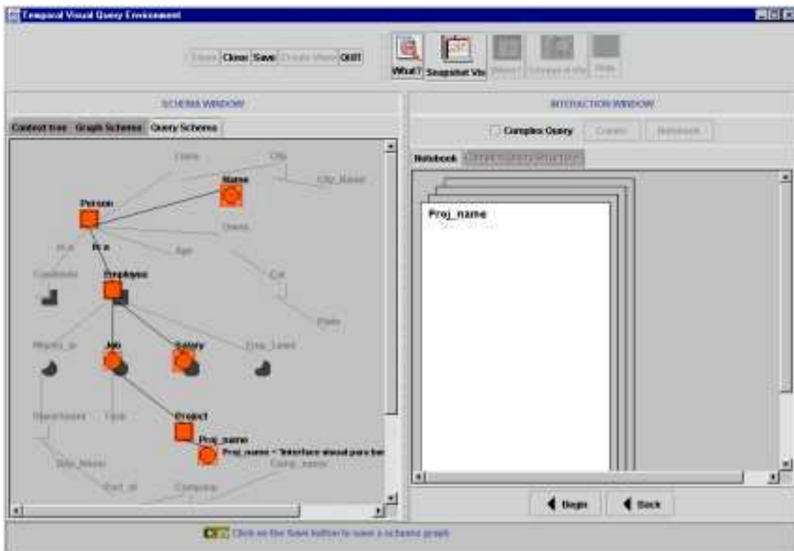
Figura 4.4 – Resultado intensional da consulta
