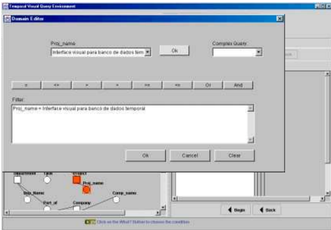
Figura 4.3 – Especificação da condição da consulta no TVQE
