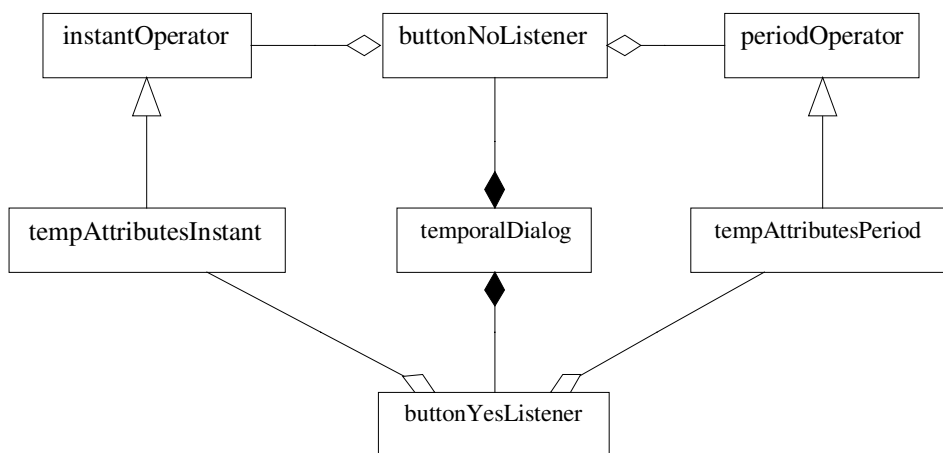
Figura 5.5 – Diagrama de Classes 3
