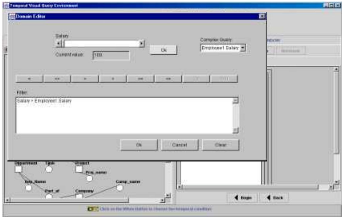
Figura 3.10 (b) – Especificação da condição da consulta complexa
