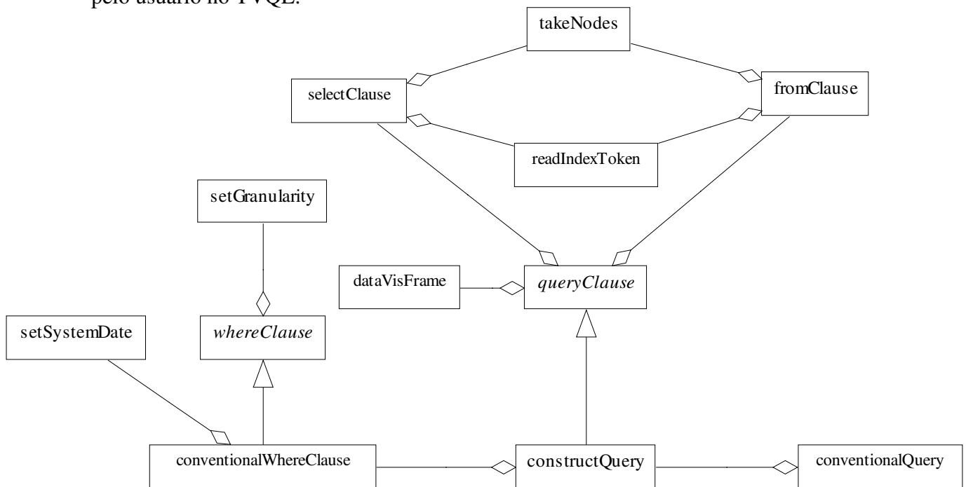
Figura 5.4 – Diagrama de Classes 2
