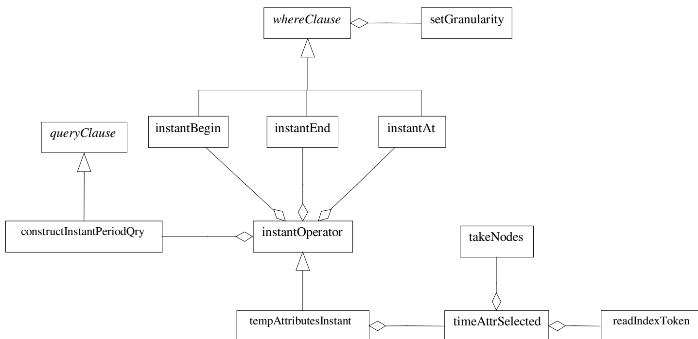
Figura 5.7 – Diagrama de classes 5
