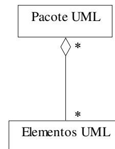
Figura 5.2 (c) – Notação de Agregação
