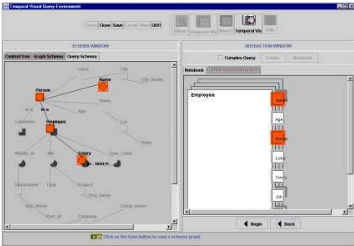
Figura 4.10(a) – Resultado intensional da consulta para o operador At
