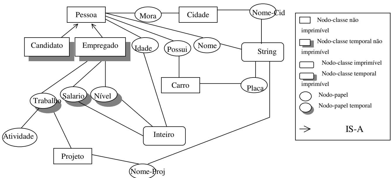
Figura 3.1 – Um typed graph g com extensão temporal
