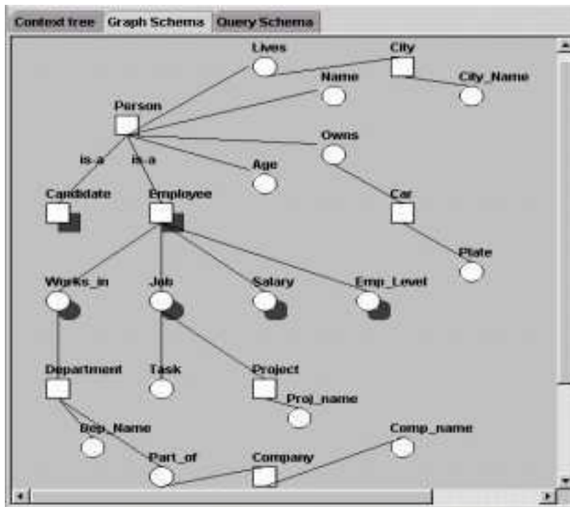
Figura 3.4 – Esquema gráfico de uma agência de empregos no TVQE
