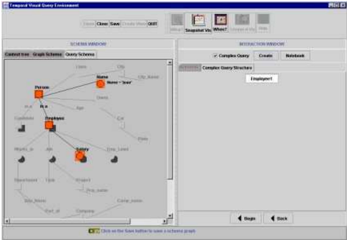
Figura 3.10 (a) – Especificação da consulta que faz parte da condição da consulta complexa
