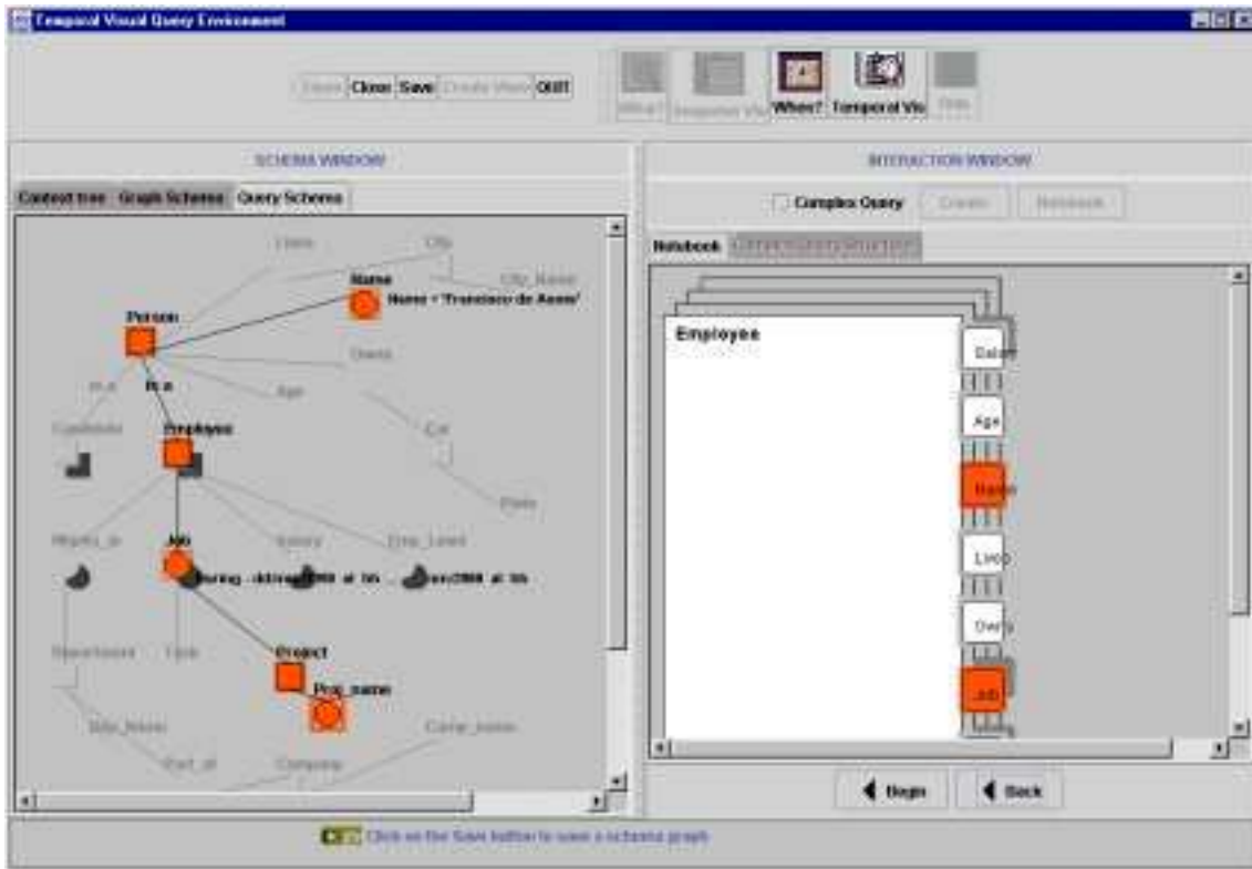
Figura 4.12(a) – Resultado intensional da consulta usando o operador During
