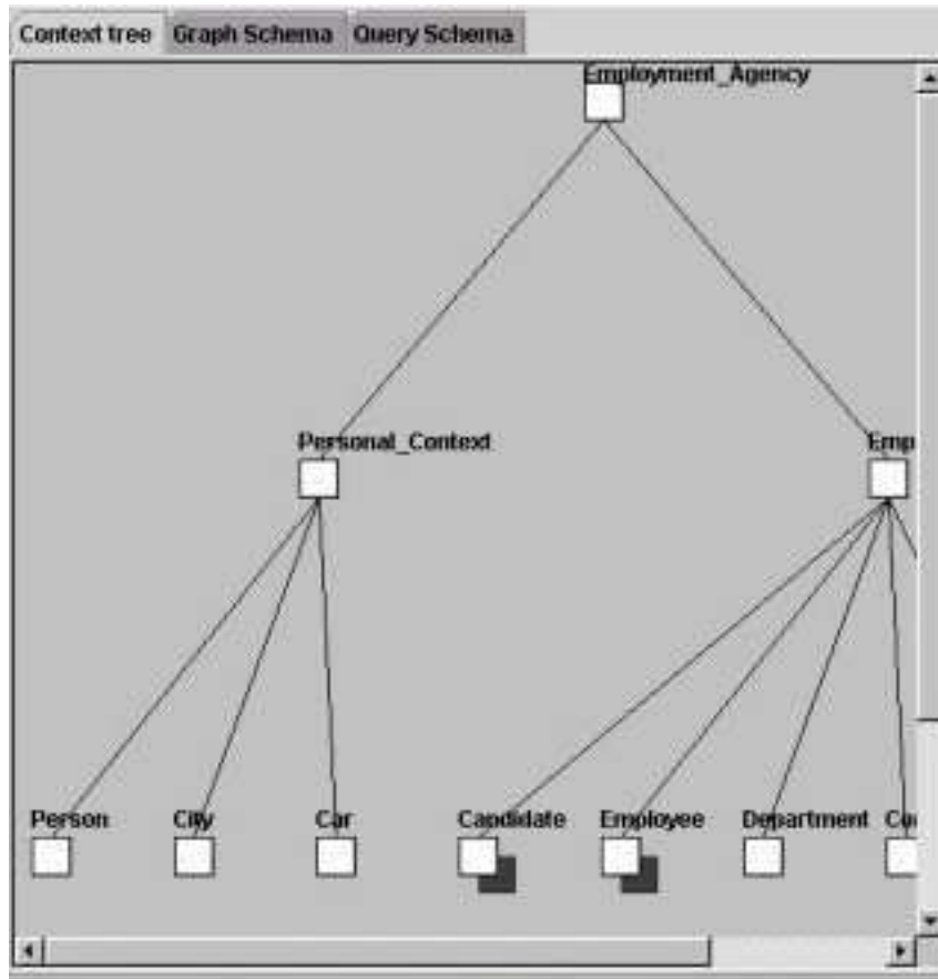
Figura 3.3 – Uma árvore de contextos de uma agência de empregos no TVQE
