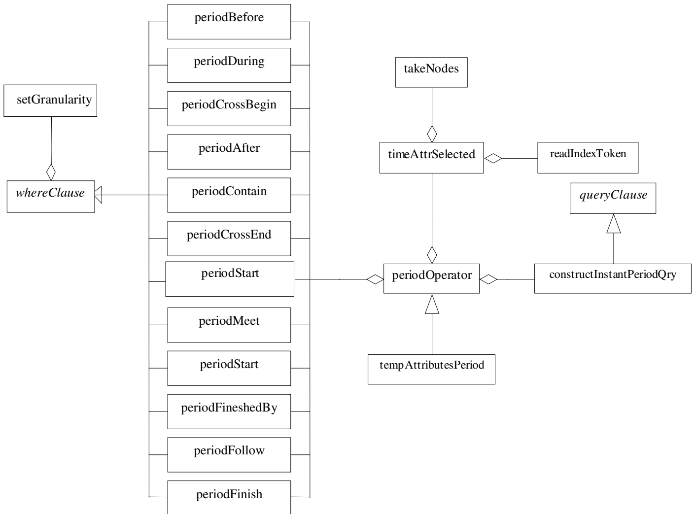
Figura 5.8 – Diagrama de Classes 6
