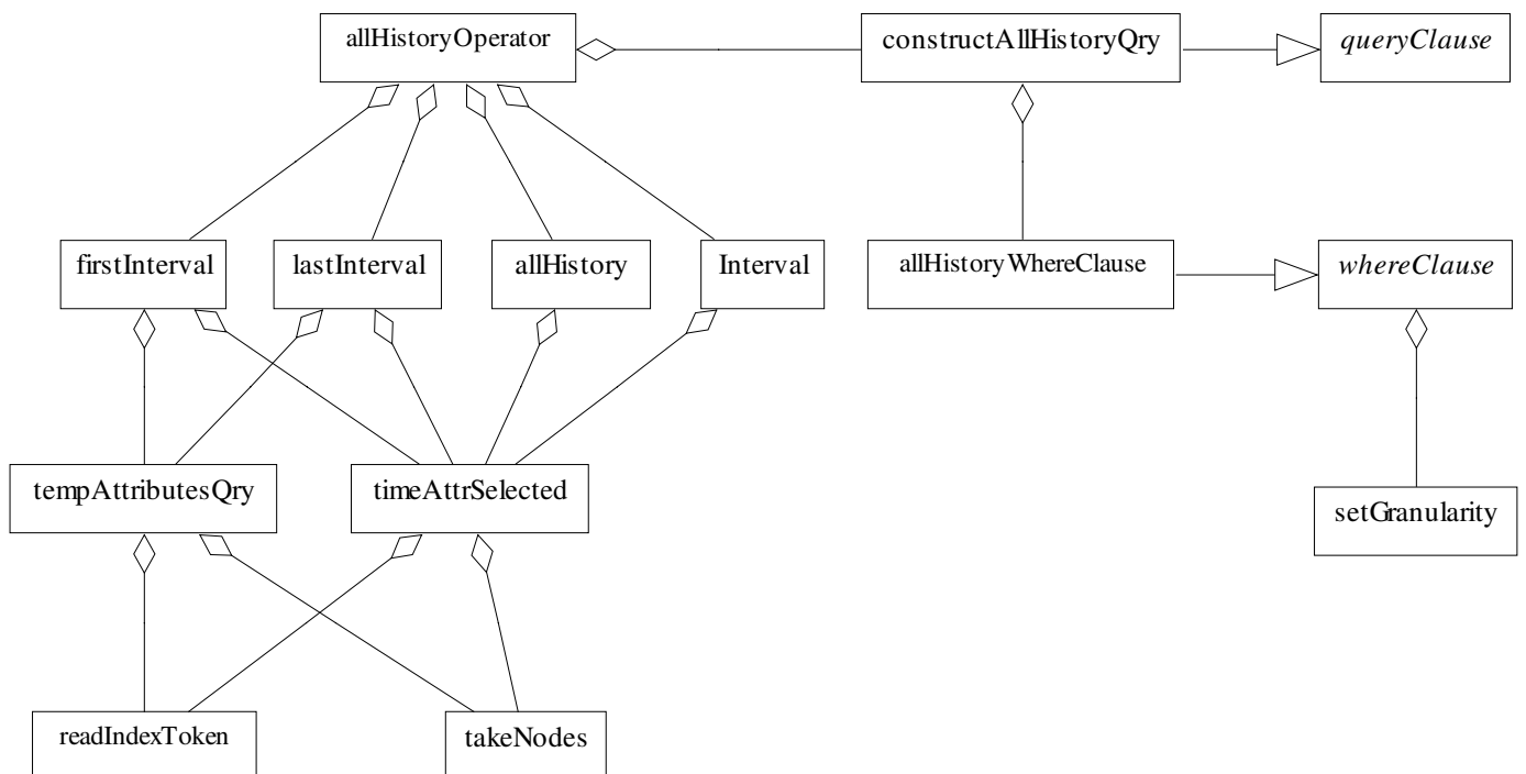
Figura 5.6 – Diagrama de Classes 4
