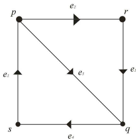
Figura 2.1: Desenho do grafo do Exemplo 2.1
