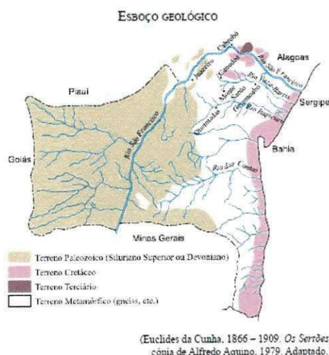
Figura 3: Esboço geológico do Estado da Bahia
