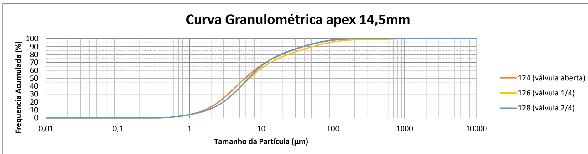
Figura 23: Distribuição porcentual do tamanho de partículas da fração do “overflow” do ciclone com variação do fluxo de alimentação. Condições operacionais: abertura do apex de 15 mm e 14,5 mm e pressão de alimentação de 0,50 kgf·cm -2 .
