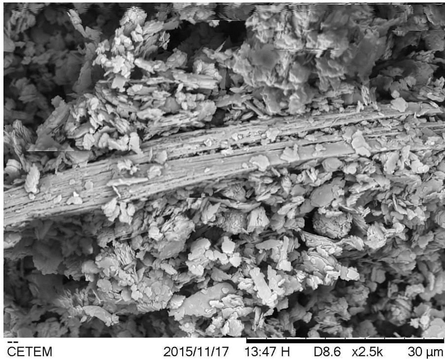
Figura 33: MEV - Micrografia da fração overflow do ciclone , mostrando partículas de caulinita e presença de mica moscovita, Aumento: 2.500x.
