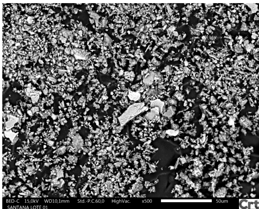
Figura 37: MEV da amostra nº 01. Aumento: 500x
