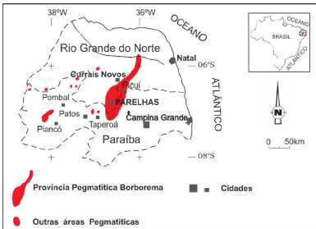
Figura 2: Localização da Província Pegmatítica da Borborema Fonte: Miranda et al. , 2012.
