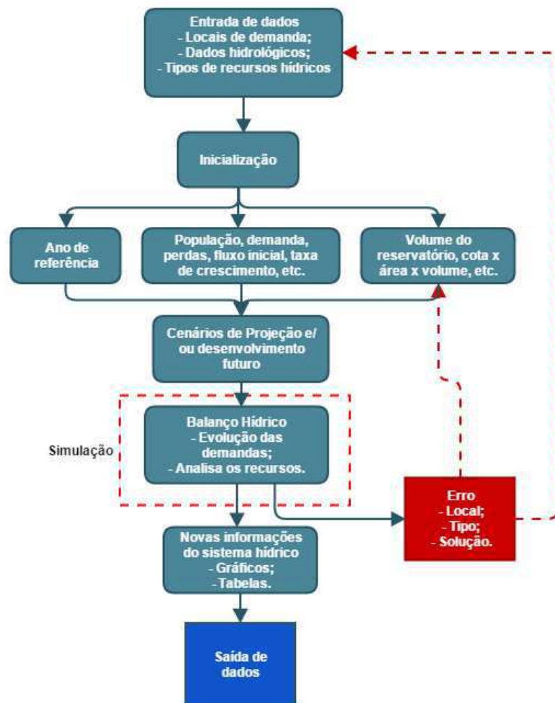
FIGURA 4 – Fluxograma representativo da operação no modelo WEAP.
