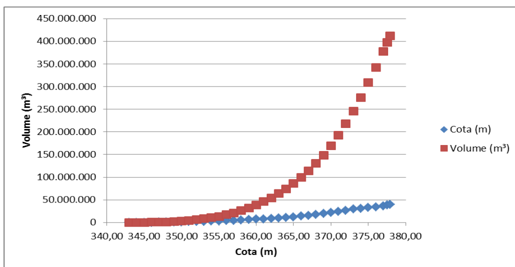
GRÁFICO 1 – Curva Cota x Área x Volume do reservatório Epitácio Pessoa – PB
