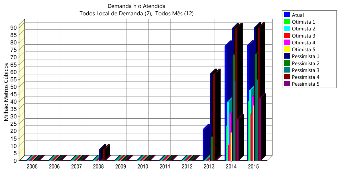
GRÁFICO 7 – Demandas não atendidas para Abastecimento de Campina Grande e Áreas Irrigadas de Boqueirão no modelo WEAP.
