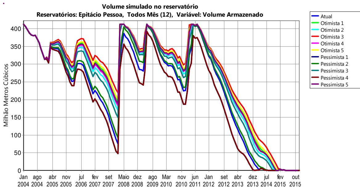
GRÁFICO 9 – Volumes do reservatório para operação entre 2004 – 2015 para todos os cenários no WEAP.
