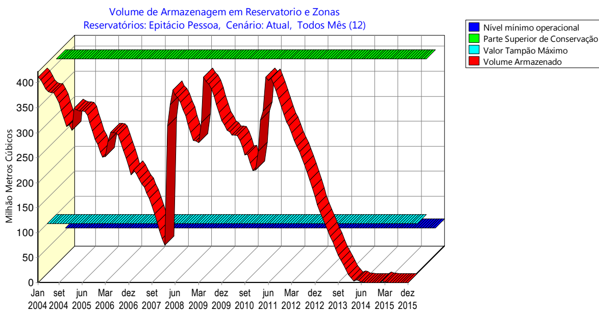
GRÁFICO 3 – Representação das zonas de operação do reservatório no Modelo WEAP – Cenário de Operação Atual.
