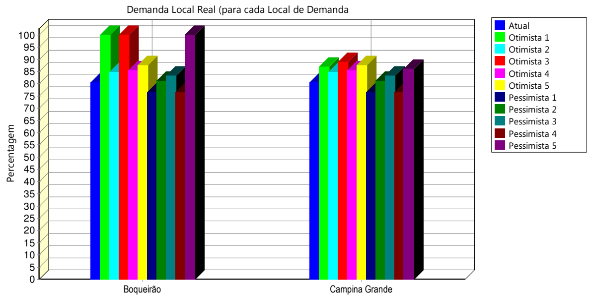
GRÁFICO 8 – Confiabilidade no atendimento às demandas para todos os cenários no WEAP.
