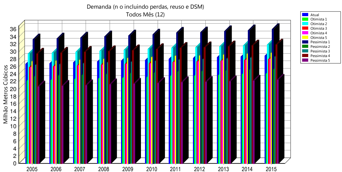
GRÁFICO 5 – Demandas para Campina Grande no modelo WEAP.
