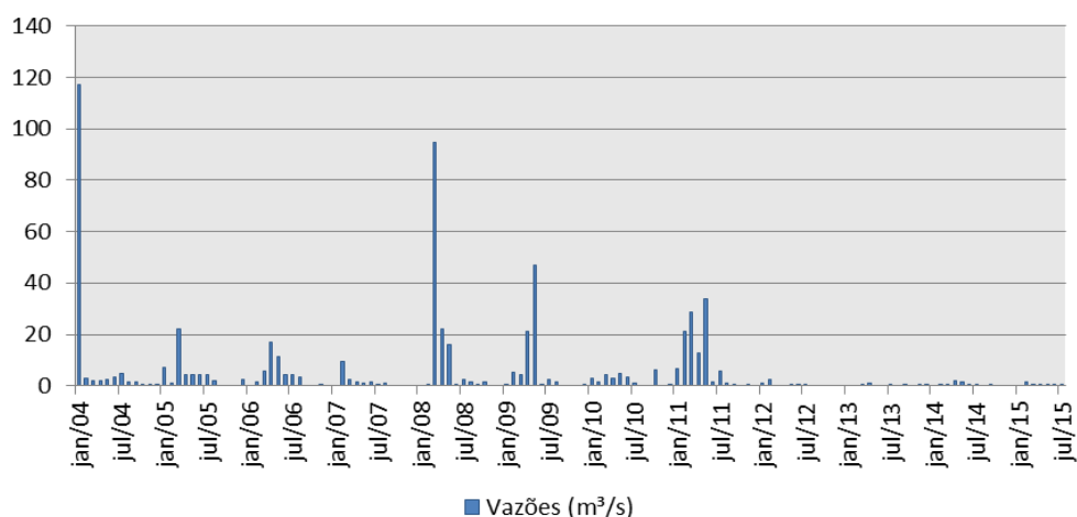
GRÁFICO 2 – Dados de vazão afluente no rio Paraíba à montante do reservatório Epitácio Pessoa – PB
