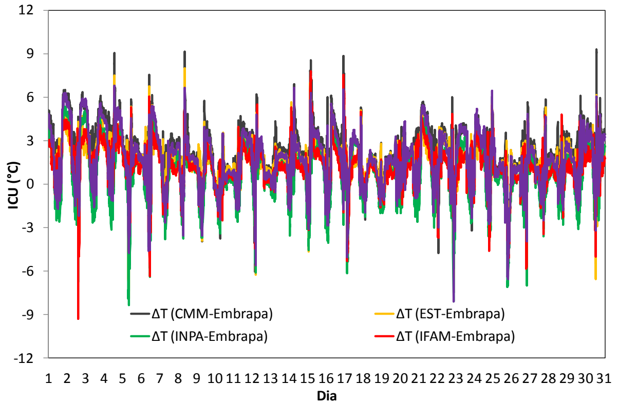
Figura 5. Variabilidade diária da ICU a cada 5 minutos para o mês de janeiro de 2014.
