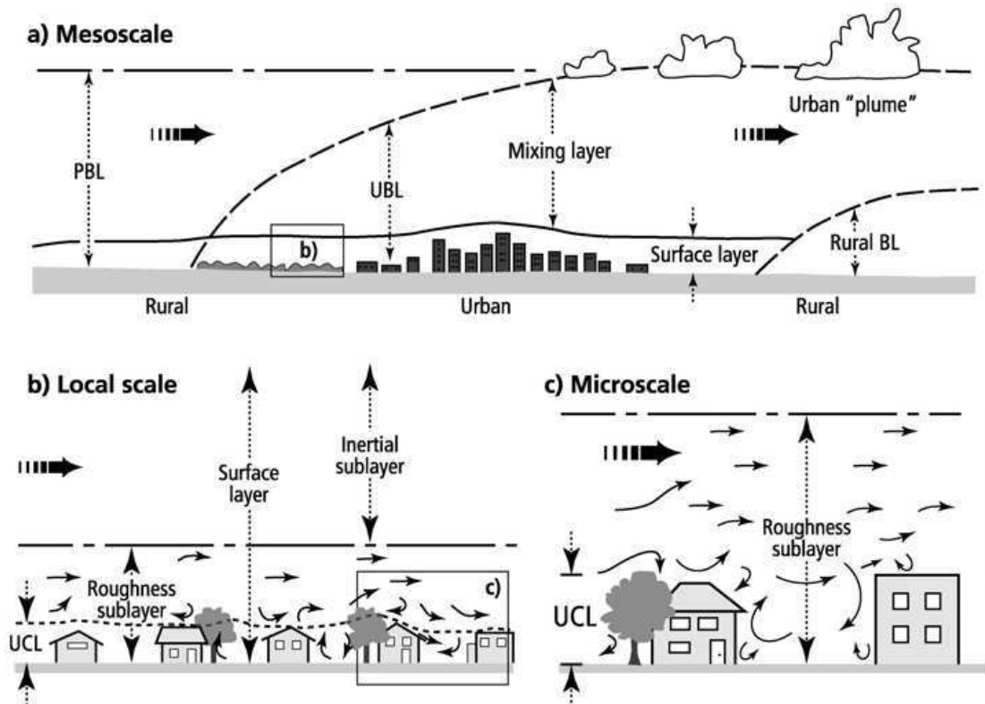
Figura 1: Esquema de escalas de clima e camadas verticais encontradas em áreas urbanas. PBL – Camada Limite Planetária, UBL – Camada Limite Urbana, UCL – Camada de Cobertura Urbana [modificado a partir de Oke, 1997].
