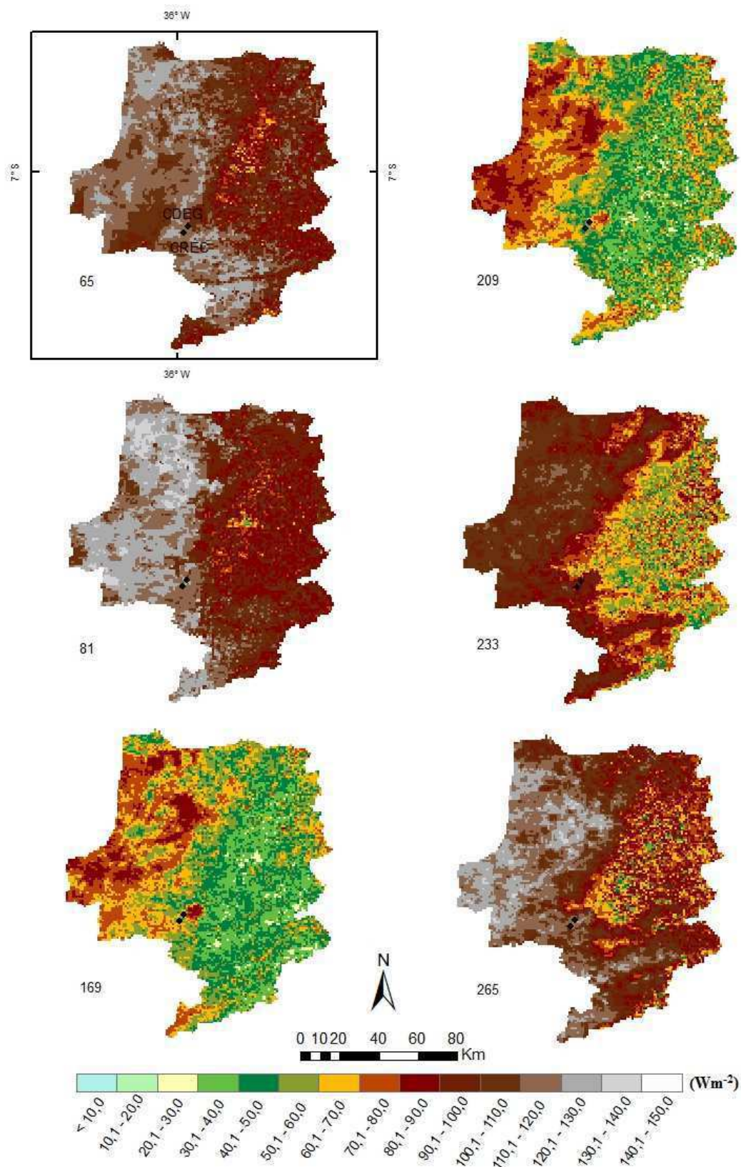
Figura 20: Fluxo de calor solo estimado a partir do Rn1 (G_1), em Wm^{-2} (Projeção: geográfica, Datum: WGS 84).
