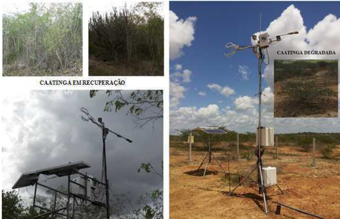
Figura 9: Torres de fluxo instaladas na área do experimento, em destaque as áreas de Caatinga em recuperação e degradada
