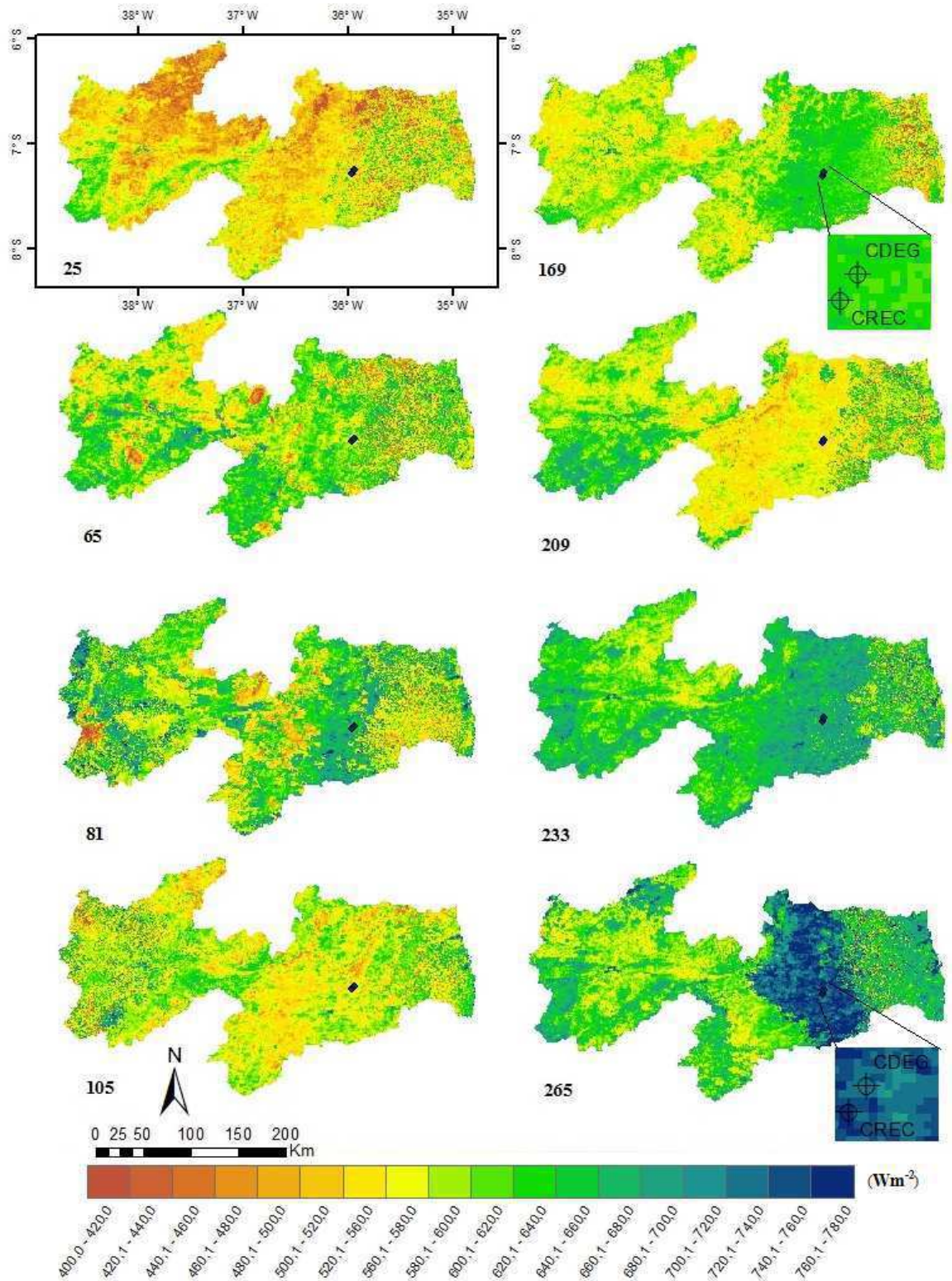
Figura 15: Cartas do saldo de radiação instantâneo ( \text{Wm}^{-2} ) obtidas através das metodologias SALDO1 para os dias de ordem do ano (DOA) 25, 65, 81, 105, 169, 209, 233, 265. Em destaque os pontos correspondentes às torres micrometeorológicas da área de Caatinga em recuperação - CREC e degradada - CDEG (Projeção: geográfica, Datum: WGS 84).
