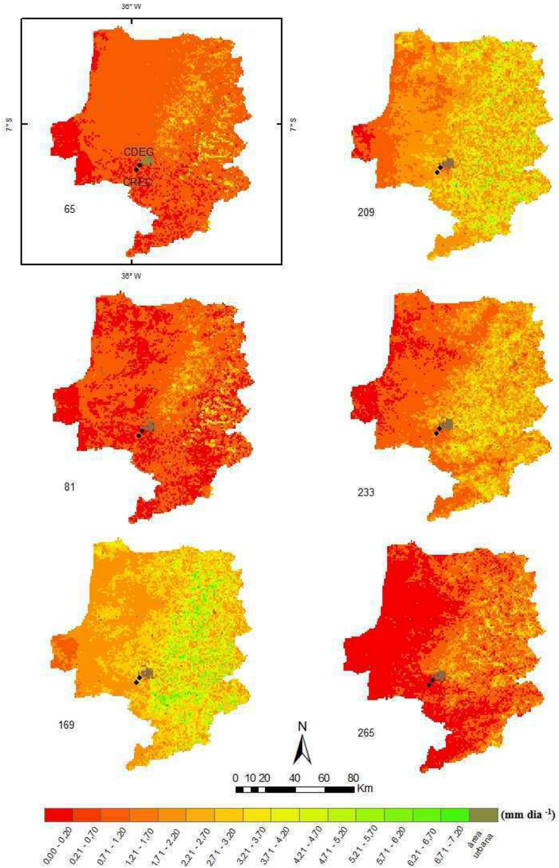
Figura 26: Distribuição espacial da evapotranspiração MOD16A2 ( \text{mm dia}^{-1} ), (Projeção: geográfica, Datum: WGS 84).
