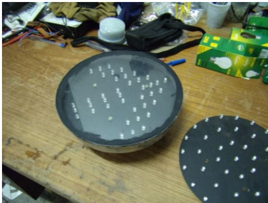
Figura 9 – Unidade Focal para LED's
