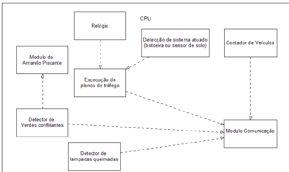
Figura 35 – Diagrama da estrutura da CPU do controlador de semáforo (SOUZA, 2008)
