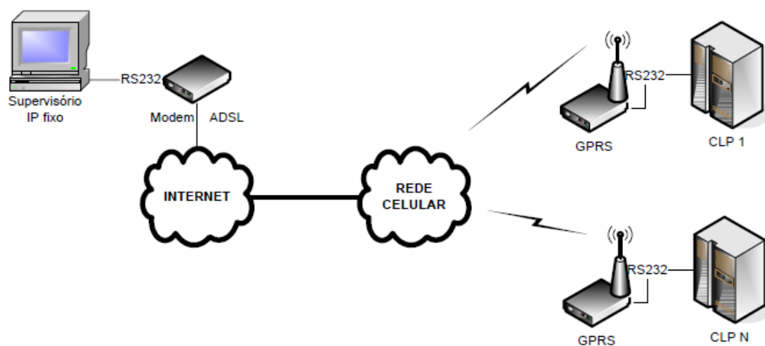
Figura 36 – Estrutura típica de comunicação entre os controladores e a central de controle através da rede GSM/GPRS
