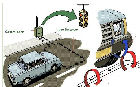
Figura 33 – Esquema de detecção por laço indutivo
