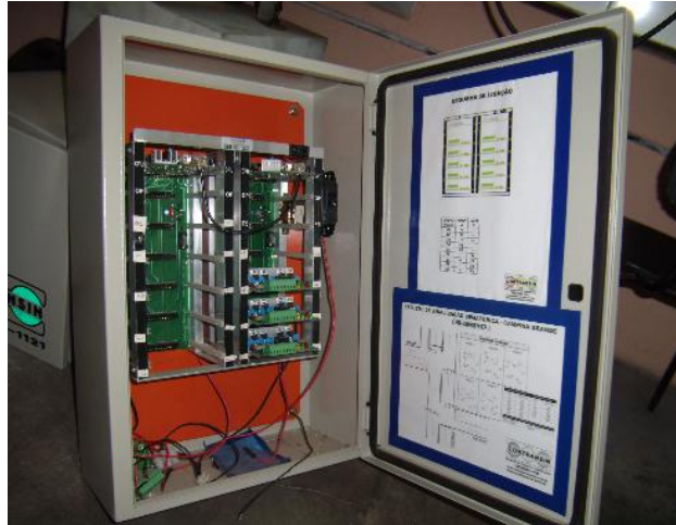
Figura 28 – Controlador da CONTRANSIN
