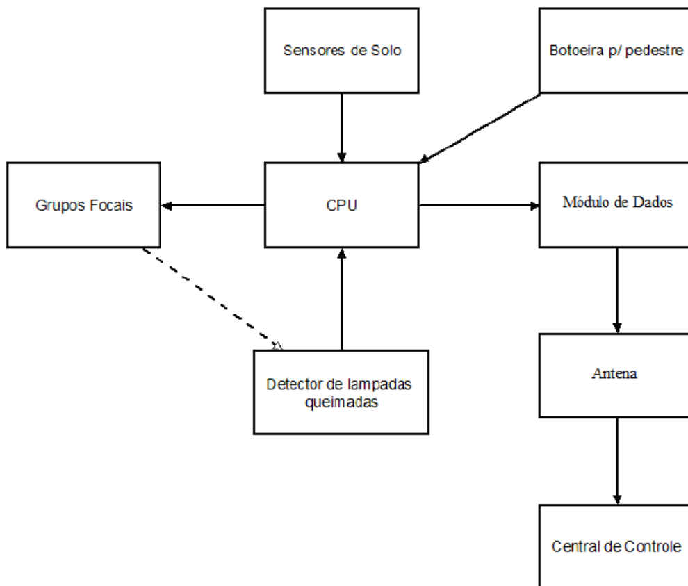
Figura 34 – Diagrama de blocos esquetizando a estrutura de um controlador e a central de controle (SOUZA, 2008).
