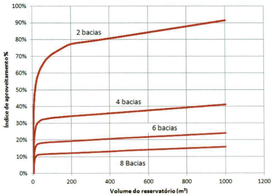
Figura 53 – Relação volume do reservatório e índice de aproveitamento do sistema para diferentes demandas de água.
