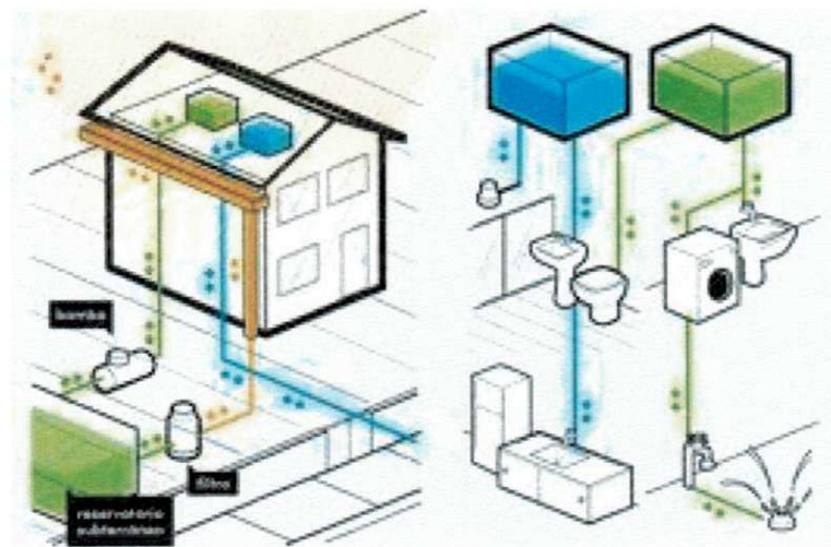
Figura 9– Esquema do sistema de captação de água chuva.
