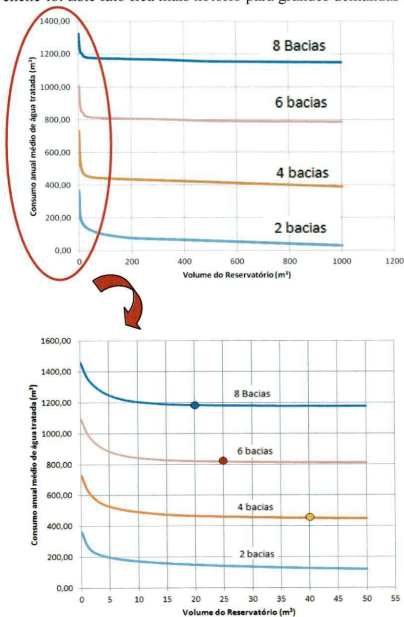
Figura 52 – Relação volume do reservatório e consumo de água tratada para diferentes demandas diárias. Abaixo, detalhe das curvas.
