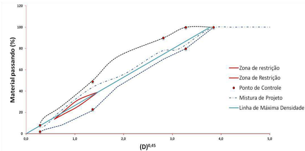
A4 - Curva fuller Método Francês - Agregado Laterítico
