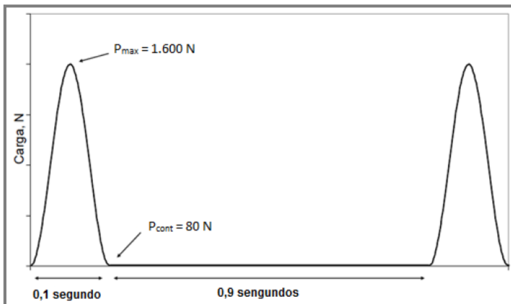
Figura 41 - Carregamento aplicado no ensaio uniaxial de carga repetida a 60°C.
