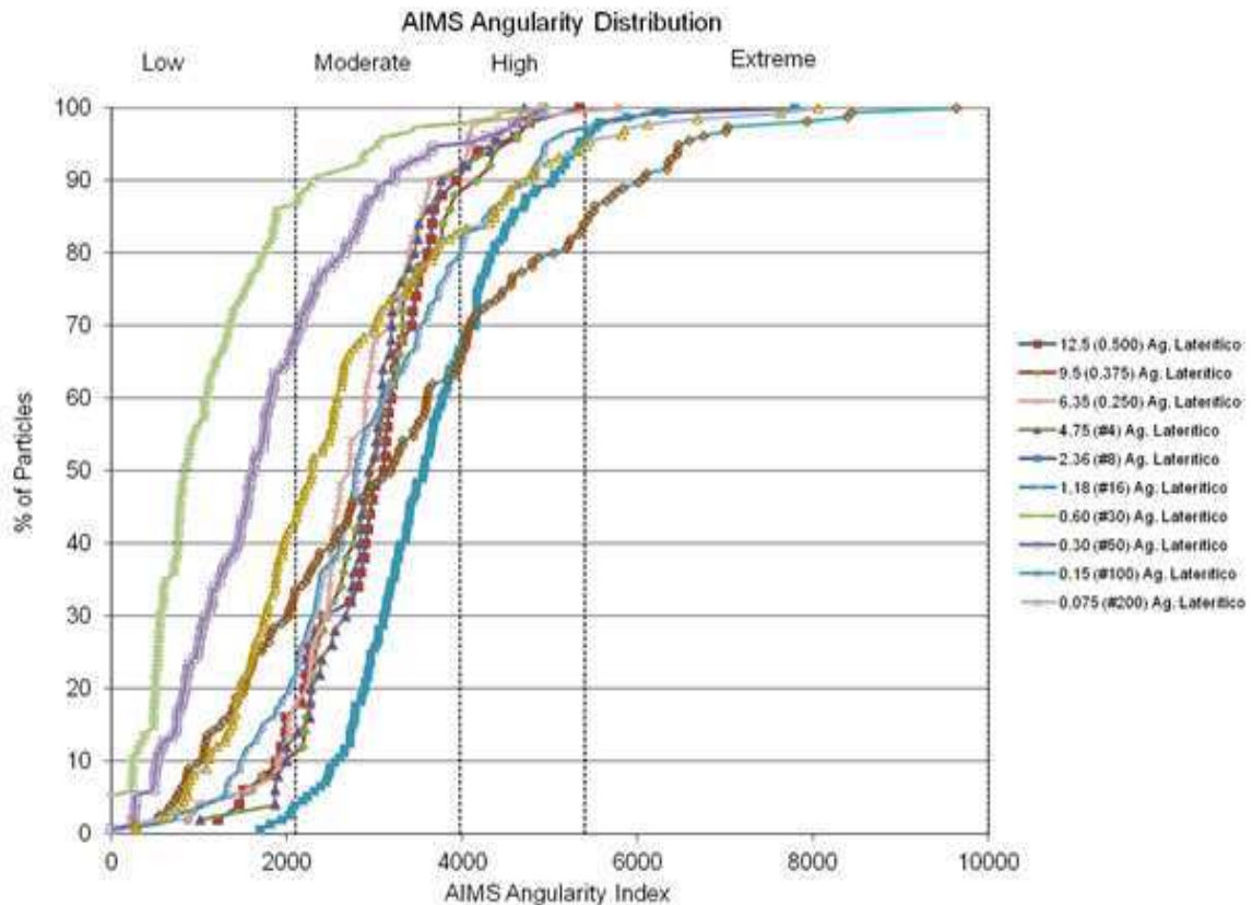
Figura 46 - Resultado do parâmetro angularidade para o agregado laterítico.
