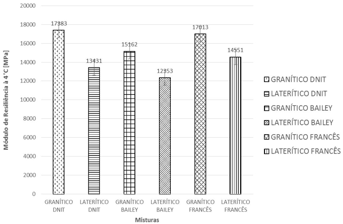
Figura 62 - Gráfico Módulo de Resiliência à 4°C × Tipo de Mistura.
