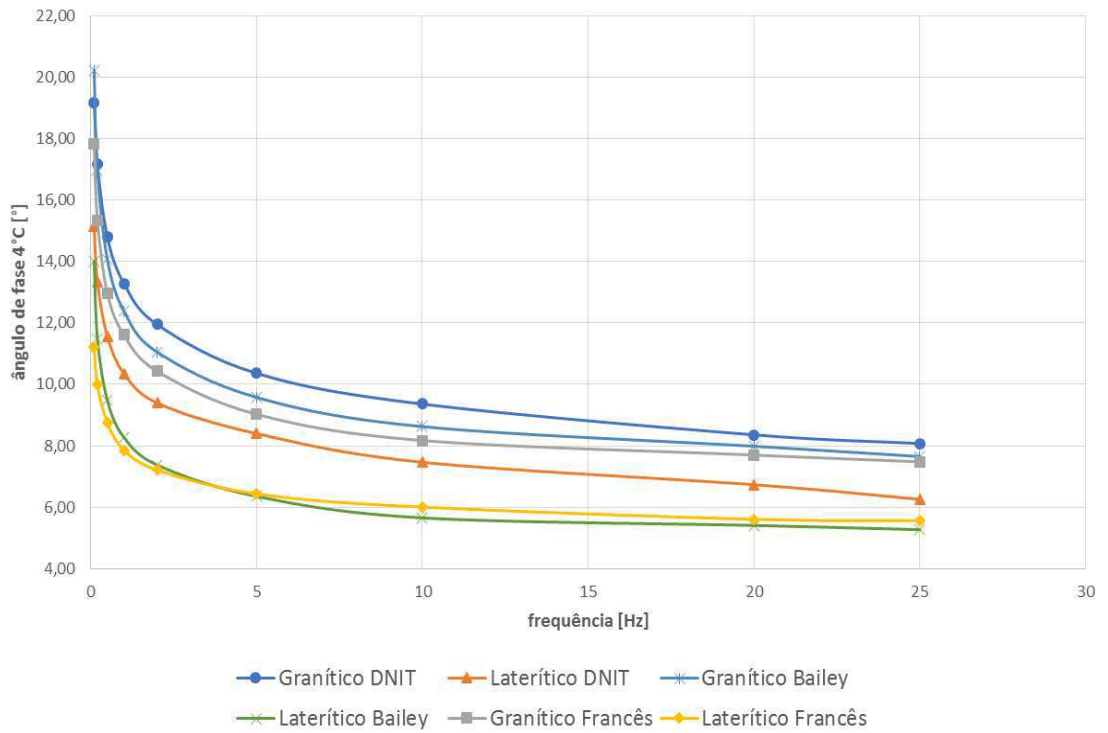
Figura 84 - Ângulos de Fase referentes as frequências de carregamento na temperatura de 4°C.
