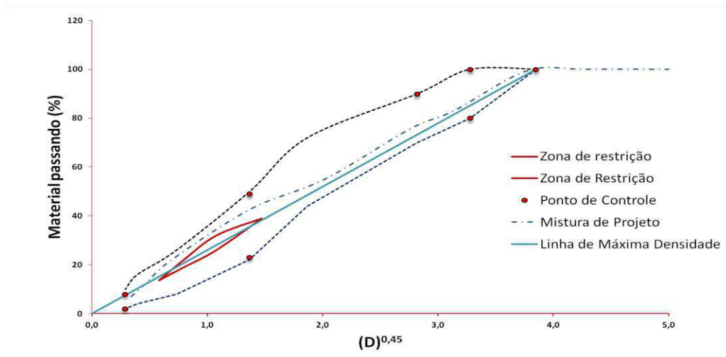
A3 - Curva fuller Método Francês - Agregado Granítico
