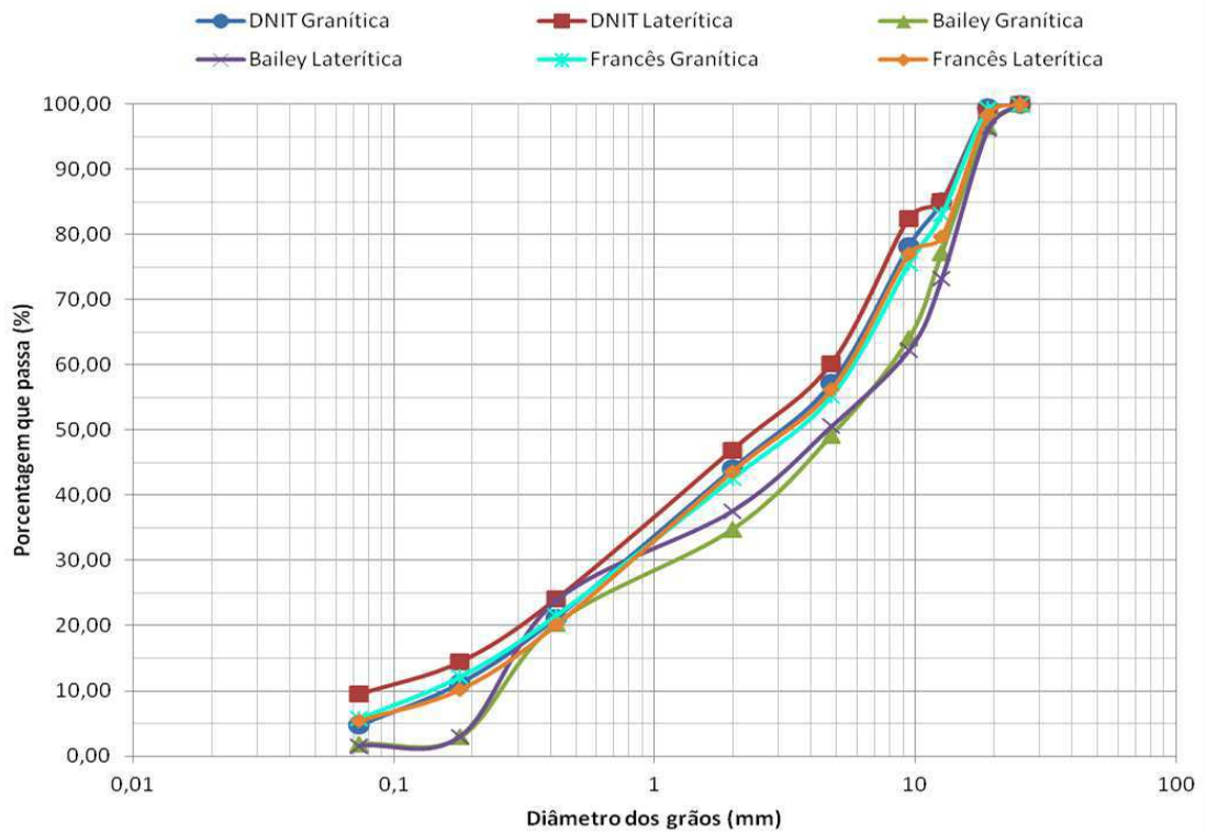
Figura 56 - Curvas granulométricas das misturas estudadas na pesquisa.
