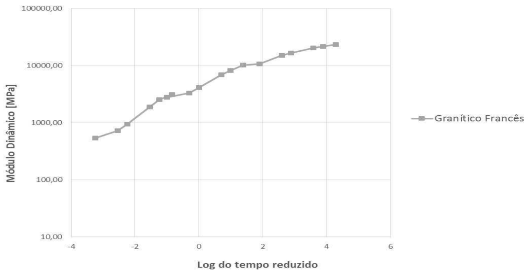
Figura 78 - Curva mestra da mistura Granítico Francês.
