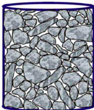
Figura 28 - Determinação da Massa Específica Compactada do Agregado Graúdo
