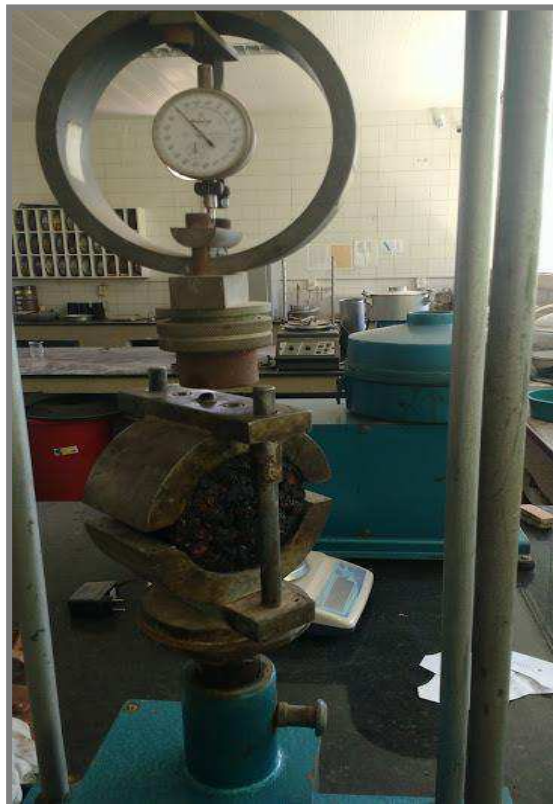
Figura 35 - Ensaio de Estabilidade Marshall.
