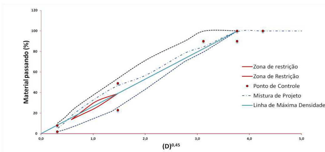
A2 - Curva fuller Método DNIT - Agregado Laterítico
