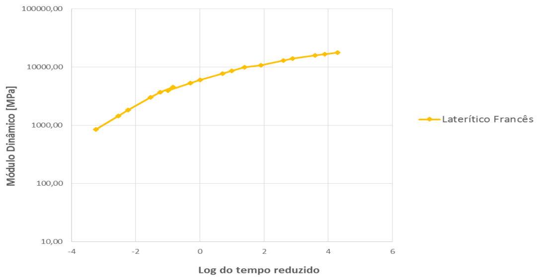
Figura 79 - Curva mestra da mistura Laterítico Francês.
