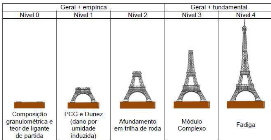
Figura 6 - Desenho esquemático da relação entre os níveis de projeto de misturas asfálticas do método francês e os respectivos ensaios
