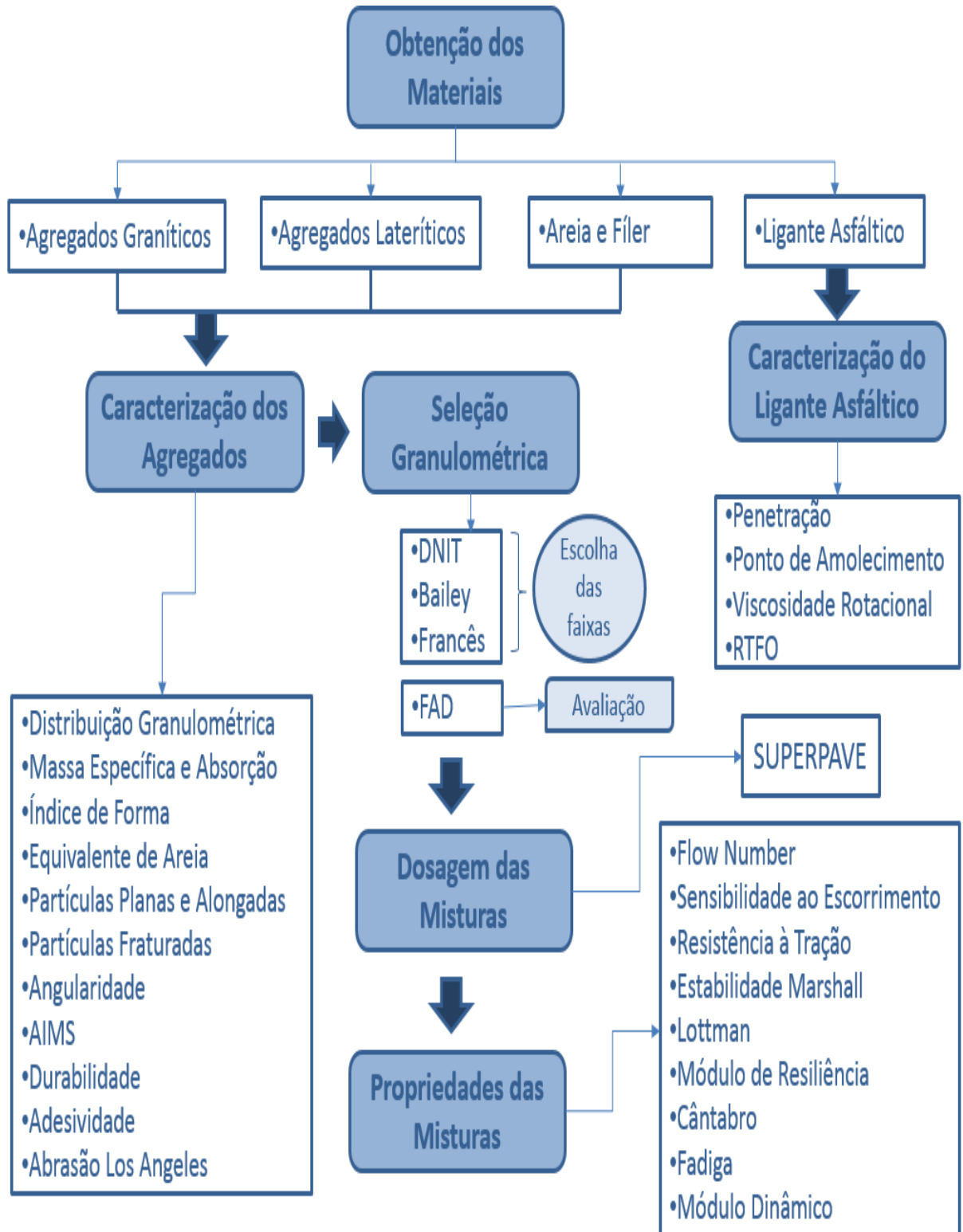
Figura 11 - Fluxograma do programa experimental da pesquisa.
