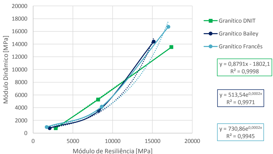
Figura 89 - Gráfico Módulo Dinâmico × Módulo de Resiliência para misturas utilizando agregados graníticos.
