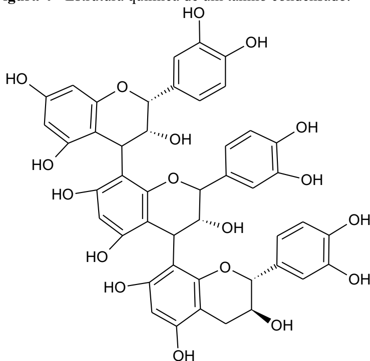
Figura 4 - Estrutura química de um tanino condensado.
