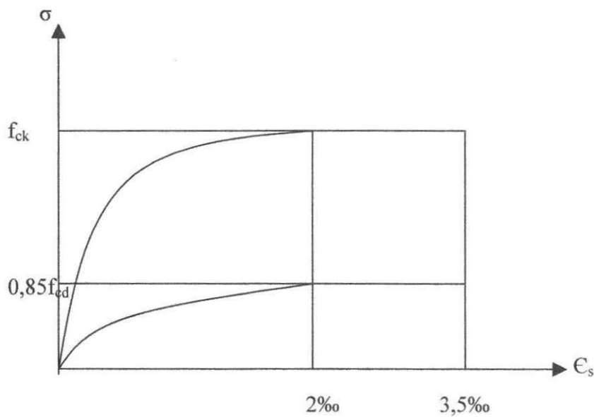
figura 3 – diagrama tensão-deformação
