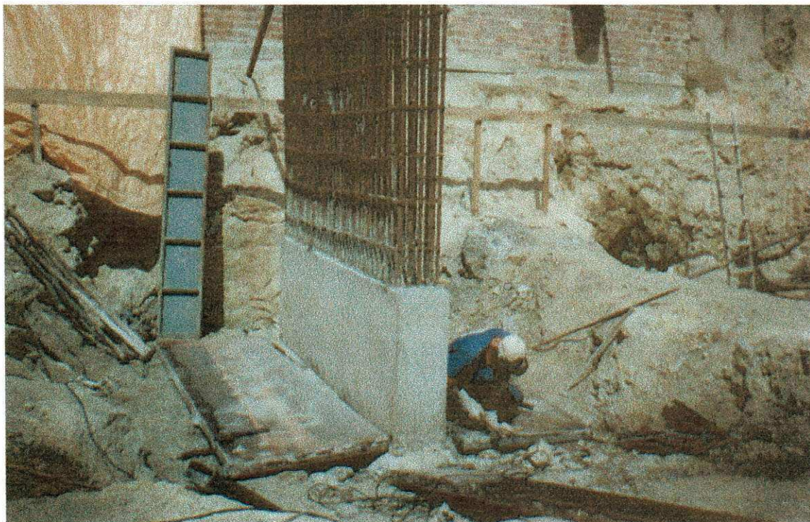
Foto 02: Desforma dos pilares
