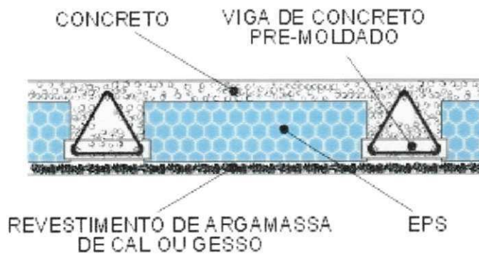
FIGURA 01 – Sistema concreto-vigota-blocos de EPS
