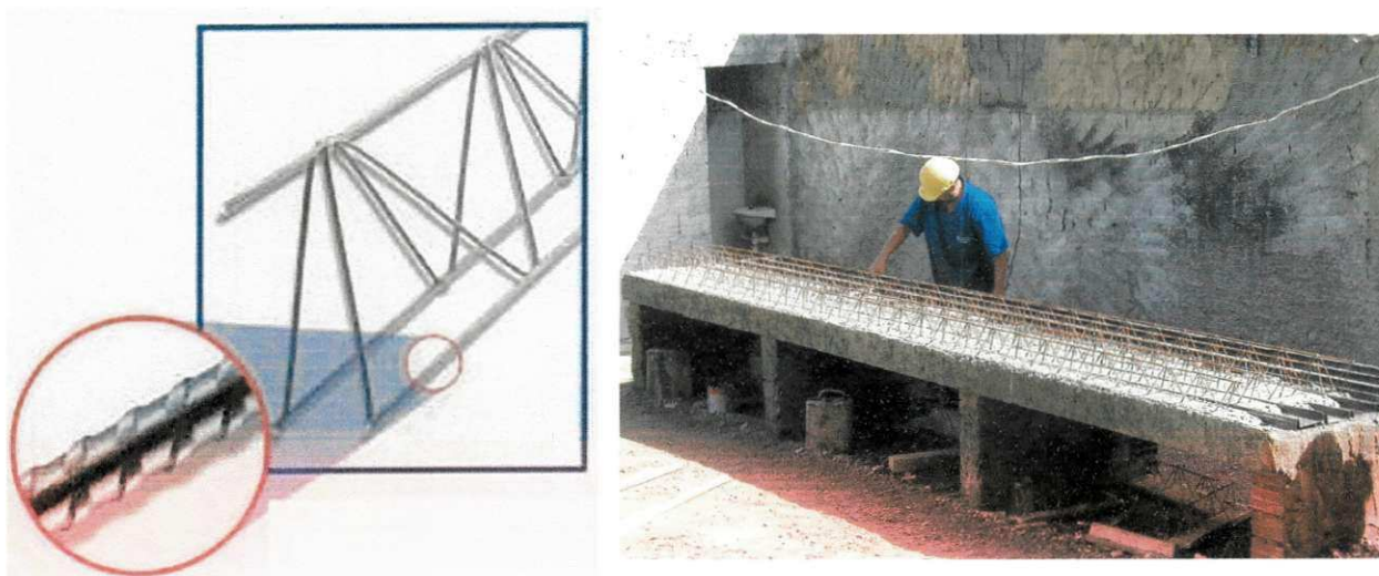
FIGURA 04 – Detalhe das nervuras na treliça e concretagem nas formas de perfis metálicos
