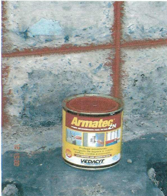
Foto 13 -Produto antioxidante utilizado nas armaduras
