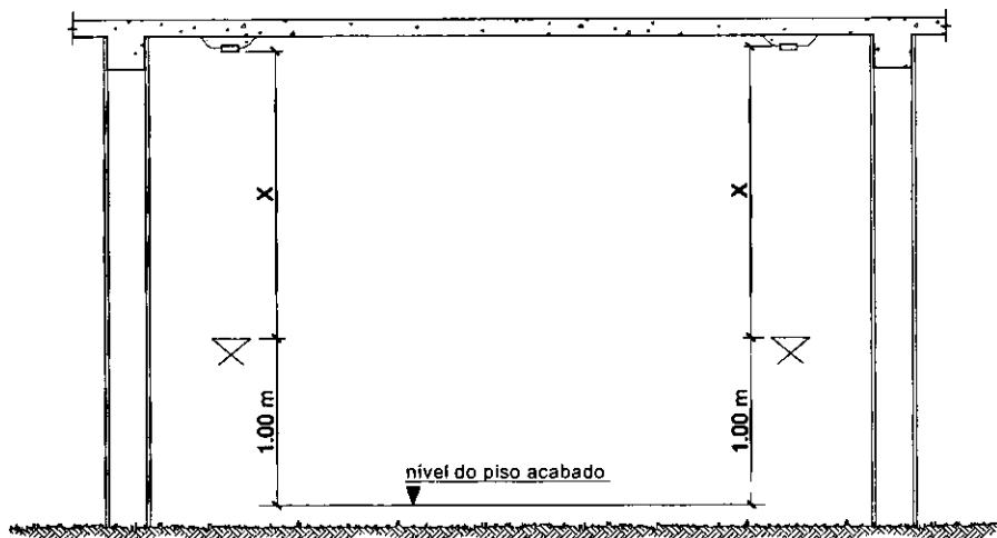
Figura 8 - Detalhe da colocação das taliscas nos tetos utilizando o nível referencial
