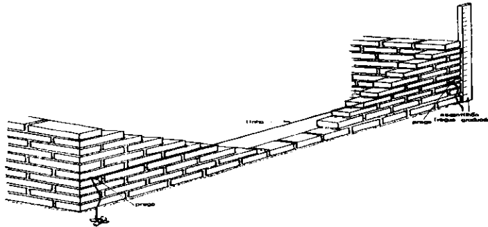
Figura 3 - Detalhe do nivelamento da elevação da alvenaria
