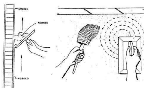
Figura 10 - Detalhe da aplicação do reboco
