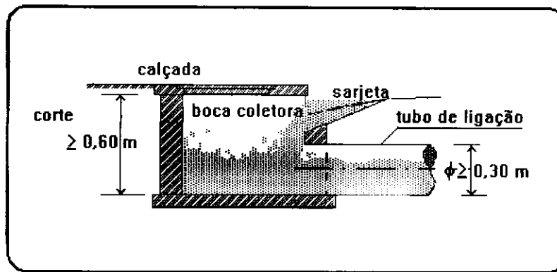
Desenho esquemático de uma boca de lobo.
