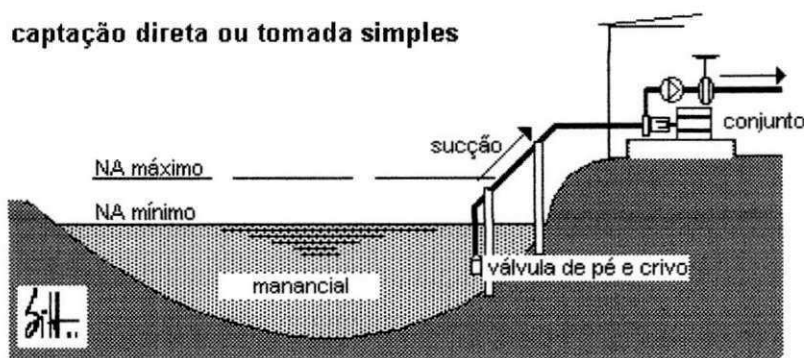
Desenho ilustrativo de captação direta ou tomada simples.
