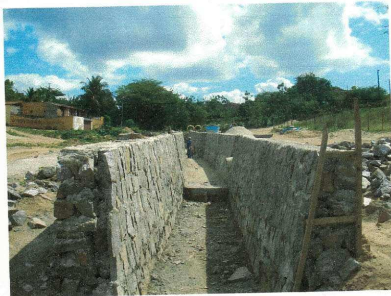
Figura 14 (Canais de macro – drenagem)
