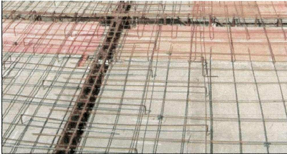
Figura 2. Distribuição do aço no encontro de duas lajes
