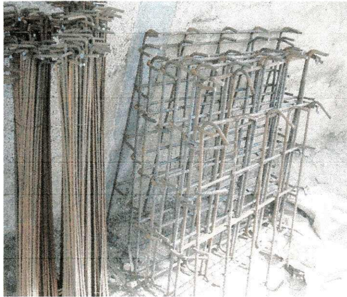
Figura 9. Lançamento do concreto magro (A) e grelhas para colocação sob sapatas (B).
