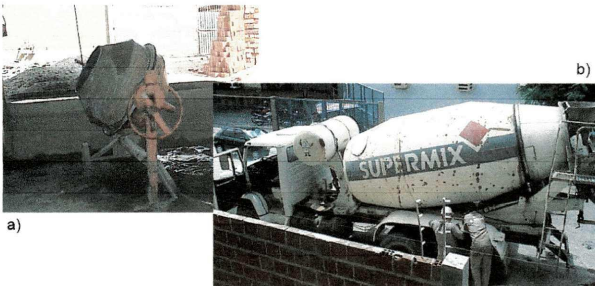
Figura 7. Equipamentos utilizados no processo de fabricação do concreto (Pinheiro, 2006).
