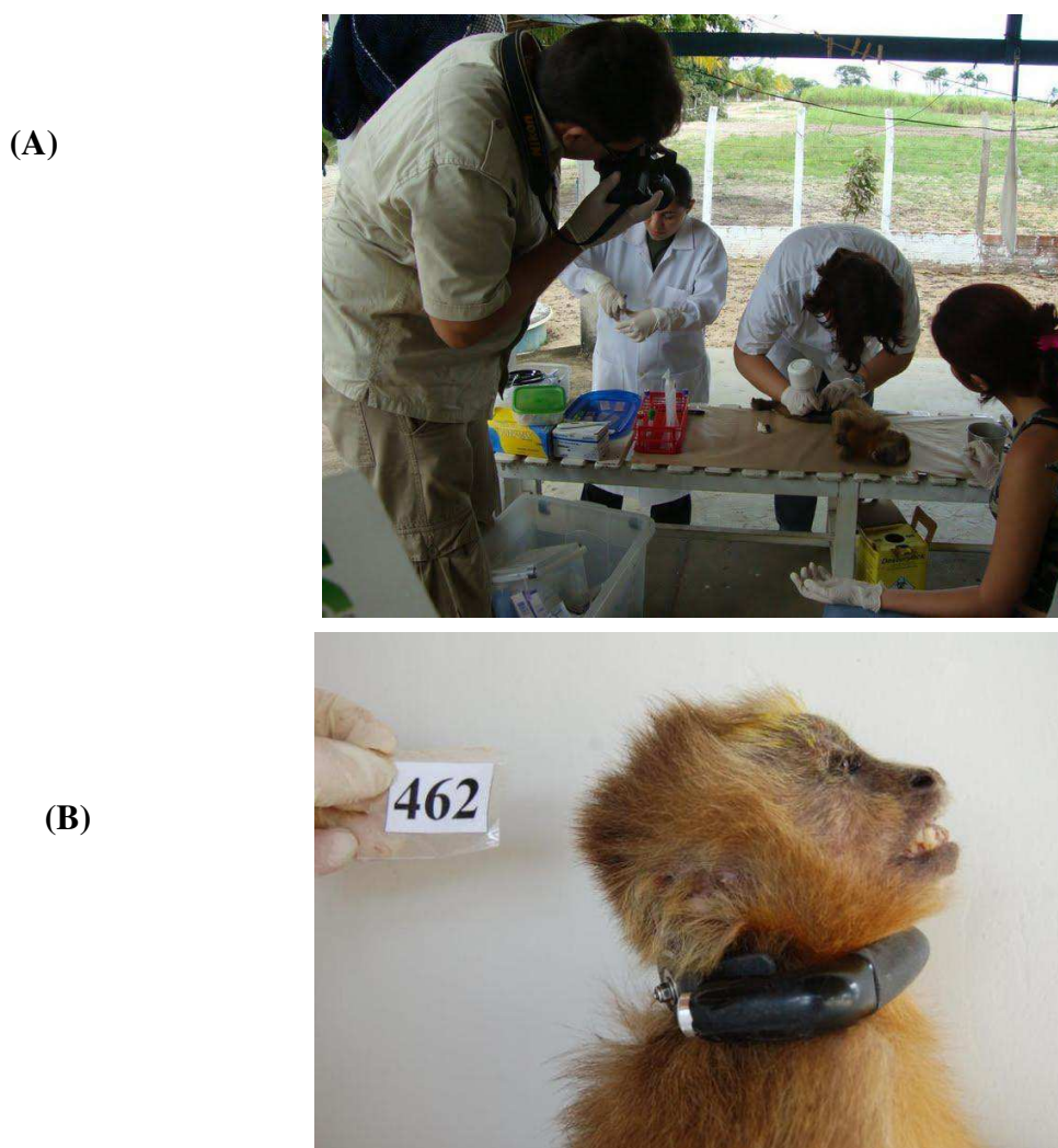
Figura 6: Processamento e colocação de rádio-colar em Cebus flavius em fragmento de Mata Atlântica em Mamanguape, PB: (A) processamento; (B) animal com o rádio-colar. Fotos: Alinny Santos (A) e Amely Martins (B).
