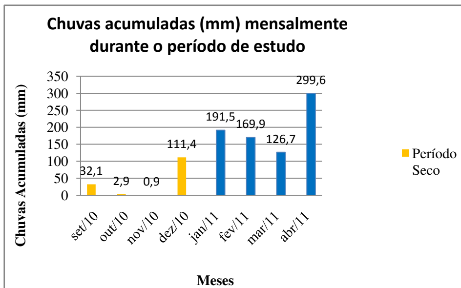
Figura 5: Chuvas acumuladas mensalmente no período de setembro de 2010 a abril de 2011 na área da Estação Experimental de Camaratuba, Mamanguape, PB. Em amarelo: período seco; em azul: período chuvoso. Fonte: AESA, 2011.
