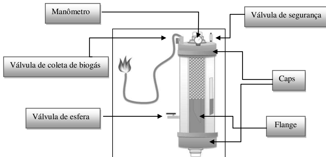
Figura 1 - Biorreator Monitorado
