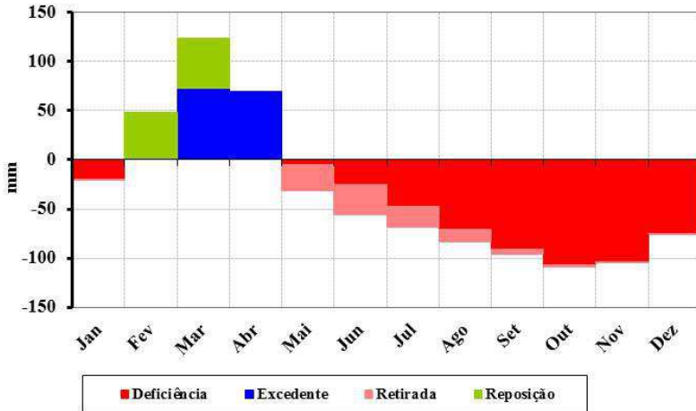
Figura 136. Balanço hídrico climatológico para o município de Nova Olinda.
