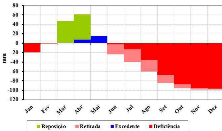
Figura 66. Balanço hídrico climatológico para o município de Caturité.
