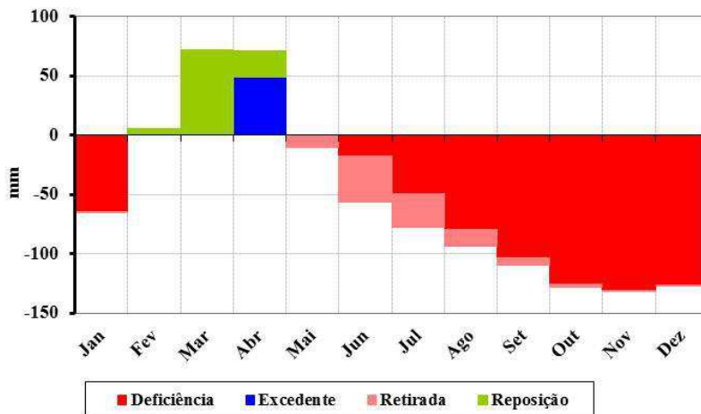
Figura 44. Balanço hídrico climatológico para o município de Brejo do Cruz.
