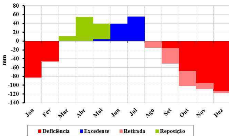
Figura 209. Balanço hídrico climatológico para o município de Serra da Raiz.
