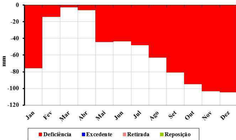
Figura 207. Balanço hídrico climatológico para o município de Seridó.
