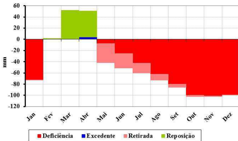
Figura 22. Balanço hídrico climatológico para o município de Areia de Baraúna.
