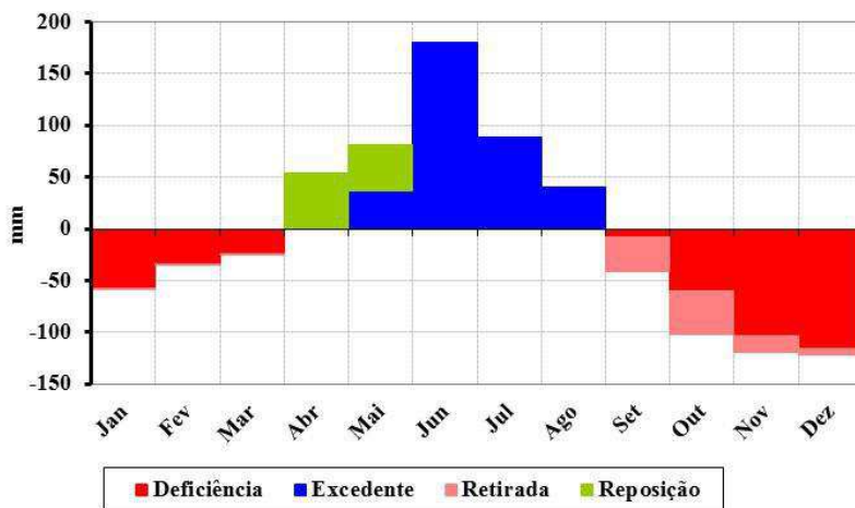
Figura 33. Balanço hídrico climatológico para o município de Bayeux.
