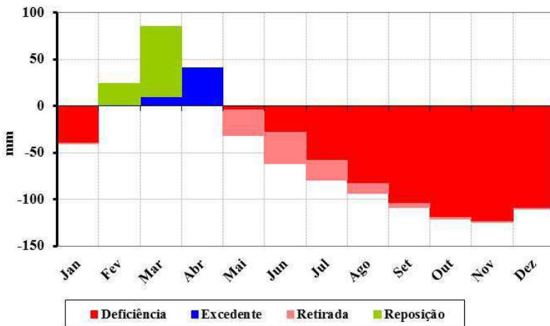
Figura 219. Balanço hídrico climatológico para o município de Sousa.
