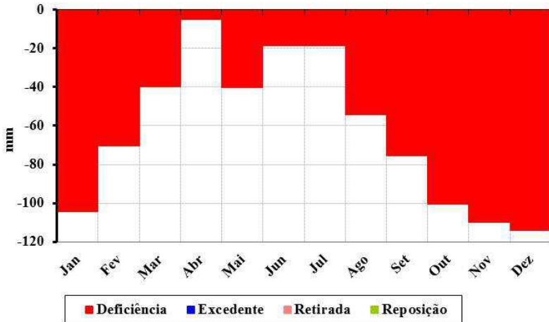
Figura 32. Balanço hídrico climatológico para o município de Barra de Santana.
