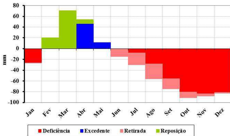
Figura 10. Balanço hídrico climatológico para o município de Araruna.
