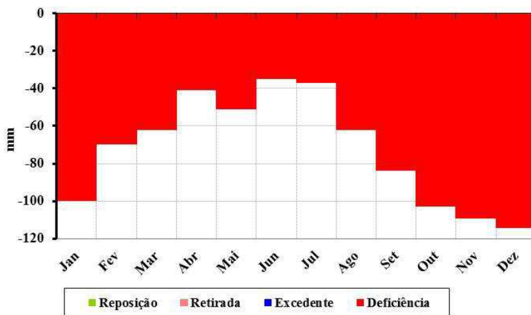
Figura 47. Balanço hídrico climatológico para o município de Cabaceiras.
