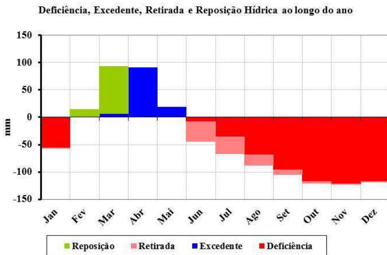
Figura 65. Balanço hídrico climatológico para o município de Catolé do Rocha.
