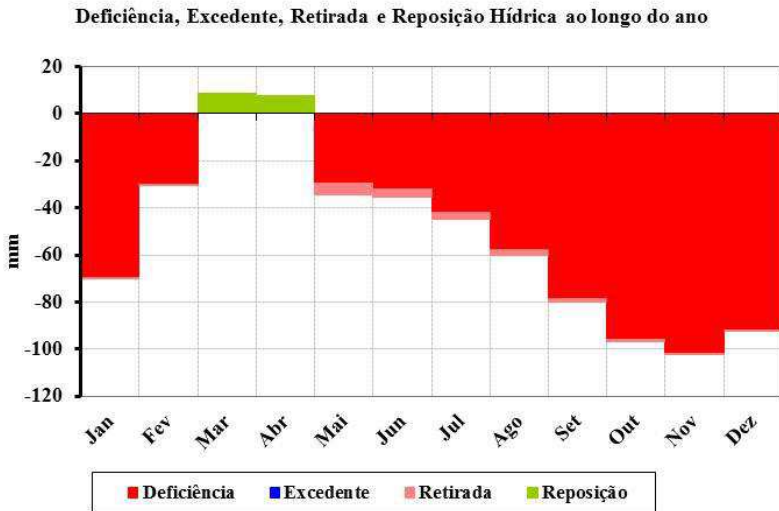
Figura 208. Balanço hídrico climatológico para o município de Serra Branca.
