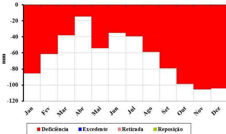
Figura 170. Balanço hídrico climatológico para o município de Riacho de Santo Antônio.
