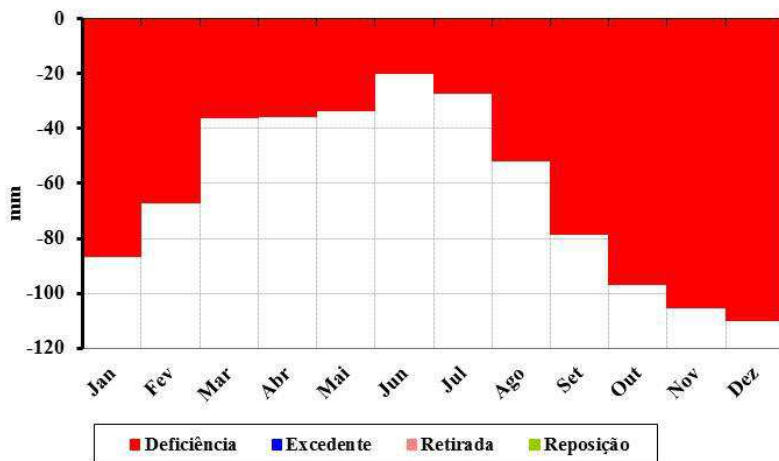
Figura 38. Balanço hídrico climatológico para o município de Boa Vista.
