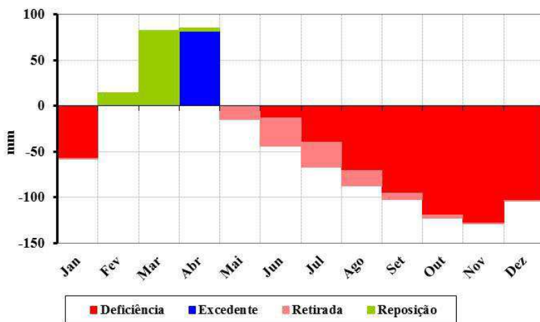
Figura 20. Balanço hídrico climatológico para o município de Araçagi.
