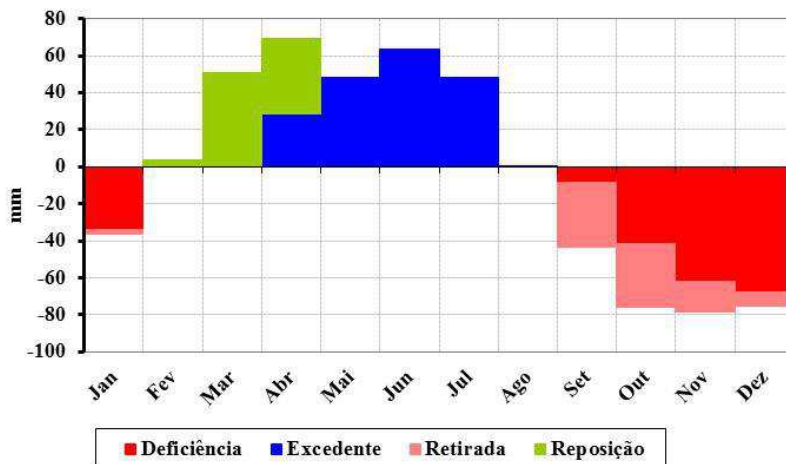
Figura 24. Balanço hídrico climatológico para o município de Areial.
