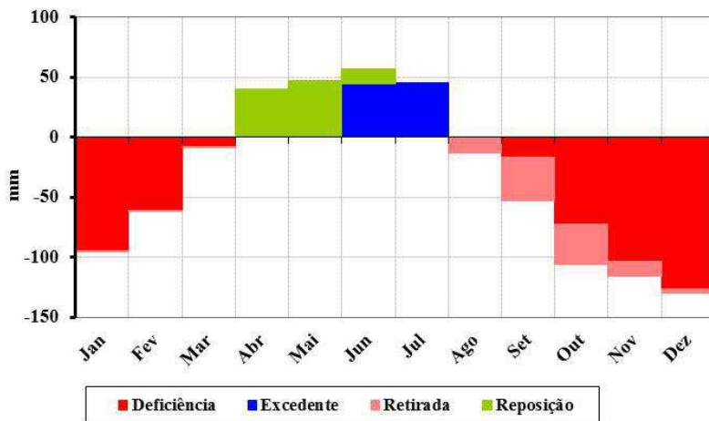
Figura 197. Balanço hídrico climatológico para o município de São Miguel de Taipu.
