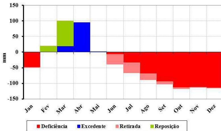
Figura 85. Balanço hídrico climatológico para o município de Emas.
