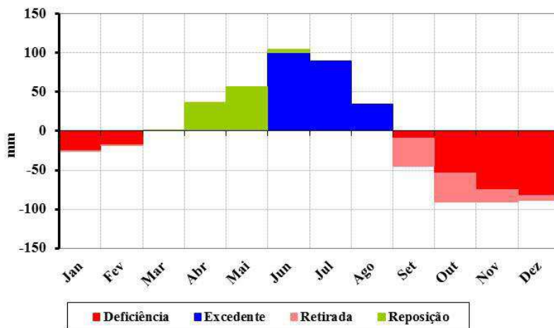
Figura 152. Balanço hídrico climatológico para o município de Pilões.
