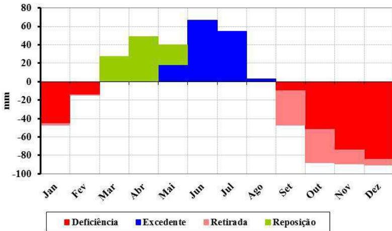
Figura 15. Balanço hídrico climatológico para o município de Alcantil.
