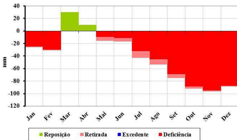
Figura 106. Balanço hídrico climatológico para o município de Junco do Seridó.
