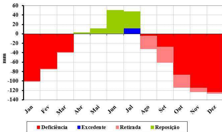
Figura 151. Balanço hídrico climatológico para o município de Pilar.
