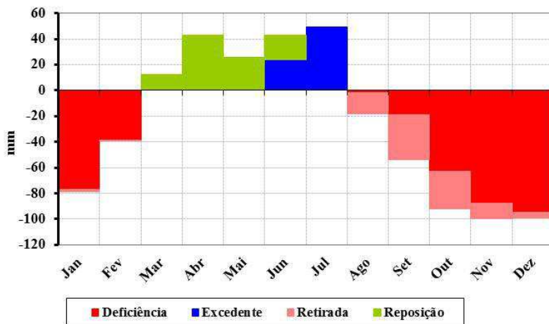
Figura 216. Balanço hídrico climatológico para o município de Solânea.
