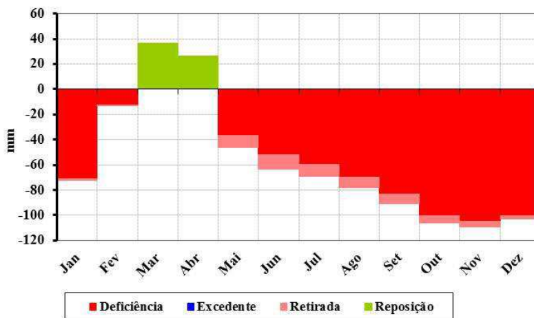
Figura 178. Balanço hídrico climatológico para o município de Santa Luzia.
