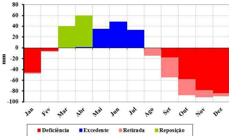
Figura 21. Balanço hídrico climatológico para o município de Arara.
