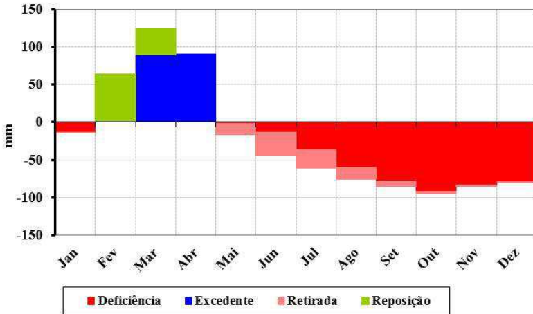
Figura 201. Balanço hídrico climatológico para o município de São João de Caiana.
