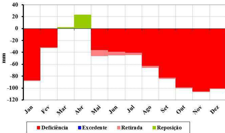
Figura 141. Balanço hídrico climatológico para o município de Parari.
