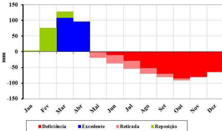
Figura 130. Balanço hídrico climatológico para o município de Monte Horebe.
