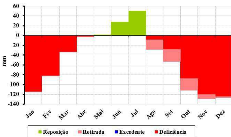
Figura 56. Balanço hídrico climatológico para o município de Caldas Brandão.
