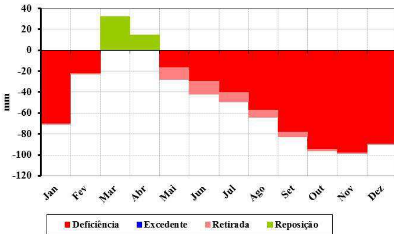
Figura 221. Balanço hídrico climatológico para o município de Taperoá.
