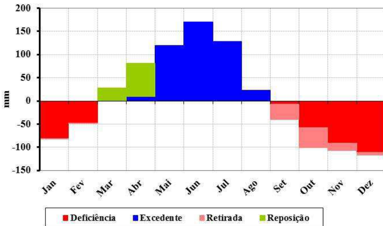
Figura 171. Balanço hídrico climatológico para o município de Rio Tinto.
