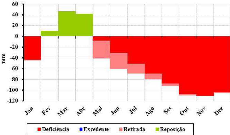
Figura 142. Balanço hídrico climatológico para o município de Passagem.
