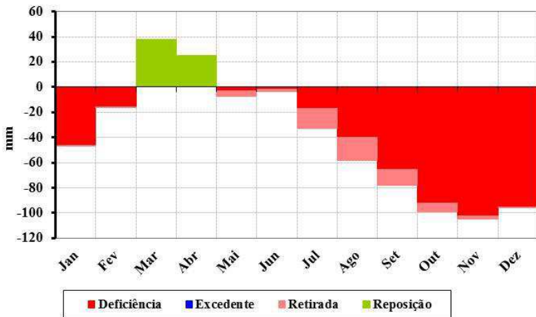
Figura 220. Balanço hídrico climatológico para o município de Sumé.
