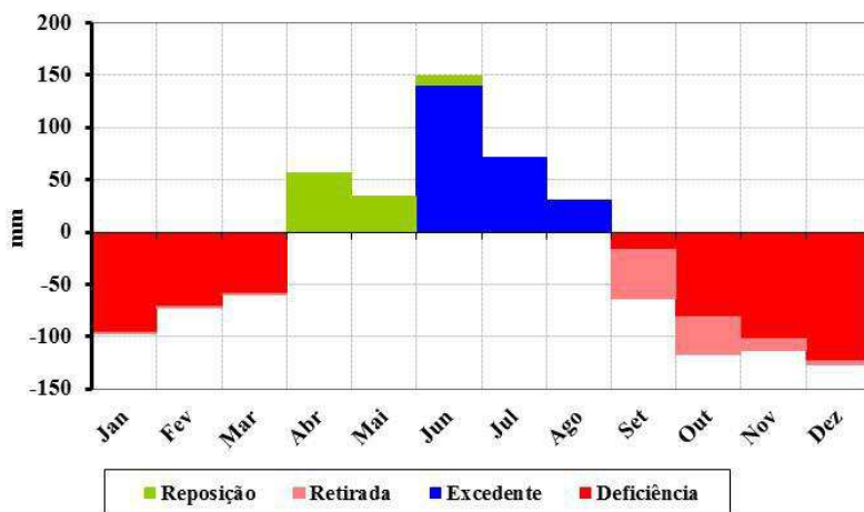
Figura 60. Balanço hídrico climatológico para o município de Capim.
