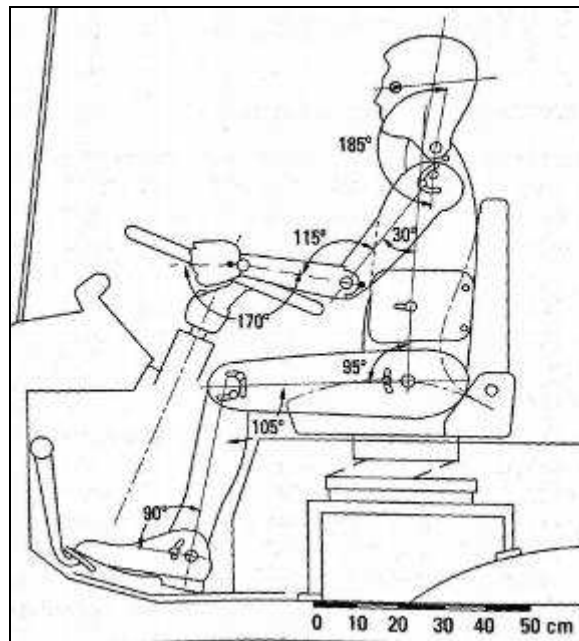
Figura 2 - Aspectos biomecânicos – postura e gabarito antropométrico.
