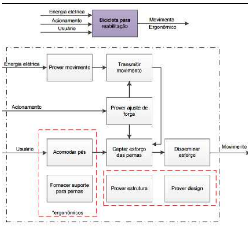
Figura 6 - Modelo funcional - Projeto bicicleta para reabilitação.
