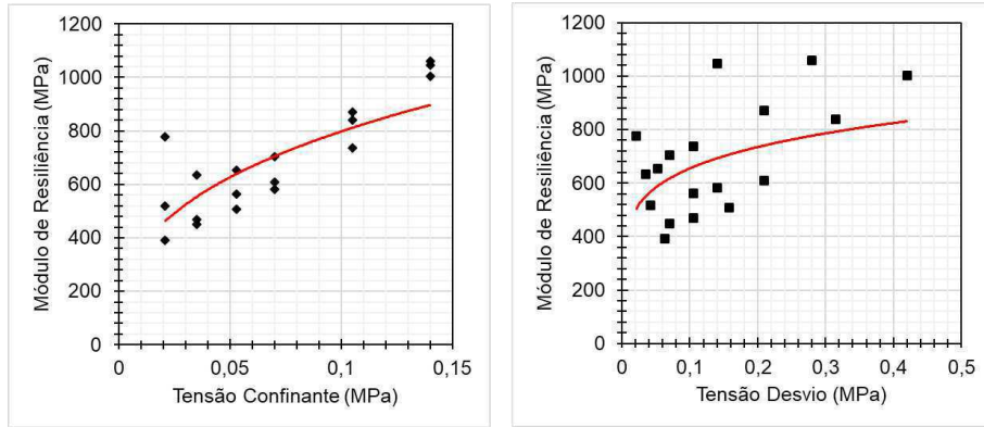
Figura 177: Curvas de ajuste usando os modelos \sigma_3 e \sigma_d para o solo BSB-3
