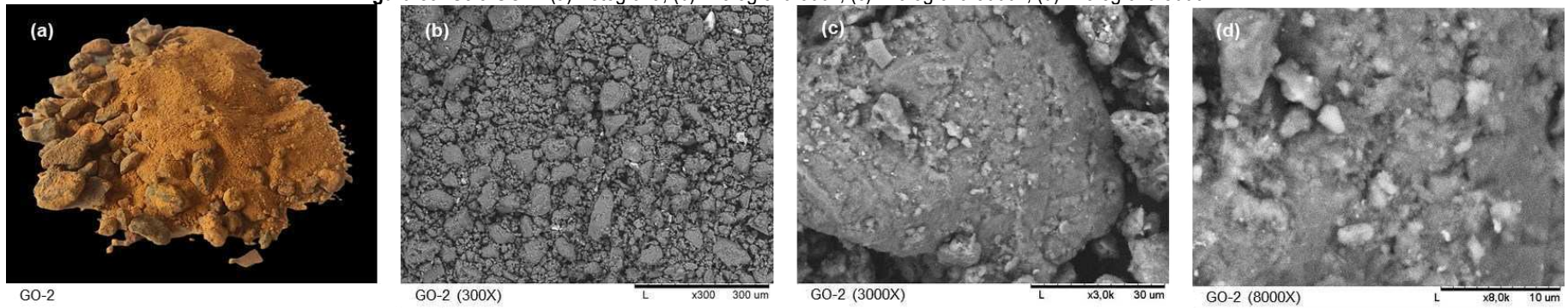
Figura 89: Solo GO-2: (a) Fotografia; (b) Micrografia 300x; (c) Micrografia 3000x; (d) Micrografia 8000x
