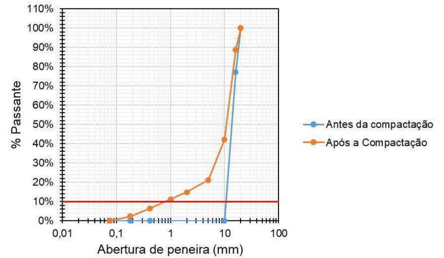
Figura 156: Ensaio de fragmentabilidade do solo PB-3
