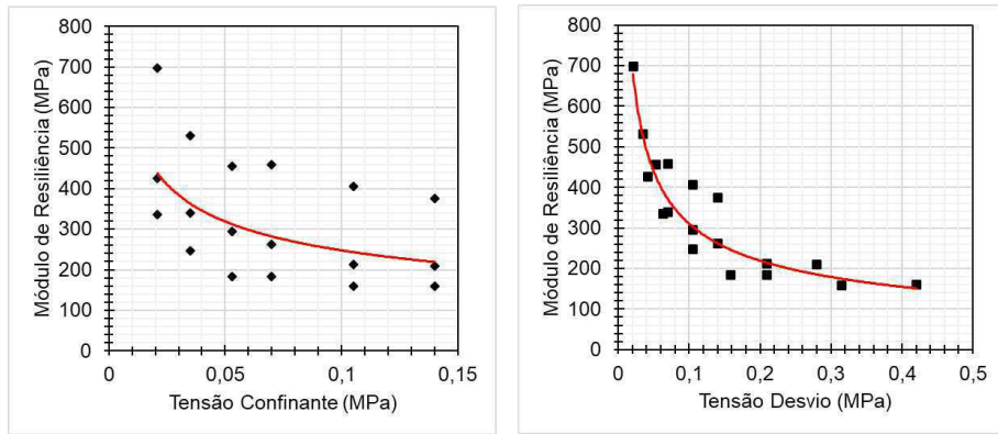
Figura 181: Curvas de ajuste usando os modelos \sigma_3 e \sigma_d para o solo GO-1
