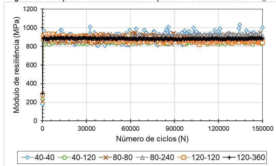
Figura 253: Variação do módulo resiliente em função do número de ciclos. Solo PB-3_2%
