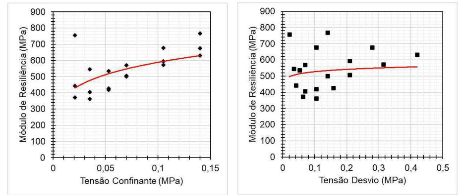
Figura 183: Curvas de ajuste usando os modelos \sigma_3 e \sigma_d para o solo GO-2
