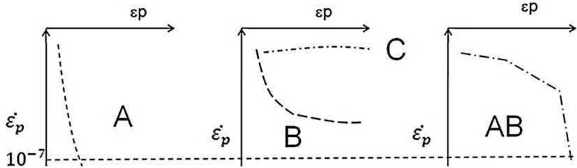
Figura 18: Modelos de comportamento a deformação permanente de solos: Análise do acomodamento ( shakedown )
