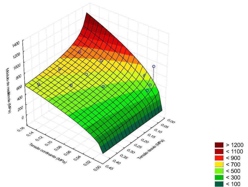
Figura 184: Superfície de ajuste usando o modelo composto para o solo GO-2
