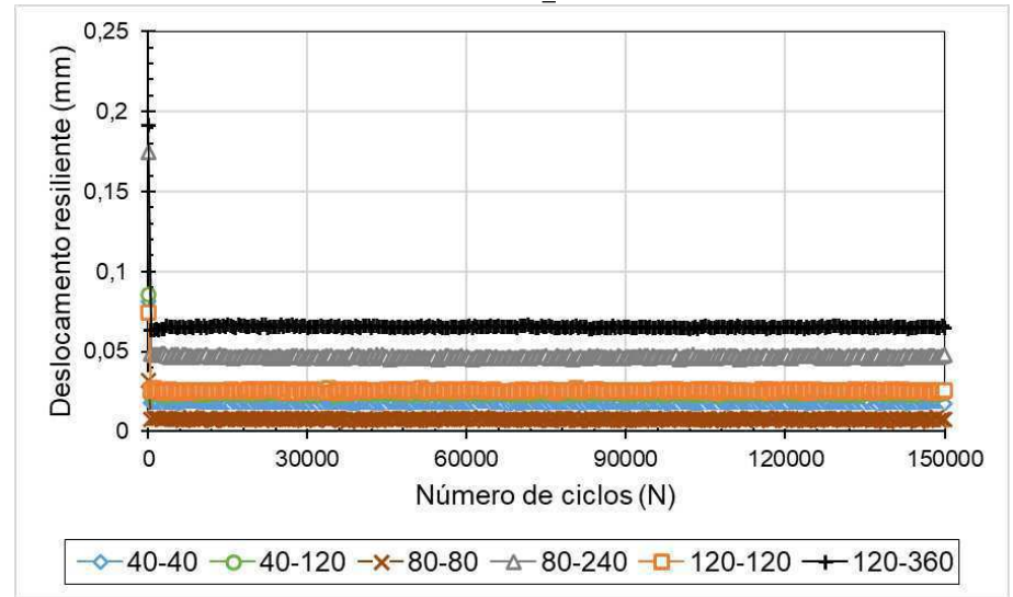
Figura 248: Deslocamento (a) e deformação (b) resilientes em função do número de ciclos. Solo PB-2_2%
