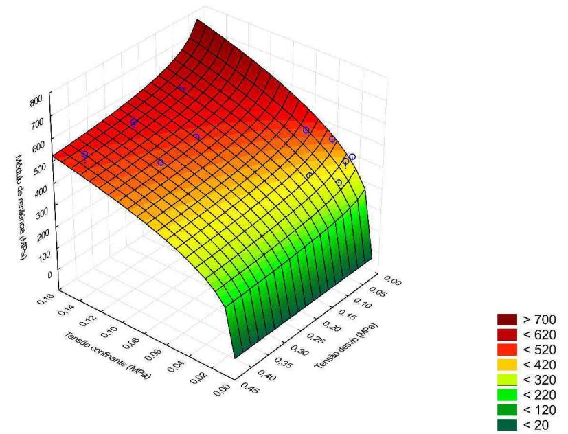
Figura 180: Superfície de ajuste usando o modelo composto para o solo BSB-4
