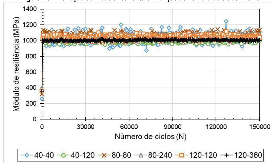
Figura 254: Variação do módulo resiliente em função do número de ciclos. BGTC
