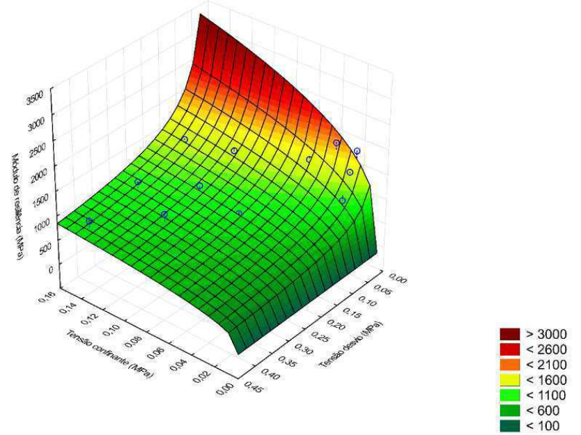
Figura 176: Superfície de ajuste usando o modelo composto para o solo BSB-2
