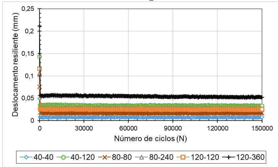
Figura 247: Deslocamento (a) e deformação (b) resilientes em função do número de ciclos. Solo PE-1_2%
