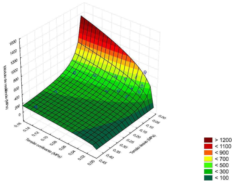
Figura 182: Superfície de ajuste usando o modelo composto para o solo GO-1
