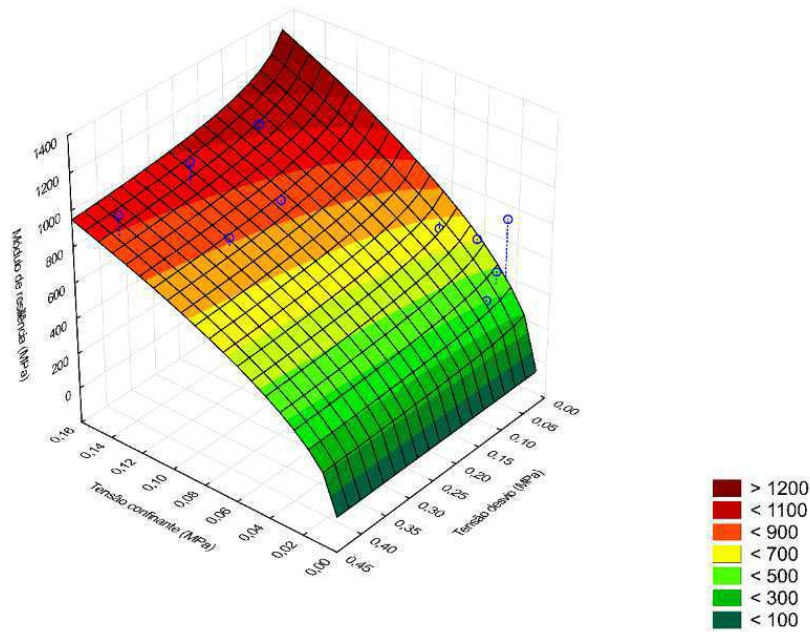
Figura 178: Superfície de ajuste usando o modelo composto para o solo BSB-3
