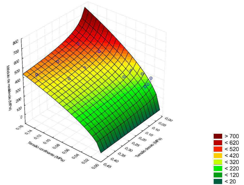
Figura 192: Superfície de ajuste usando o modelo composto para o solo GO-6
