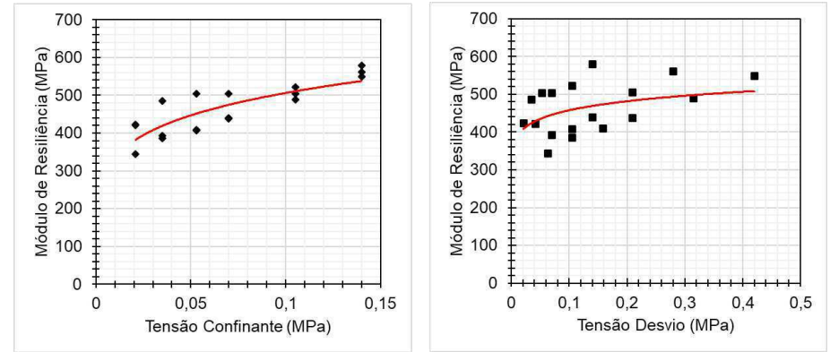
Figura 179: Curvas de ajuste usando os modelos \sigma_3 e \sigma_d para o solo BSB-4
