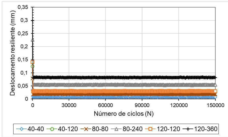
Figura 233: Deslocamento (a) e deformação (b) resilientes em função do número de ciclos. Solo PB-3
