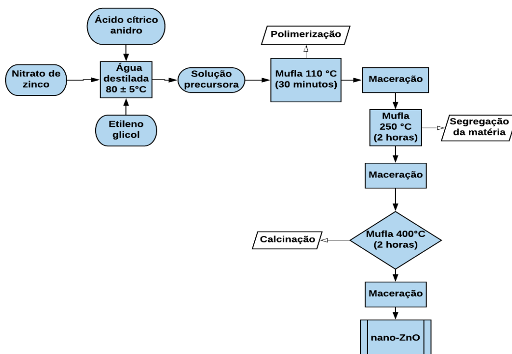
Figura 22 - Fluxograma das etapas de sintetização de nano-ZnO
