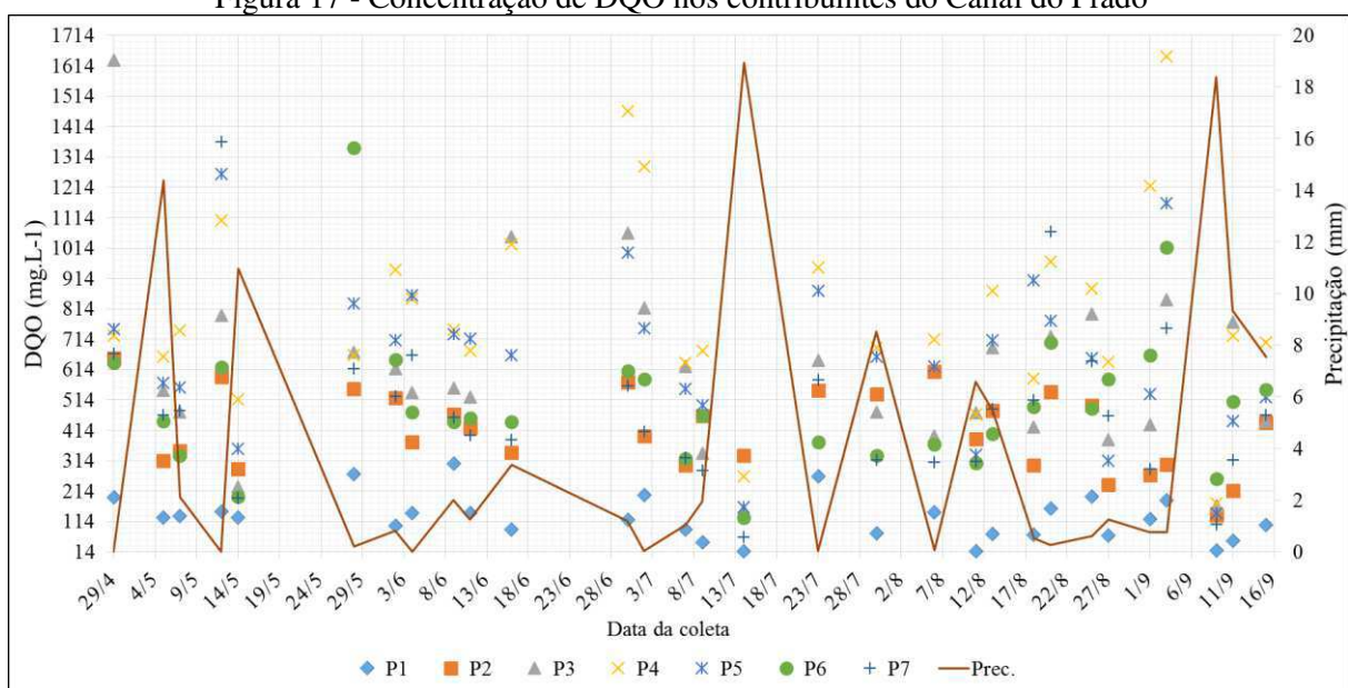
Figura 17 - Concentração de DQO nos contribuintes do Canal do Prado
