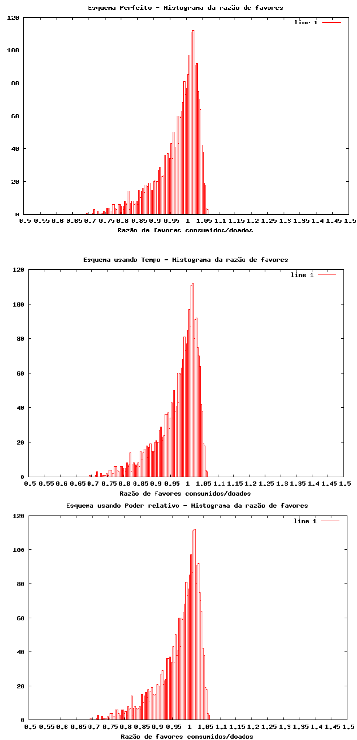
Figura 8. Histogramas da razão de favores para os esquemas de contabilidade no cenário 1.
