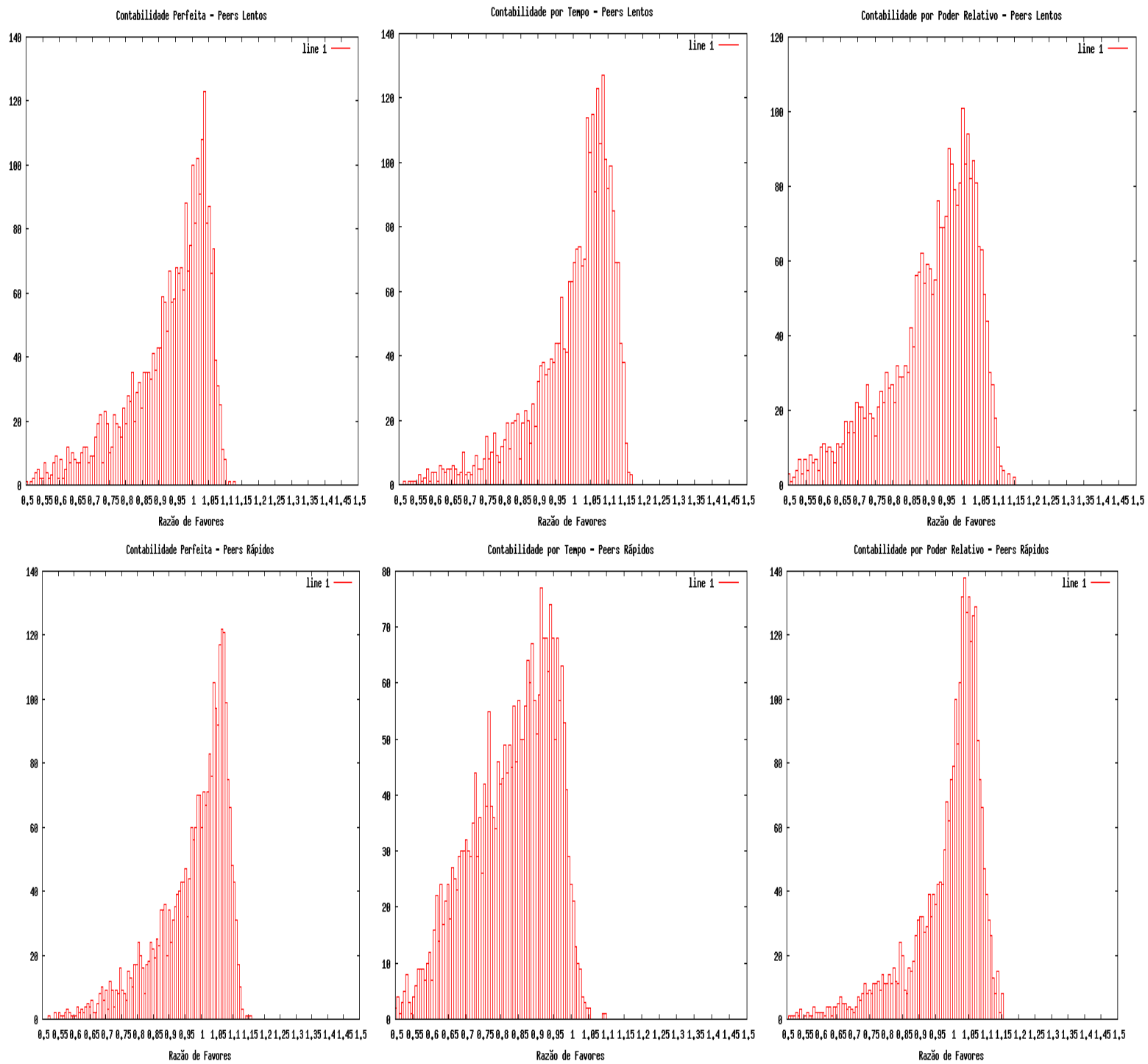
Figura 11. Histograma da razão de favores para esquemas de contabilidade no cenário 4.
