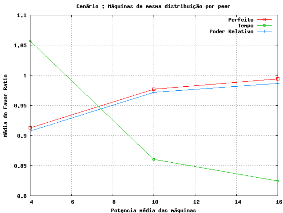
Figura 16. Evolução da média da razão de favores de acordo com o poder das máquinas do peer no cenário 6.
