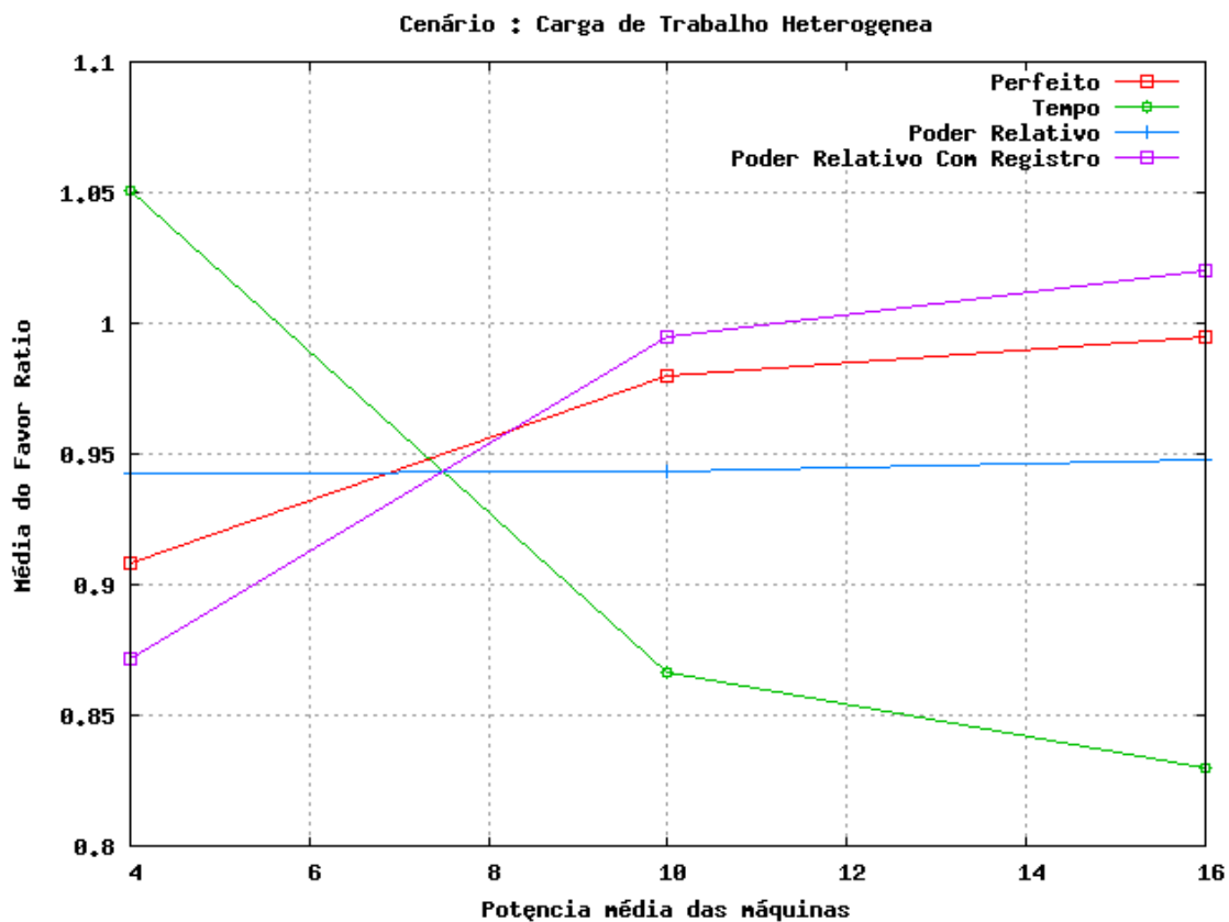
Figura 18. Evolução da média da razão de favores de acordo com o poder das máquinas do peer no cenário 7.
