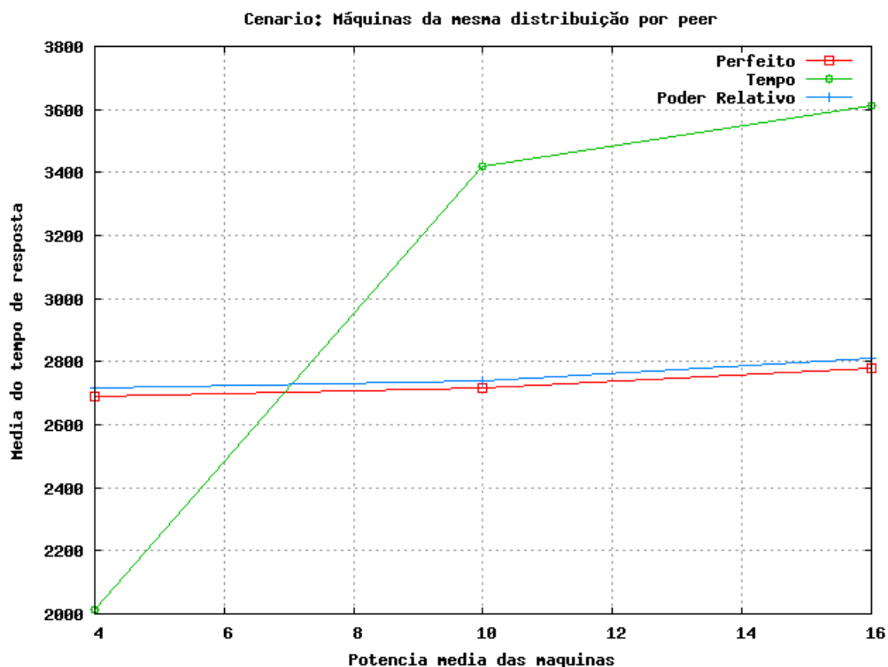
Figura 15. Evolução do tempo de resposta das aplicações de acordo com o poder das máquinas do peer no cenário 6.
