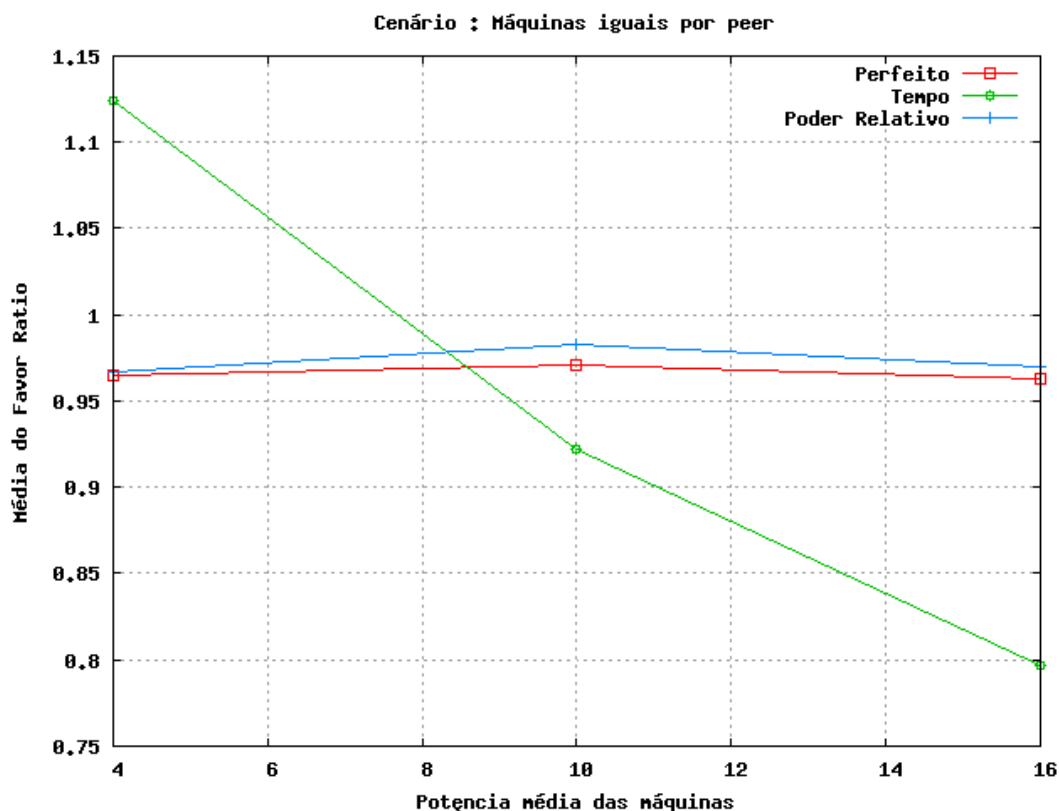
Figura 14. Evolução da média da razão de favores de acordo com o poder das máquinas do peer no cenário 5.
