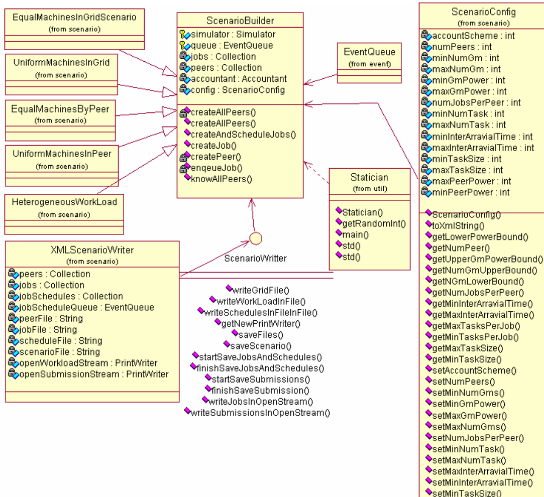
Figura 4. Núcleo do diagrama de classes do gerador de cenários.
