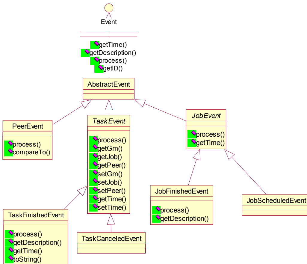
Figura 6. Eventos do simulador.
