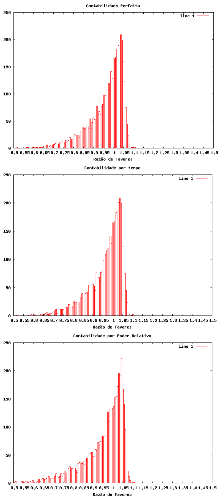
Figura 9. Histogramas da razão de favores para os esquemas de contabilidade no cenário 2.
