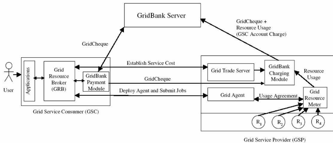
Figura 1. Protocolo de funcionamento do GridBank [7].
