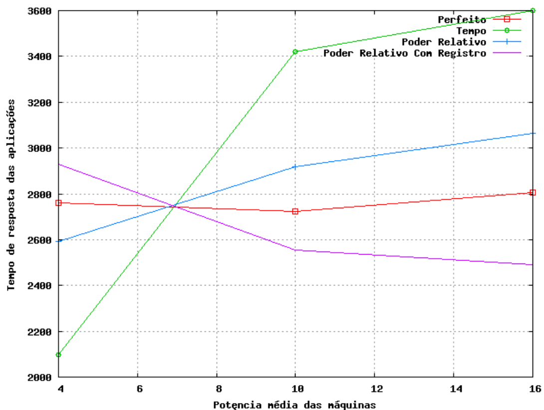
Figura 17. Evolução da média do tempo de resposta das aplicações de acordo com o poder das máquinas do peer no cenário 7.
