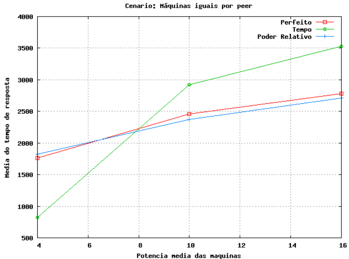
Figura 12. Evolução da média do tempo de resposta das aplicações de acordo com o poder das máquinas do peer no cenário 5.
