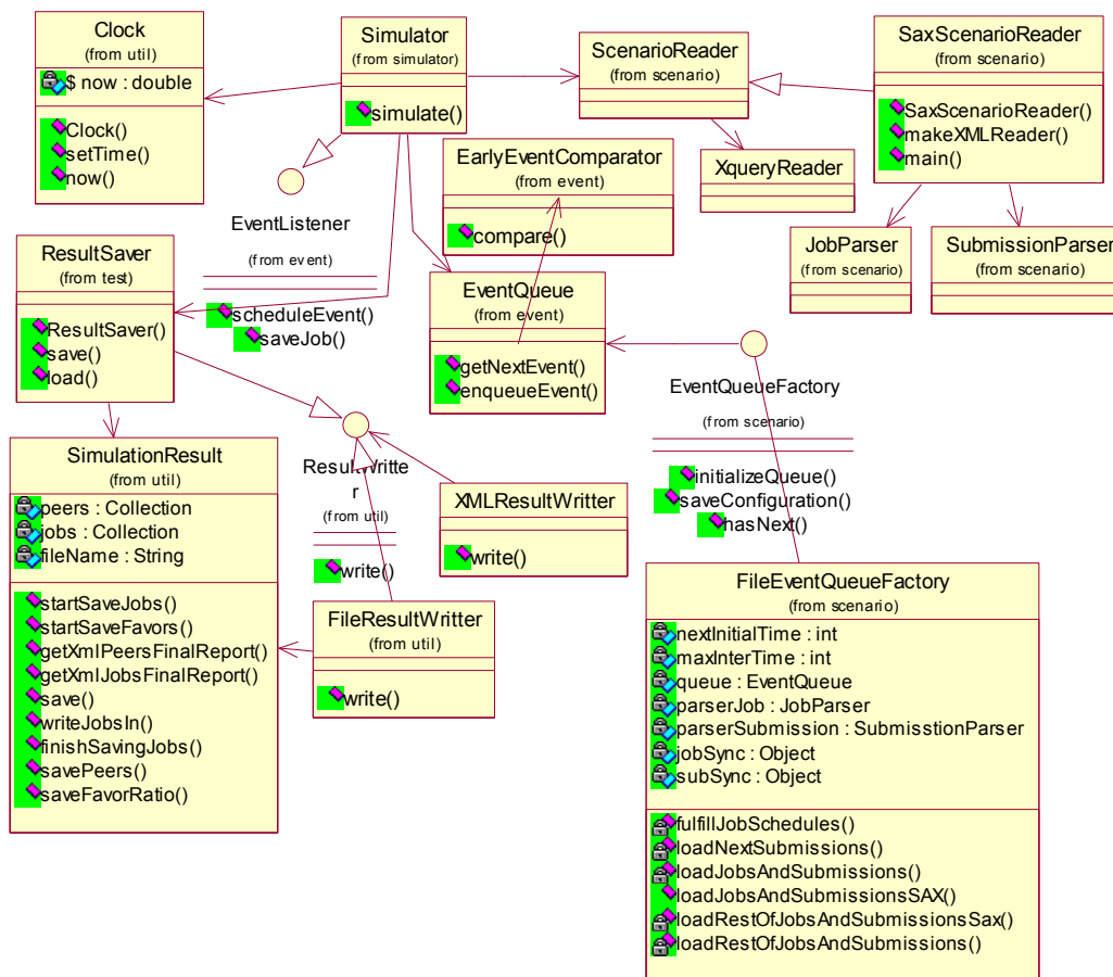
Figura 5. Diagrama da leitura de cenários, processamento e escrita de resultados.
