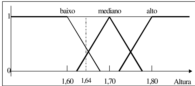
Figura 4.1 - Representação de valores na lógica fuzzy.
