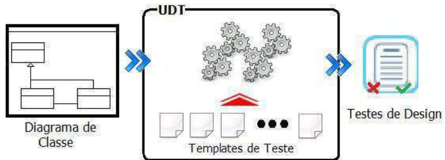
Figura 3.1: Processo geral para o uso de templates para a verificação de diagramas de classe
