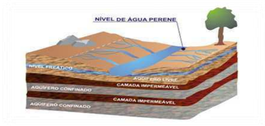
FIGURA 2: Tipos de Aquíferos quanto à pressão Fonte: BORGHETTI et al., (2004), adaptado de IGM, 2001.
