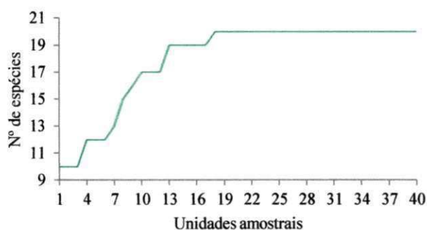
Figura 1. Suficiência amostral para a vegetação de caatinga na Fazenda Laranjeiras, município de São José de Espinharas – PB
