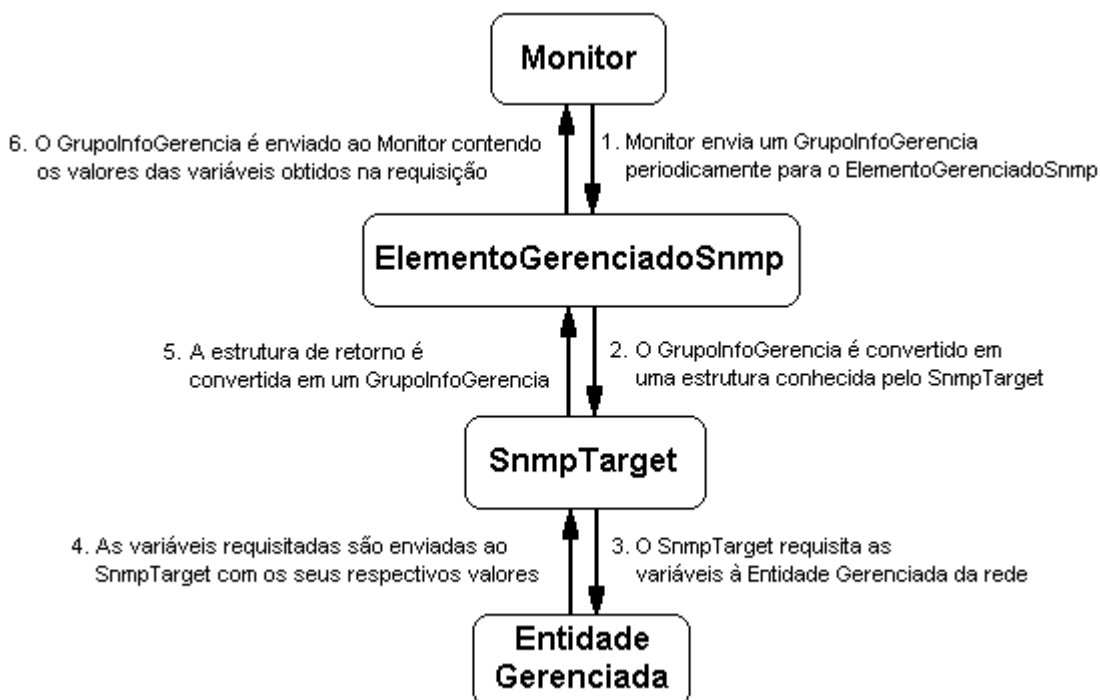
Figura 3.3. Representação de uma Requisição SNMP no fwGF
