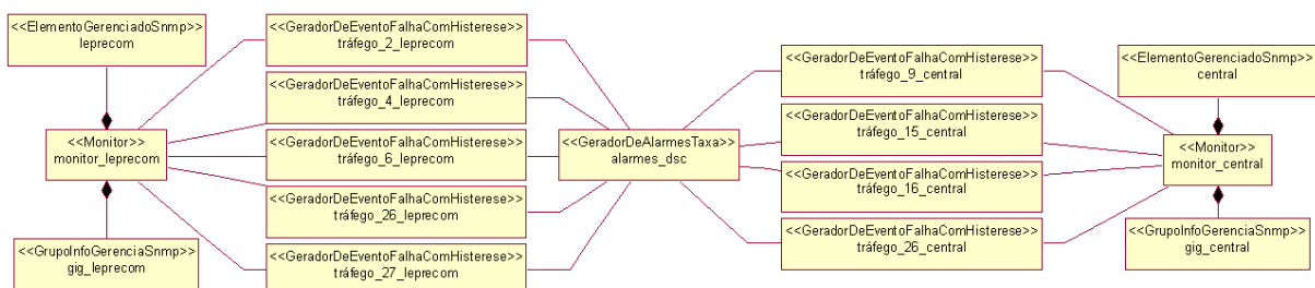
Figura 4.26. Componentes Monitor , GeradorDeEventoFalhaComHisterese e GeradorDeAlarmesTaxa para a aplicação Monitoramento de Tráfego em Interfaces de Comunicação.
