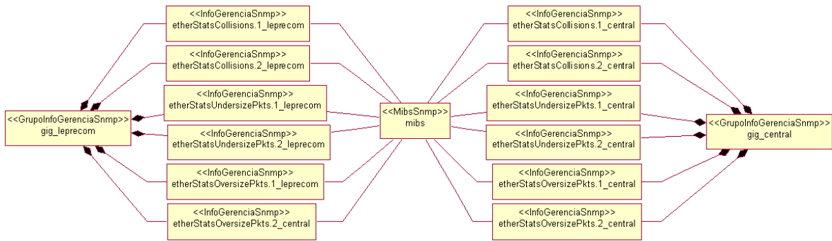
Figura 4.22. Componentes GrupoInfoGerenciaSnmpp, InfoGerenciaSnmpp e MibsSnmpp para a aplicação Monitoramento de Erros de Tamanho de Quadros e de Colisões.
