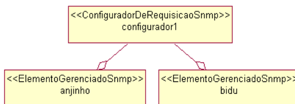
Figura 4.27. Componentes ConfiguradorDeRequisiçãoSnmpp e ElementoGerenciadoSnmpp para a aplicação Monitoramento de Espaço em Disco de Servidores.
