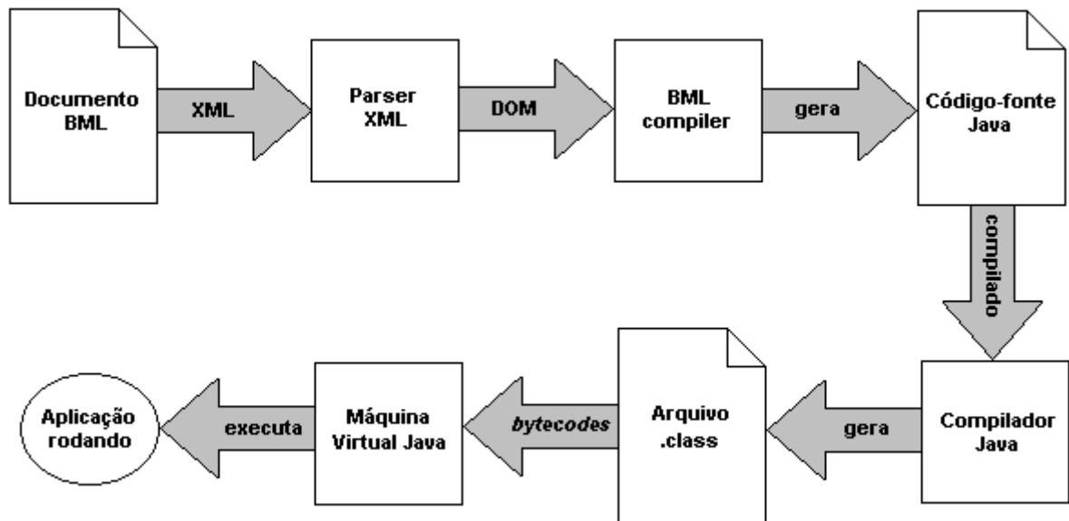
Figura 3.22. Executando uma aplicação com o BML compiler
