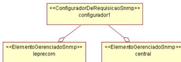
Figura 4.21. Componentes ConfiguradorDeRequisiçãoSnmp e ElementoGerenciadoSnmp para a aplicação Monitoramento de Erros de Tamanho de Quadros e de Colisões.
