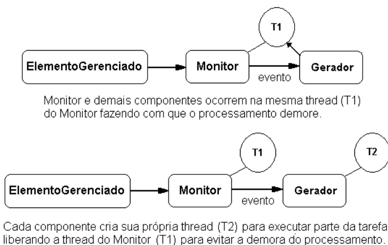
Figura 4.36. Processamento efetuado em uma ou mais threads
