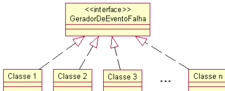
Figura 3.1. Herança de interface com o GeradorDeEventoFalha
