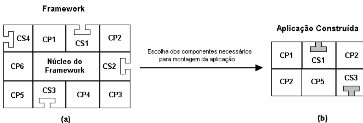
Figura 2.1. Representação dos componentes do framework
