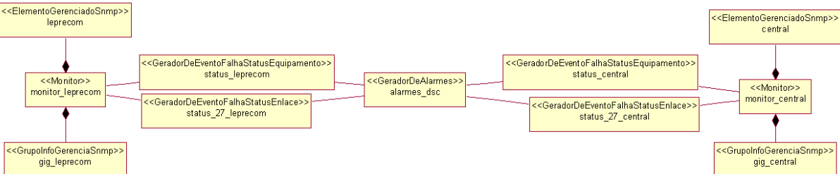
Figura 4.13. Componentes Monitor, GeradorDeEventoFalhaStatusEquipamento, GeradorDeEventoFalhaStatusEnlace e GeradorDeAlarmesStatus para a aplicação Conectividade.
