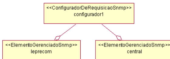
Figura 4.18. Componentes ConfiguradorDeRequisiçãoSnmpp e ElementoGerenciadoSnmpp para a aplicação Monitoramento de Erros em Interfaces de Comunicação.
