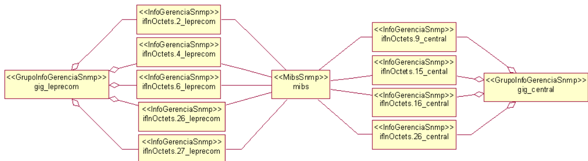
Figura 4.25. Componentes GrupoInfoSnmp , InfoGerenciaSnmp e MibsSnmp para a aplicação Monitoramento de Tráfego em Interfaces de Comunicação.
