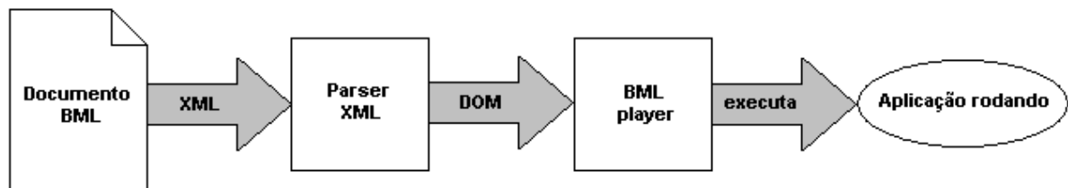
Figura 3.21. Executando uma aplicação com o BML player
