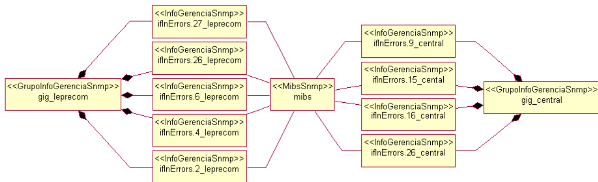
Figura 4.19. Componentes GrupoInfoGerenciaSnmP, InfoGerenciaSnmP e MibsSnmP para a aplicação Monitoramento de Erros em Interfaces de Comunicação.
