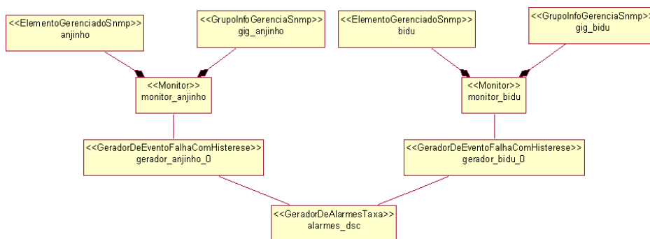
Figura 4.32. Componentes Monitor, GeradorDeEventoFalhaComHisterese e GeradorDeAlarmesTaxa para a aplicação Monitoramento de Saturação de Conexões.
