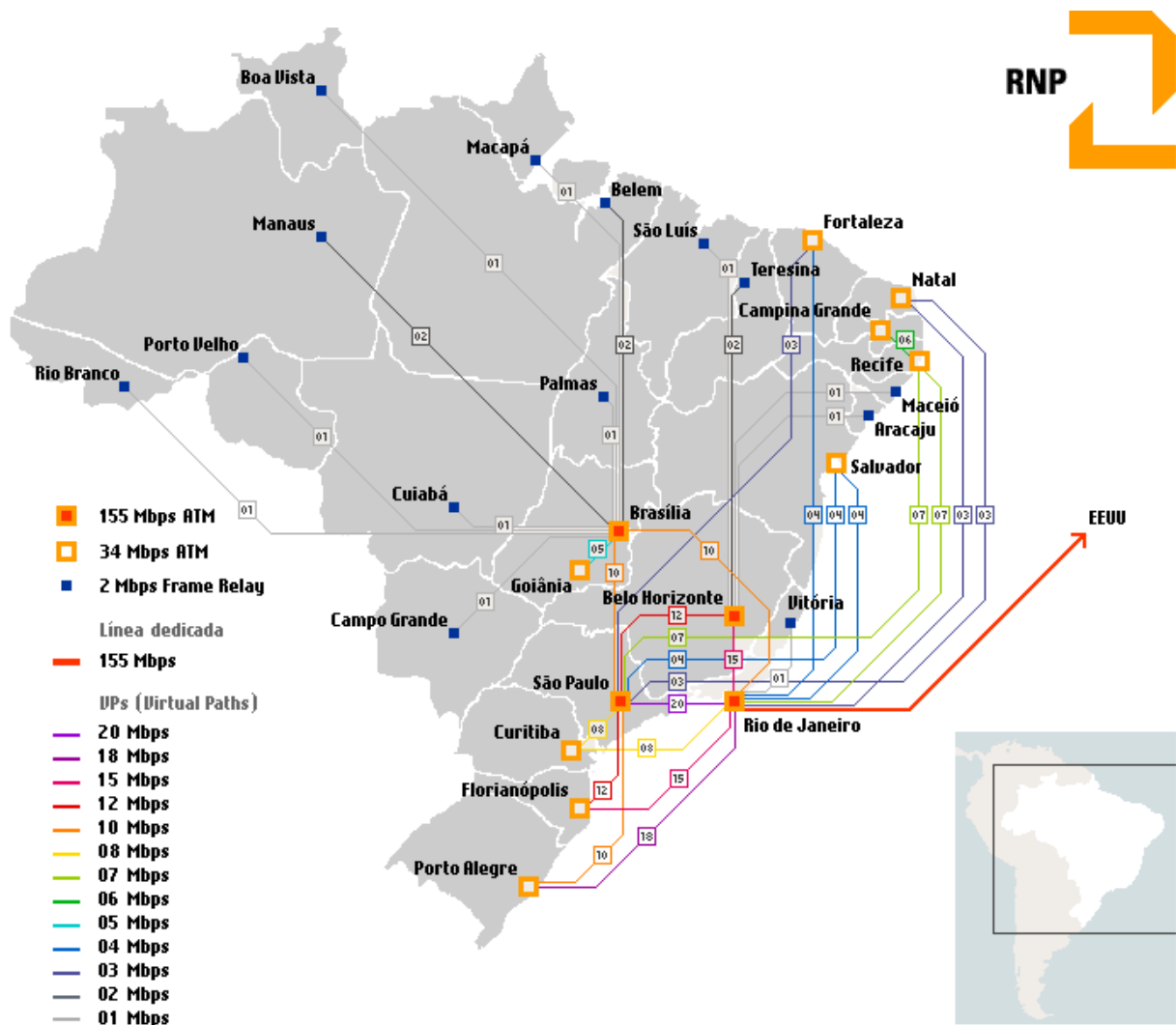
Figura 5.10. Estrutura do Backbone da Rede Nacional de Pesquisa (RNP)
