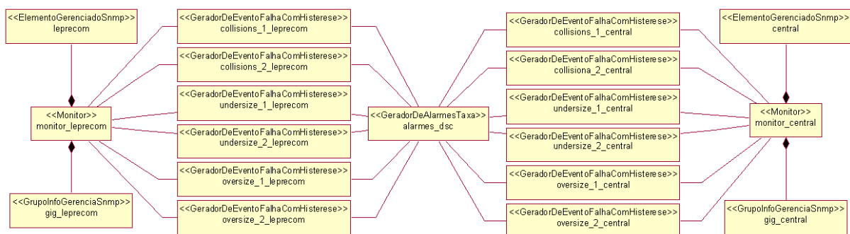
Figura 4.23. Componentes Monitor, GeradorDeEventoFalhaComHisterese e GeradorDeAlarmesTaxa para a aplicação Monitoramento de Erros de Tamanho de Quadros e de Colisões.
