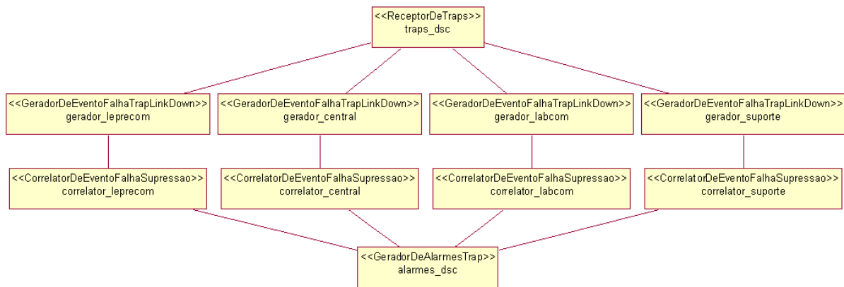
Figura 4.34. Componentes ReceptorDeTrapsSnmp, CorrelatorDeEventoFalhaSupressao, GeradorDeEventoFalhaTrapLinkDown e GeradorDeAlarmesTrap para a aplicação Monitoramento Assíncrono da Rede.
