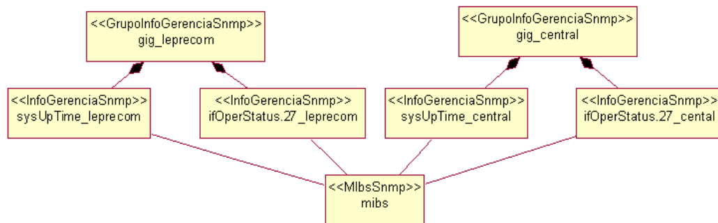
Figura 4.9. Componentes GrupoInfoGerenciaSnm, InfoGerenciaSnm e MibsSnm para a aplicação Conectividade.
