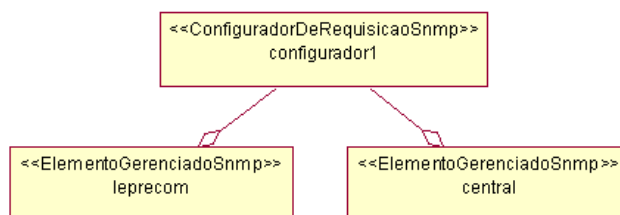
Figura 4.24. Componentes ConfiguradorDeRequisiçãoSnmpp e ElementoGerenciadoSnmpp para a aplicação Monitoramento de Tráfego em Interfaces de Comunicação.
