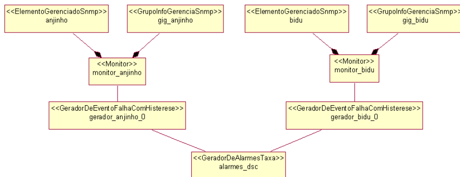
Figura 4.29. Componentes Monitor, GeradorDeEventoFalhaComHisterese e GeradorDeAlarmesTaxa para a aplicação Monitoramento de Espaço em Disco de Servidores.
