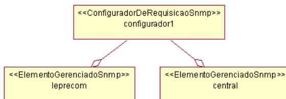
Figura 4.6. Componentes ConfiguratorDeRequisiçãoSnmp e ElementoGerenciadoSnmp para a aplicação Conectividade.
