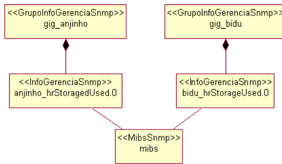
Figura 4.28. Componentes GrupoInfoSnmpp, InfoGerenciaSnmpp e MibsSnmpp para a aplicação Monitoramento de Espaço em Disco de Servidores.
