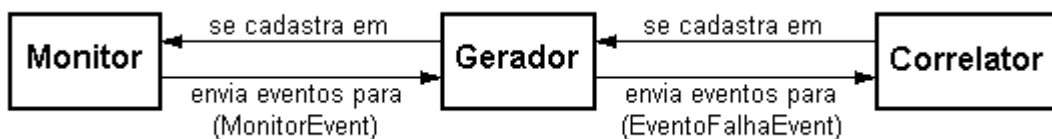
Figura 2.5. Padrão Observer no framework .
