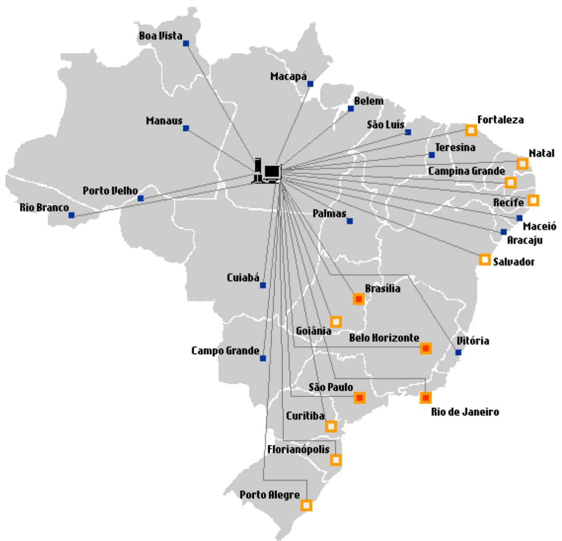
Figura 5.11. Backbone da RNP monitorado por uma aplicação de gerência centralizada
