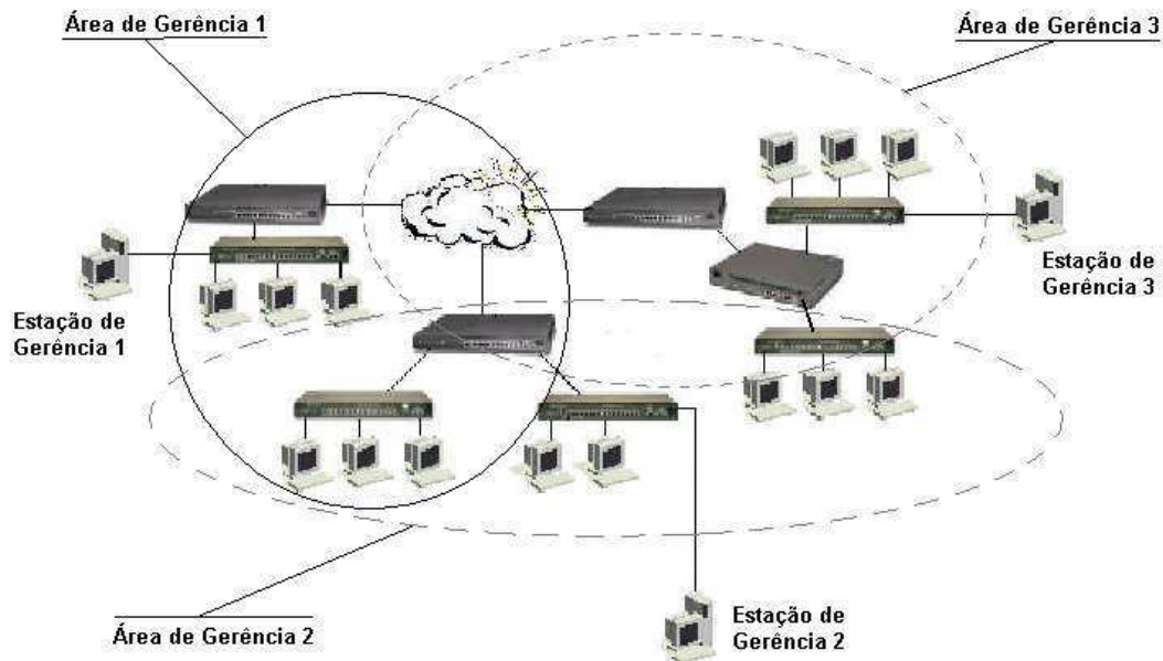
Figura 5.5. Sobreposição de áreas de gerenciamento
