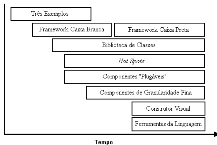
Figura 5.1. Evolução de Frameworks
