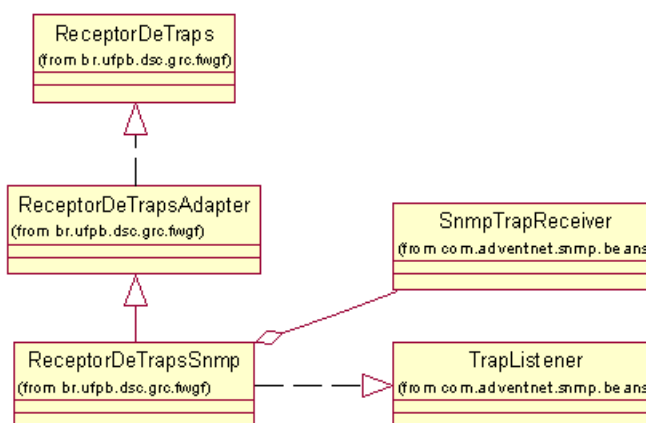
Figura 3.7. Uso do padrão de projeto Adapter no ReceptorDeTrapsSnmp
