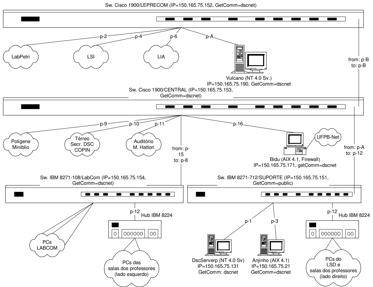
Figura 4.3. Topologia da Rede do DSC.
