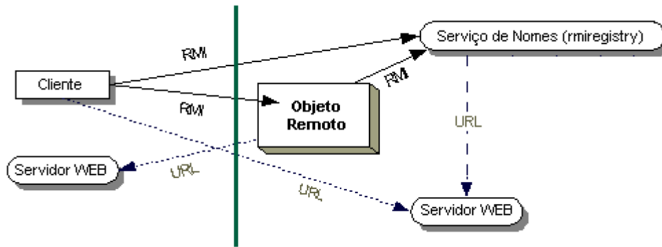
Figura 5.6. Arquitetura de uma aplicação RMI
