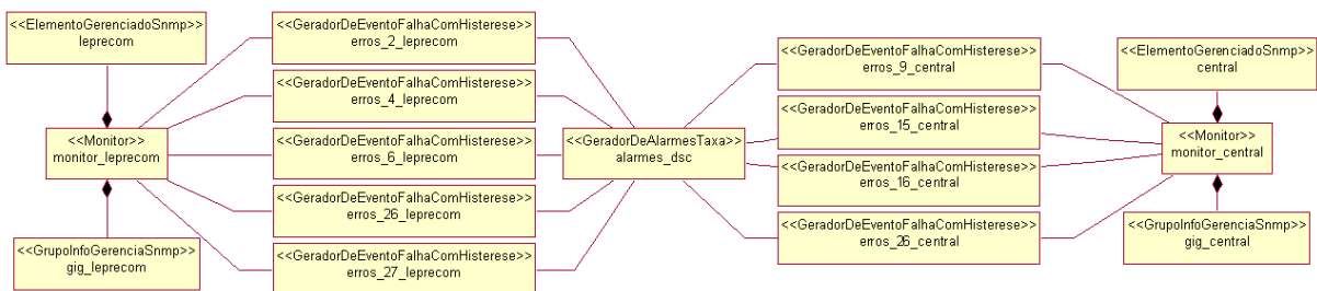
Figura 4.20. Componentes Monitor, GeradorDeEventoFalhaComHisterese e GeradorDeAlarmesStatus para a aplicação Monitoramento de Erros em Interfaces de Comunicação.
