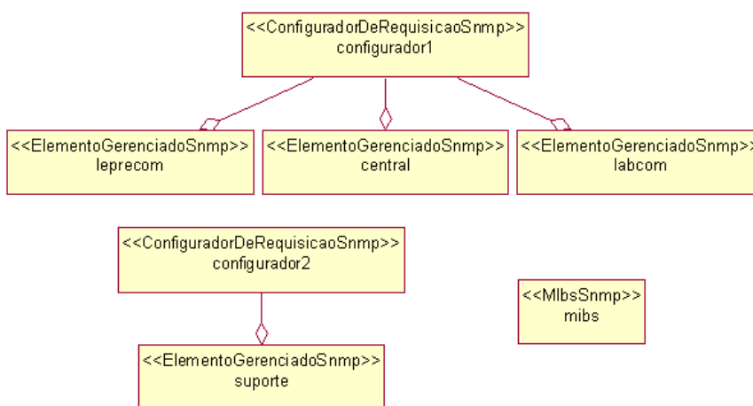
Figura 4.33. Componentes ConfiguradorDeRequisiçãoSnmpp, ElementoGerenciadoSnmpp e MibsSnmpp para a aplicação Monitoramento Assíncrono da Rede.
