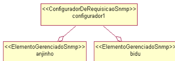
Figura 4.30. Componentes ConfiguradorDeRequisicaoSnmp e ElementoGerenciadoSnmp para a aplicação Monitoramento de Saturação de Conexões.
