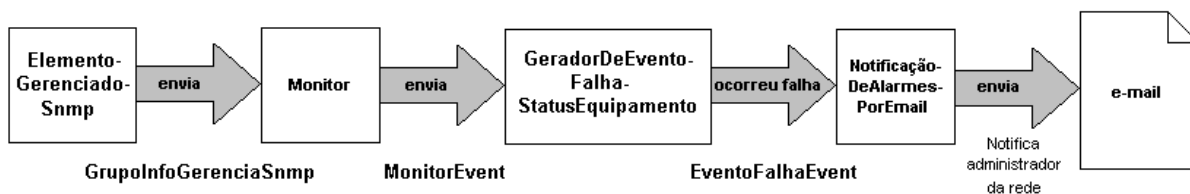
Figura 2.6. Aplicação de monitoração de um roteador construída com o fwGF: Comunicação entre os componentes
