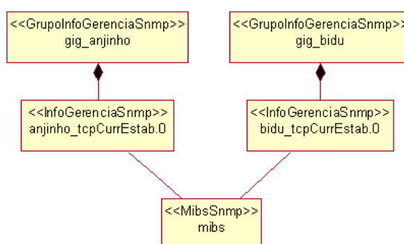
Figura 4.31. Componentes GrupoInfoSnm , InfoGerenciaSnm e MibsSnm para a aplicação Monitoramento de Saturação de Conexões.
