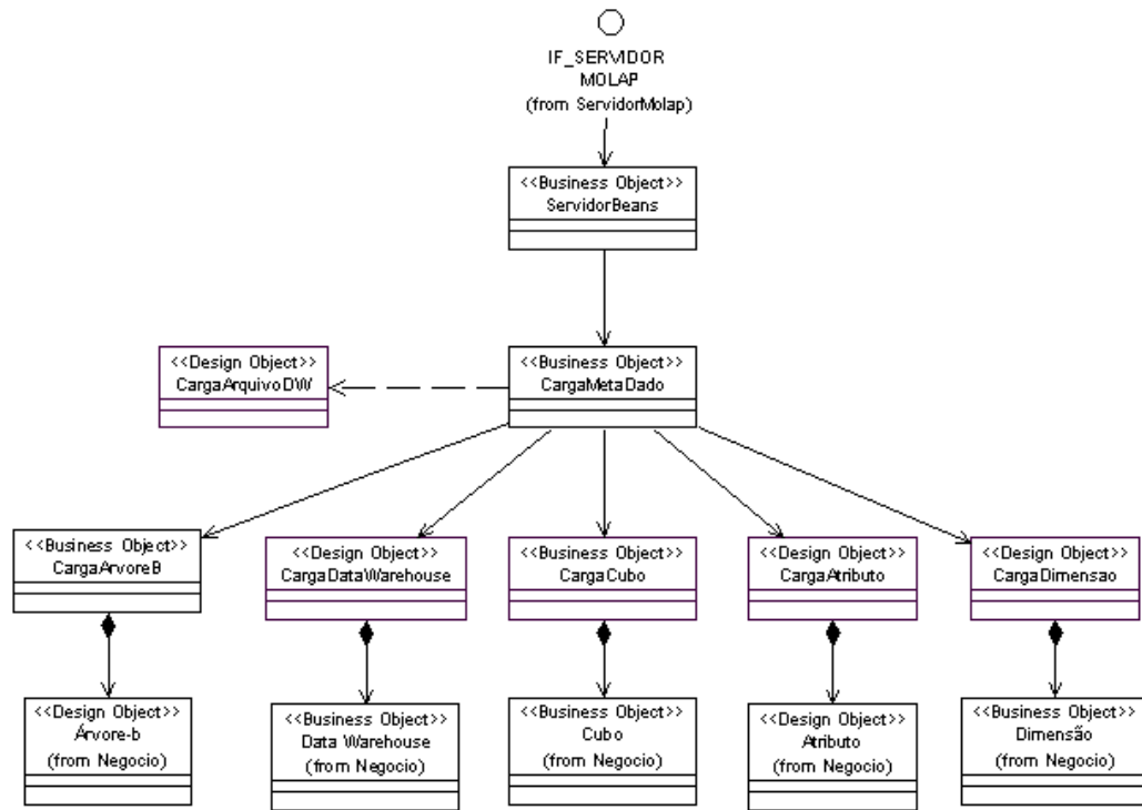
Figura 18: Pacote CargaMetadado
