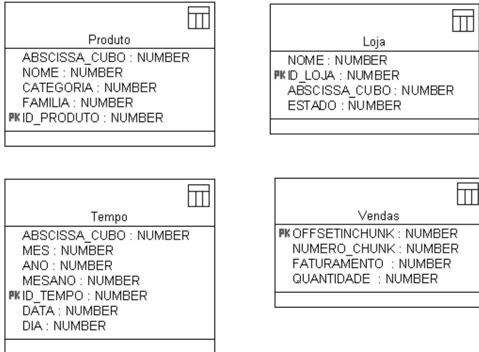
Figura 22: Tabelas do Pacote EsquemaSGBD
