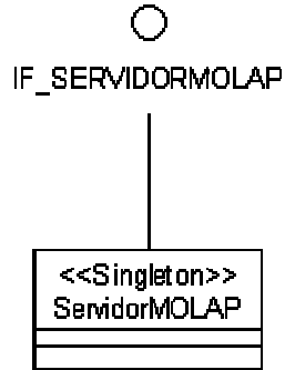
Figura 21: Subsistema ServidorMolap
