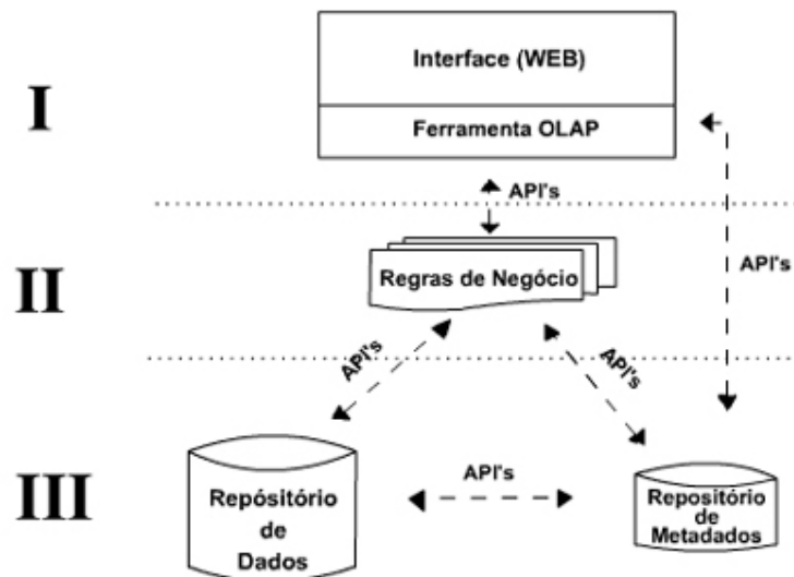
Figura 13: Arquitura em Camadas do Protótipo
