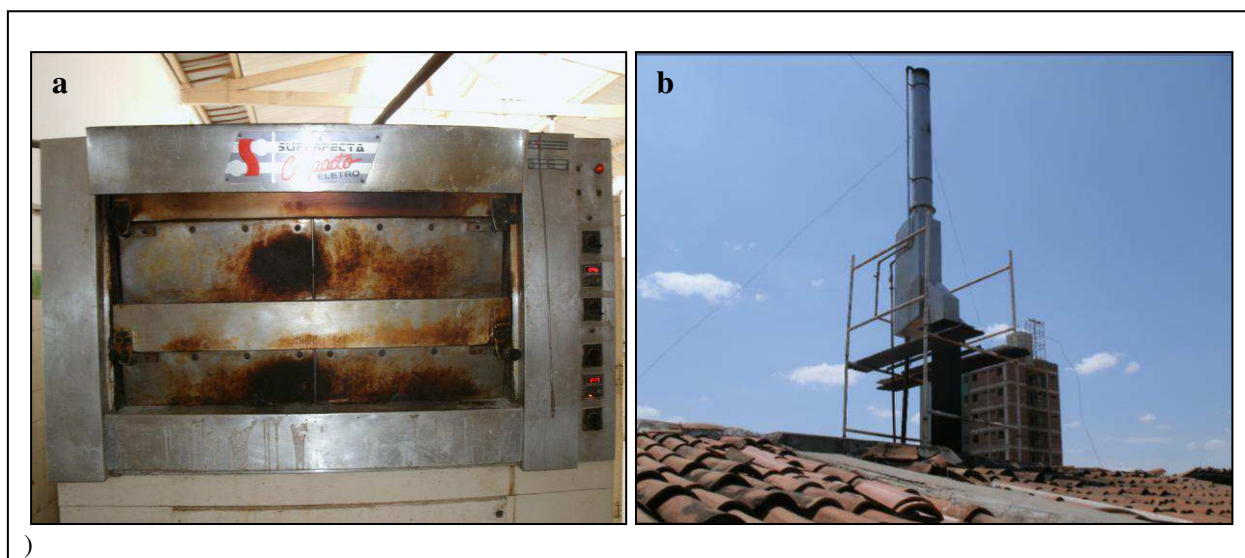
Figura 5 – Equipamentos da padaria que utiliza tecnologia limpa na cidade de Patos – PB. Detalhes do forno (a) e do ecofiltro (b)
