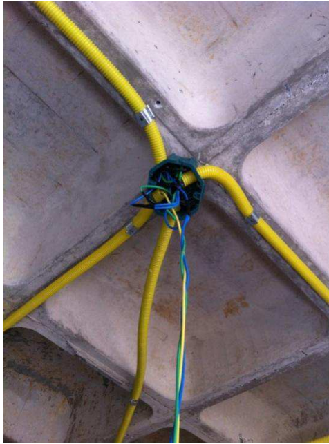
Figura 3. Ponto de iluminação 1h envia três eletrodutos.
