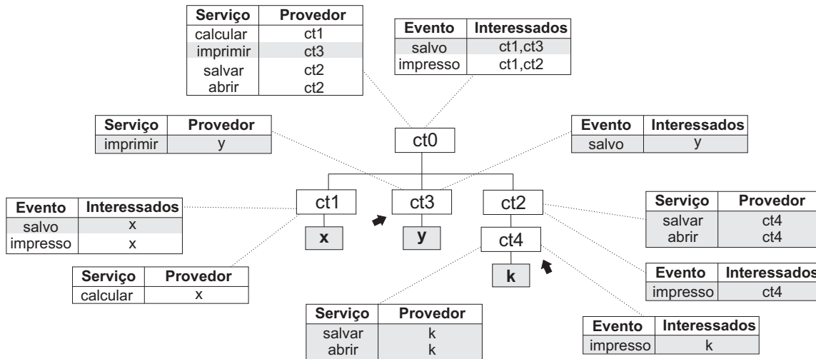
Figura 4.25: Cenário de evolução de nível 2 de complexidade.
