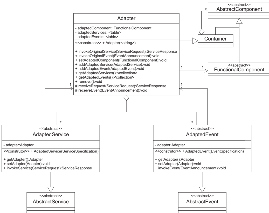
Figura A.17: Diagrama de classes relacionadas ao modelo de adaptadores.
