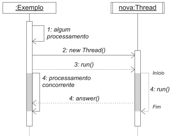
Figura B.3: Diagrama de seqüência de eventos com criação de nova thread .
