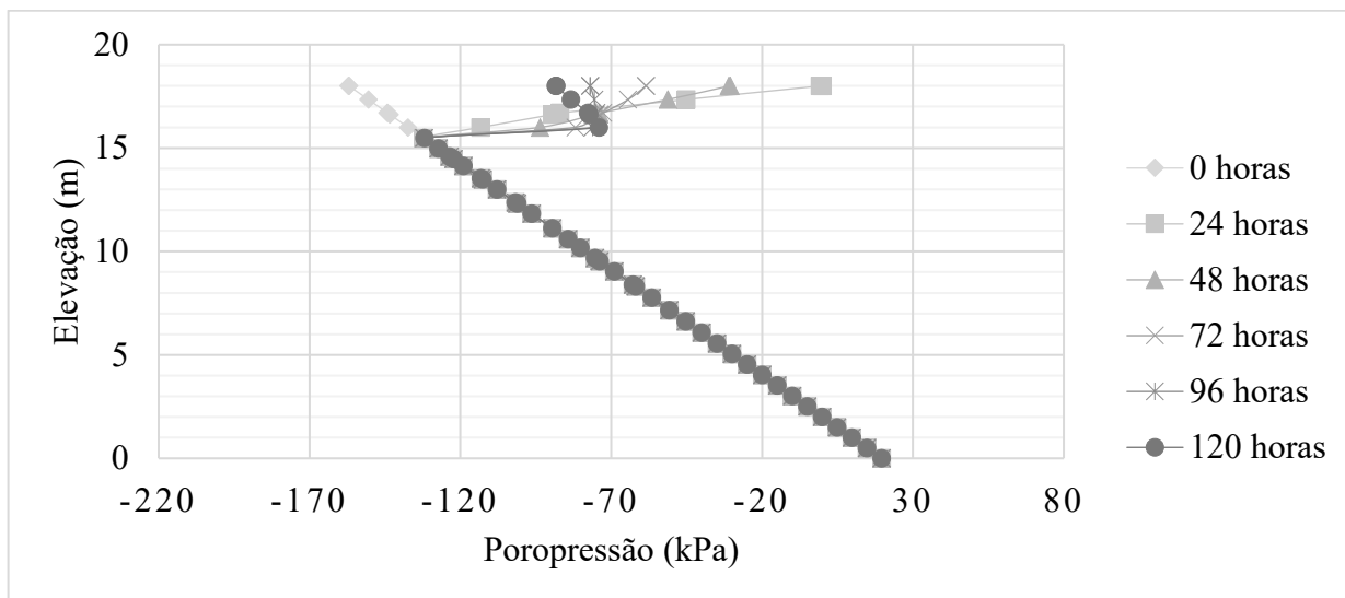
Figura 54-Distribuição de poropressão para os eventos de chuva de 24h de duração do talude João Lourenço
