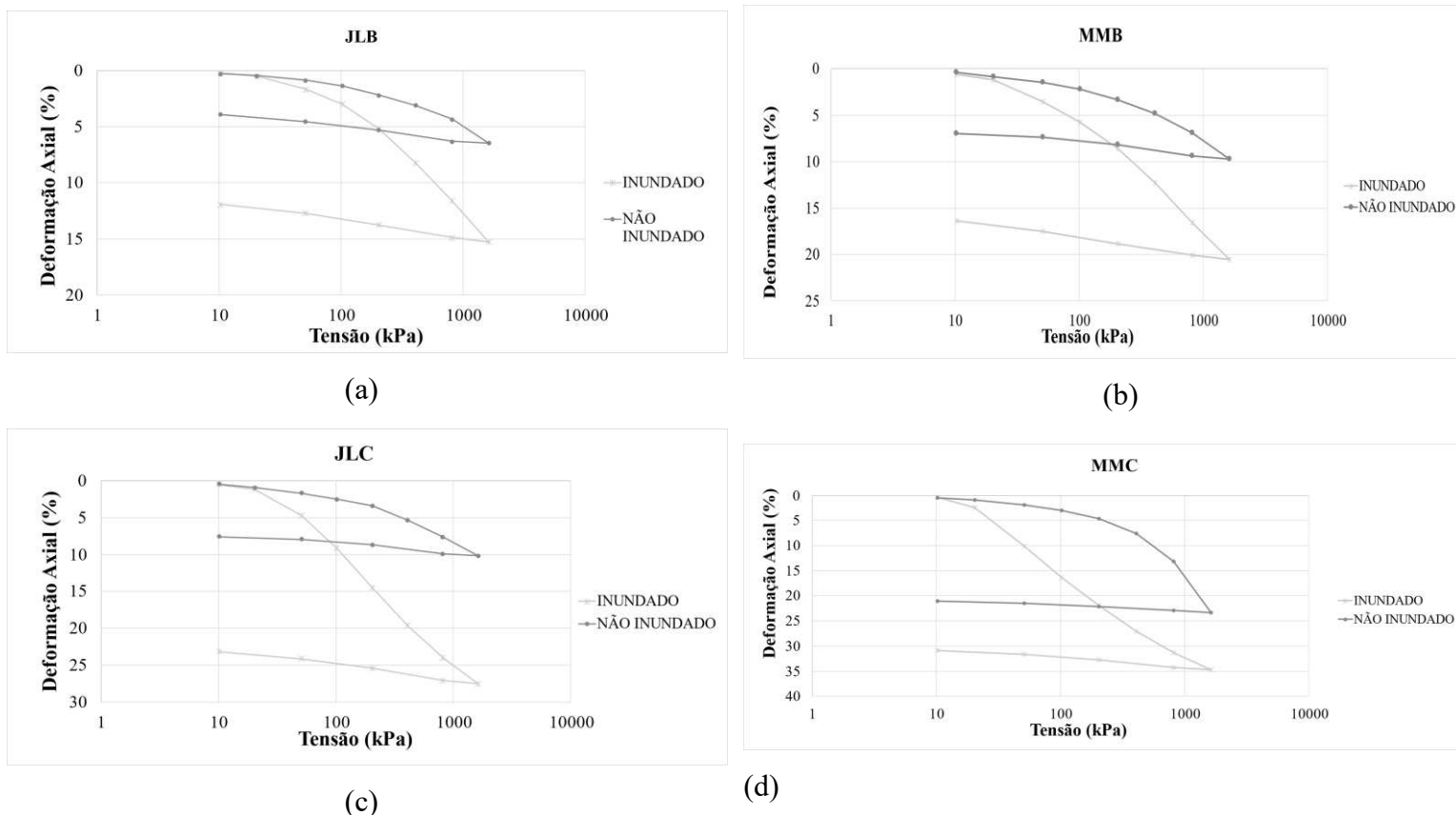
Figura 40-Curvas de deformação axial versus tensão dos solos
