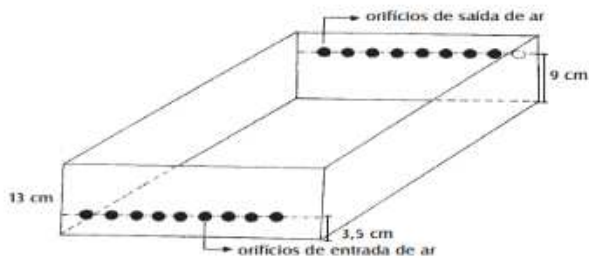
Figura 1. Disposição dos furos na caixa. Fonte: ESALQ (2004).
