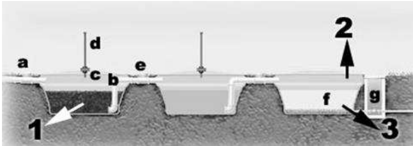
Figura 1. Esquema da construção da Fossa Séptica.
