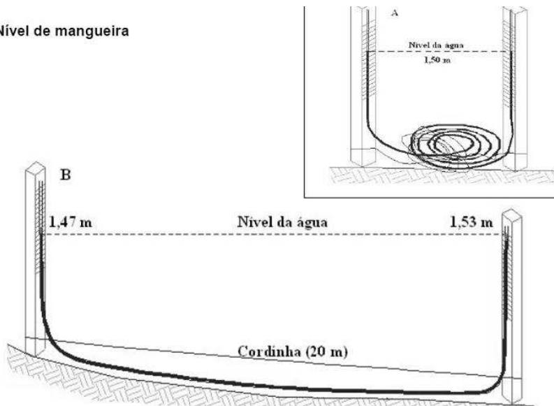
Figura 1. Tomada do nível. Fonte: PATAC (1987).
