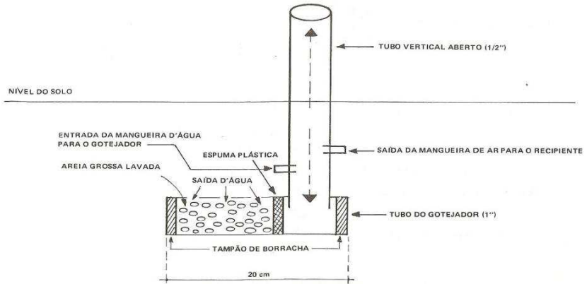
Figura 1. Corte longitudinal do gotejador. Fonte: EMATER (1981).
