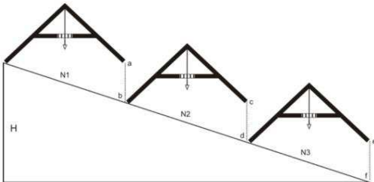
Figura 2. Marcação do terreno. Fonte: PATAC (1987).
