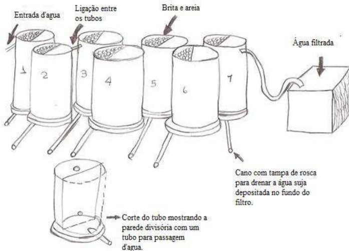
Figura 1. Processo de Montagem. Fonte: EMBRATER (1984).
