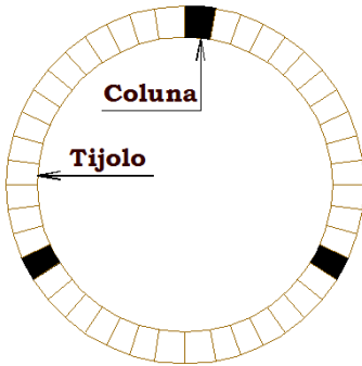
Planta baixa do poço onde se observa a disposição das colunas e dos tijolos
