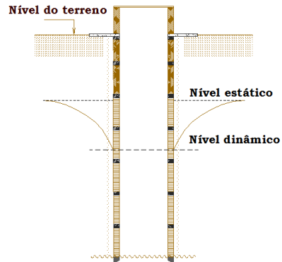
Corte esquemático, identificando a posição dos elementos estruturais e a sua disposição ao longo do poço.
