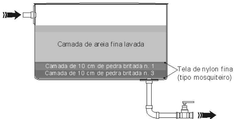
Figura 2. Esquema de montagem da caixa. Fonte: EMBRAPA (2013).
