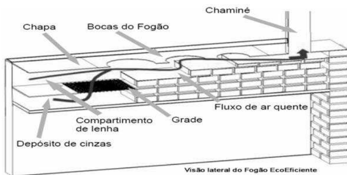
Figura 1. Estrutura e materiais.
