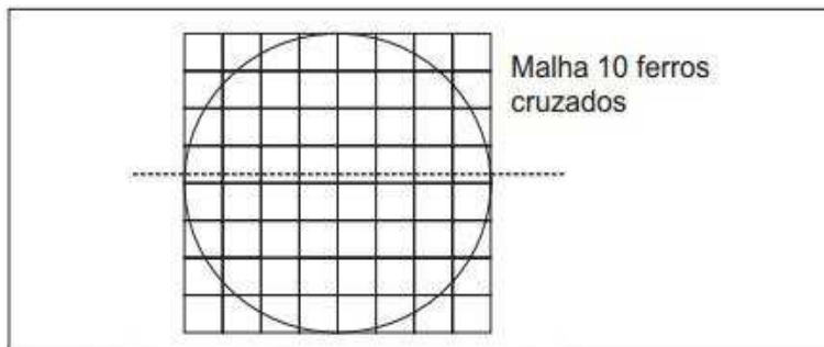
Figura 3. Estrutura da malha de ferro do fundo da cisterna.
