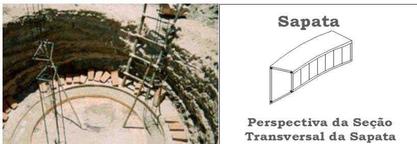
Figura 3. Sapata moldada, com a ferragem das colunas; detalhe da sapata cortante.
