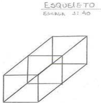
Figura 2. Estrutura de cano Esquema.
