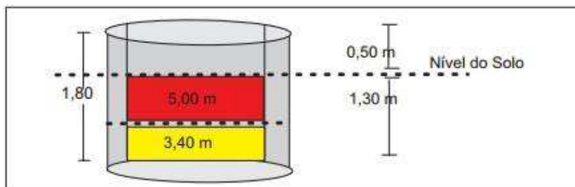
Figura 2. Dimensões da escavação. Fonte: Programa Sertão Vivo (2005).
