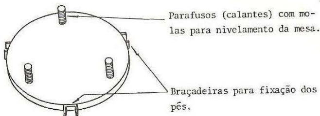
Figura 1. Roda inferior da mesa. Fonte: EMATER (1985).
