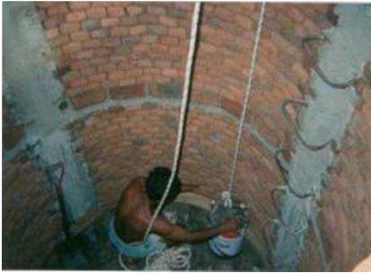
Figura 5. Interior do poço: sapata, alvenaria seca, cinta, coluna e escada.
