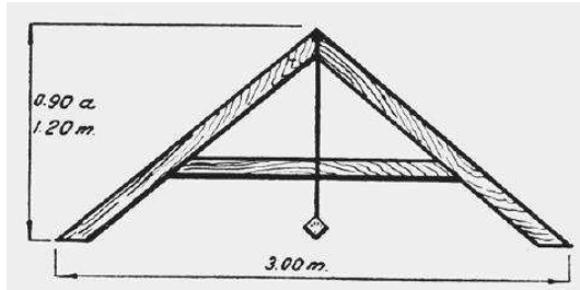
Figura 1. Nível A. Fonte: PATAC (1987).
