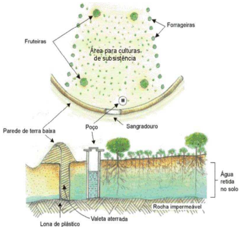
Figura 1. Esquemática de montagem da barragem subterrânea.
