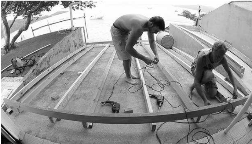
Figura 2. Construção da estrutura de madeira da plataforma.
