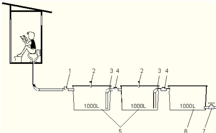
Figura 1. Esquema de montagem. Fonte: EMBRAPA (2013).
