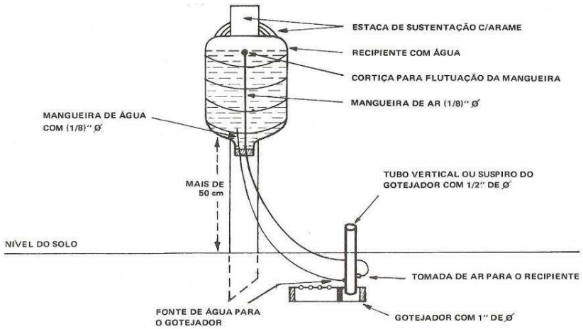
Figura 1. Corte longitudinal do gotejador. Fonte: EMATER (1981).
