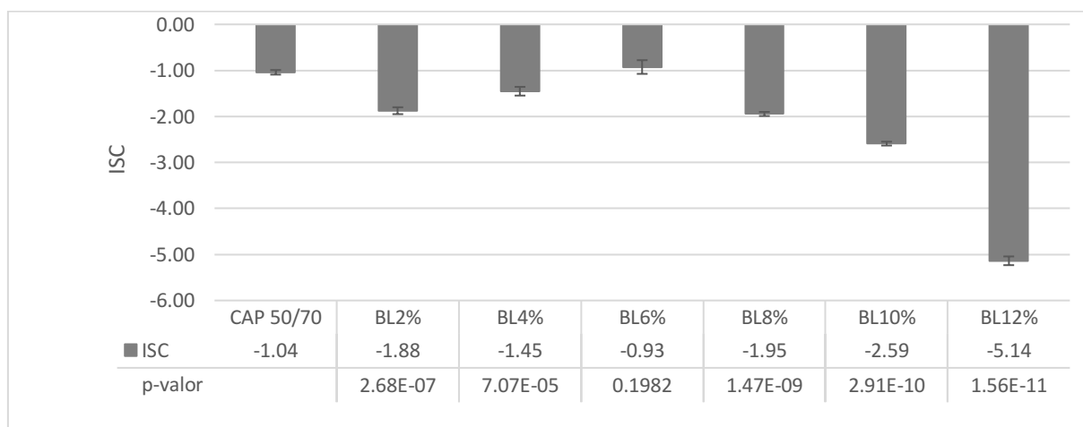
Figura 36 - Resultados do Índice de Susceptibilidade Térmica
