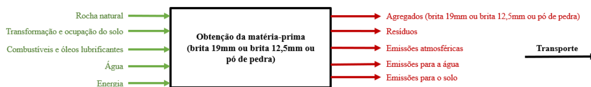
Figura 72- DFV do processo elementar de obtenção da matéria prima (brita 19mm ou brita 12,5mm ou pó de pedra)
