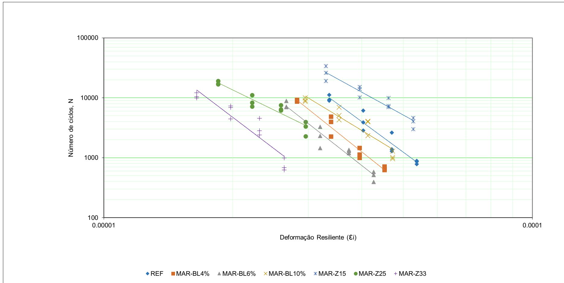
Figura 66 - Número de ciclos versus deformação resiliente inicial
