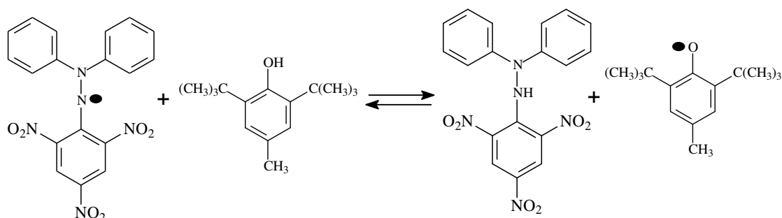
Figura 3 Reação química entre o BHT e o radical DPPH•. Fonte: SANTOS, F.O. (2011).
