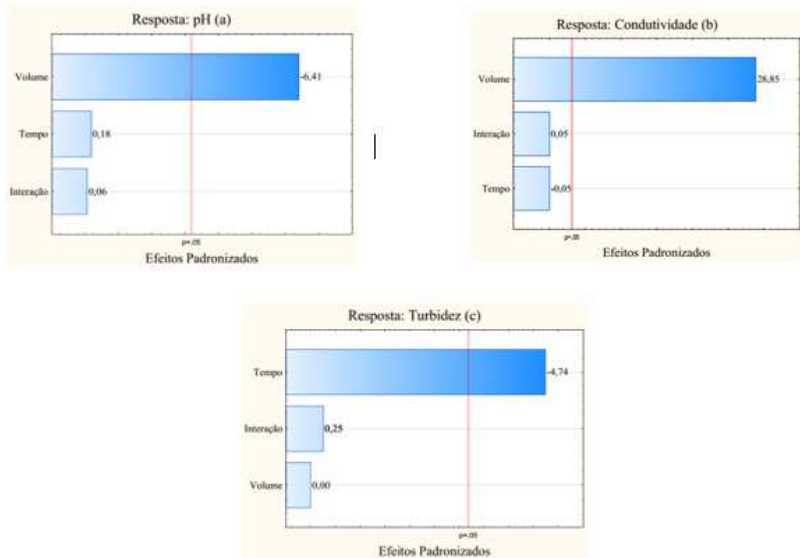
Figura 5 – Diagramas de Pareto para os efeitos padronizados em p = 0,05 , para as repostas pH (a), condutividade (b) e turbidez (c), aplicando o sulfato em solução.
