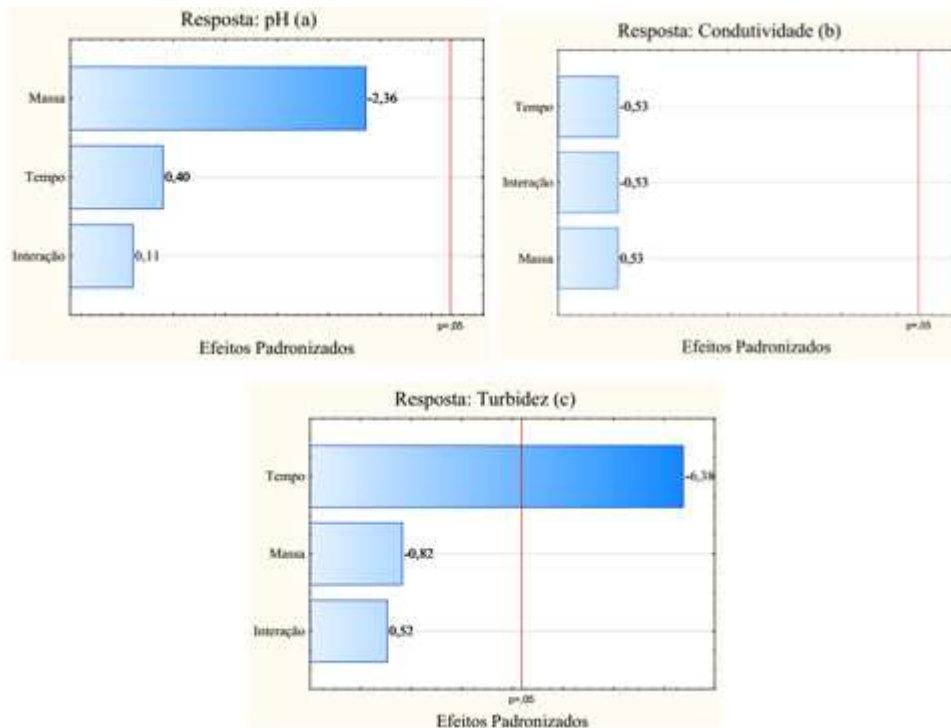
Figura 6 – Diagramas de Pareto para os efeitos padronizados em p = 0,05 , para as repostas pH (a), condutividade elétrica (b) e turbidez (c), aplicando o sulfato em pó como coagulante.
