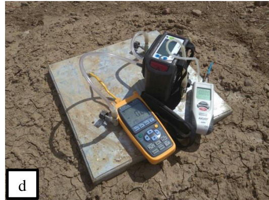
(d) instalação dos equipamentos de medição e início do ensaio
