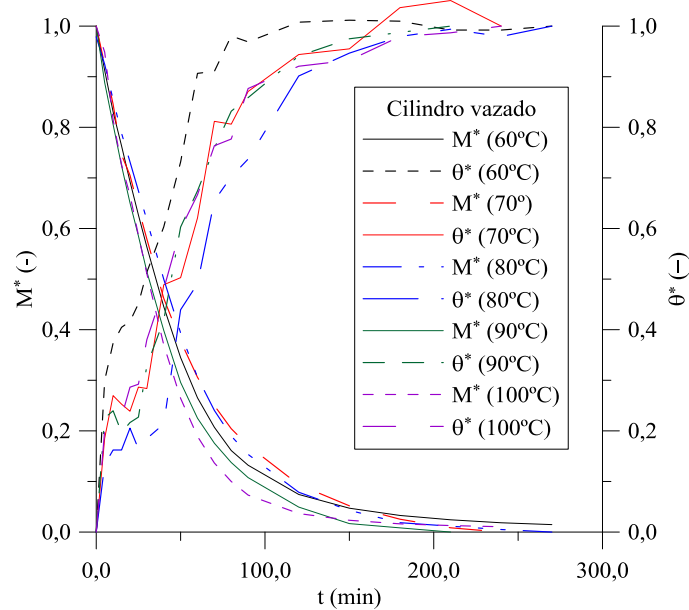
Figura 4.8 – Variação do teor de umidade e do aquecimento em todas as temperaturas pesquisadas acoplados para o cilindro vazado.
