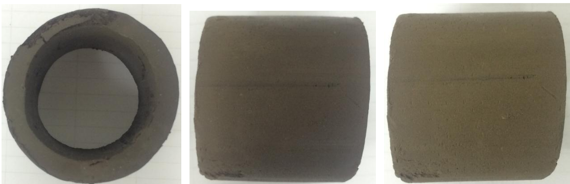
Figura 4.13 – Imagem do cilindro vazado no processo de secagem a 80°C.
