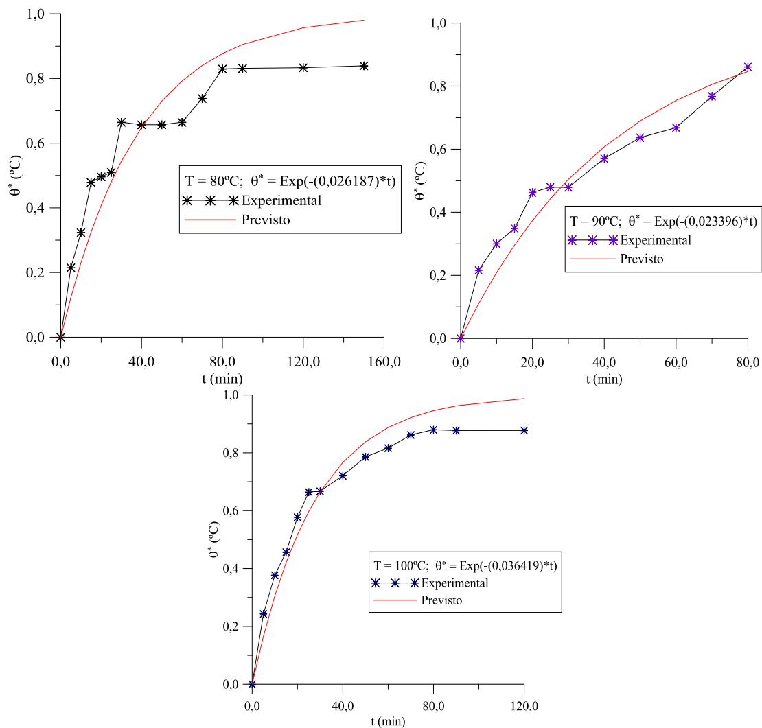
Figura 4.58 – Comparação entre as temperaturas da amostra experimental e prevista para o experimento realizado com o cilindro vazado com barra transversal nas temperaturas de 80°C, 90°C e 100°C.
