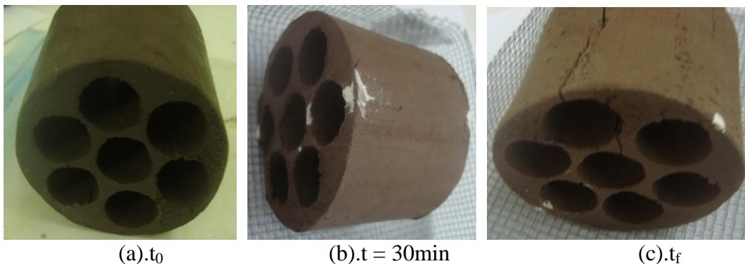
(a). t_0 (b). t = 30\text{min} (c). t_f Figura 4.27 – Imagem do cilindro vazado com sete furos (tambor) no processo de secagem a 100^\circ\text{C}
