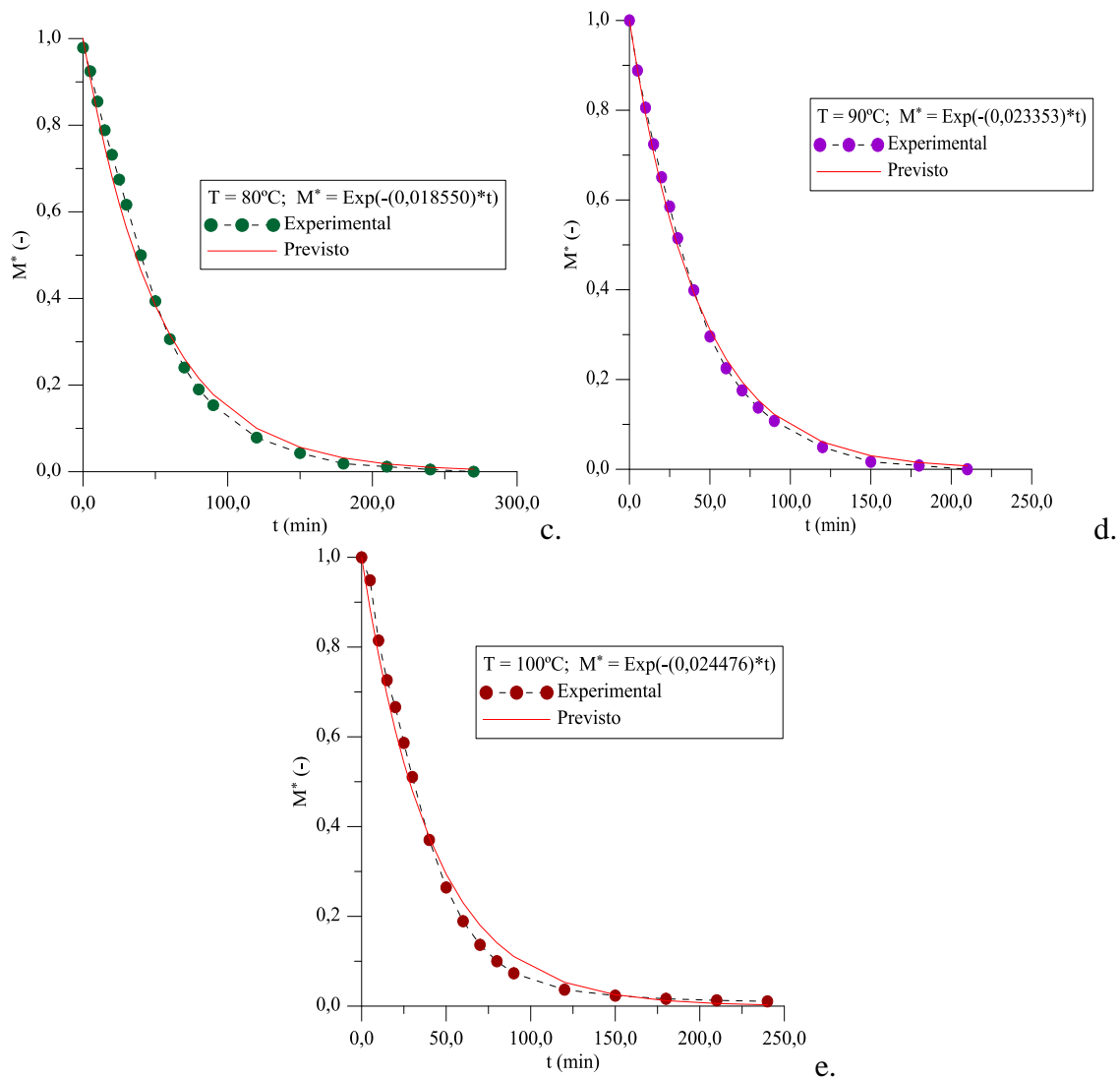
Figura 4.48 – Comparação entre os teores de umidade médios da amostra experimental e previsto para o experimento realizado com o cilindro vazado nas temperaturas de 80°C, 90°C e 100°C.
