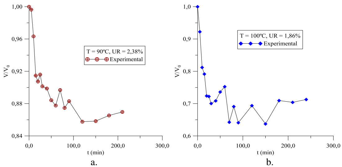
Figura 4.10 – Variação do volume do cilindro vazado durante a secagem para diferentes temperaturas (90°C e 100°C) em função do tempo de secagem.
