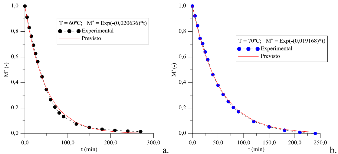
Figura 4.47 – Comparação entre os teores de umidade médios da amostra experimental e previsto para o experimento realizado com o cilindro vazado nas temperaturas de 60°C e 70°C.
