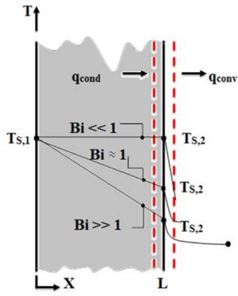
Figura 2.2 - Efeito do número de Biot na distribuição de temperatura em regime permanente numa parede plana com convecção na superfície (Incropera e De Witt, 2002).
