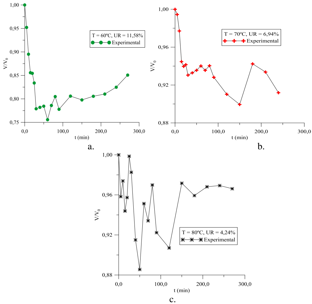
Figura 4.9 – Variação do volume do cilindro vazado durante a secagem para diferentes temperaturas (60°C, 70° e 80°C) em função do tempo de secagem.
