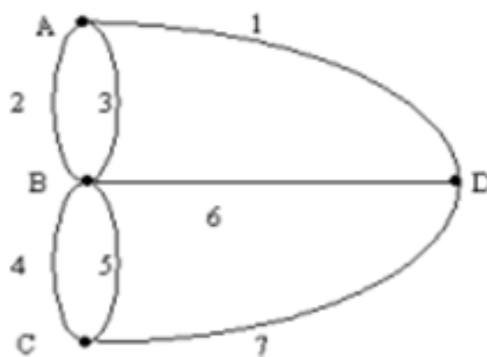
Figura 6 – Modelo Matemático para a solução do problema
