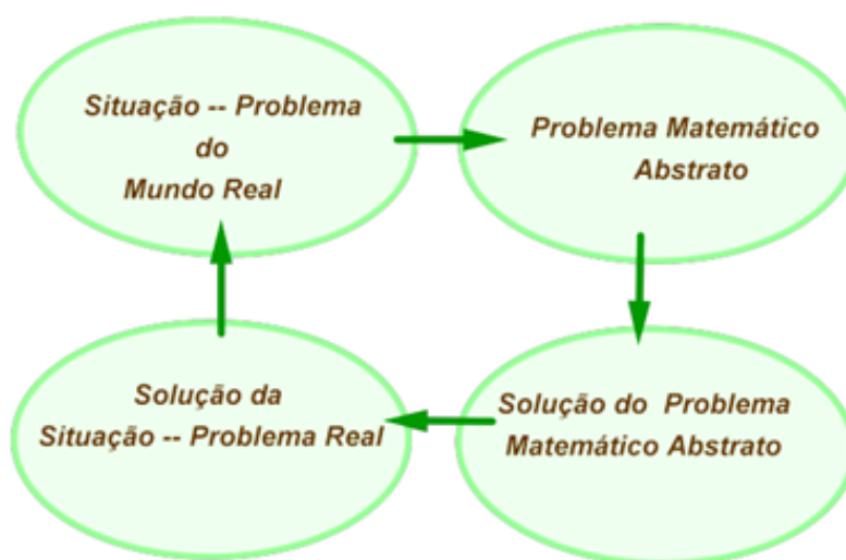
Figura 2 – Diagrama da Modelagem Matemática
