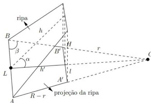
Figura 9 – Projeção ortogonal de uma ripa
